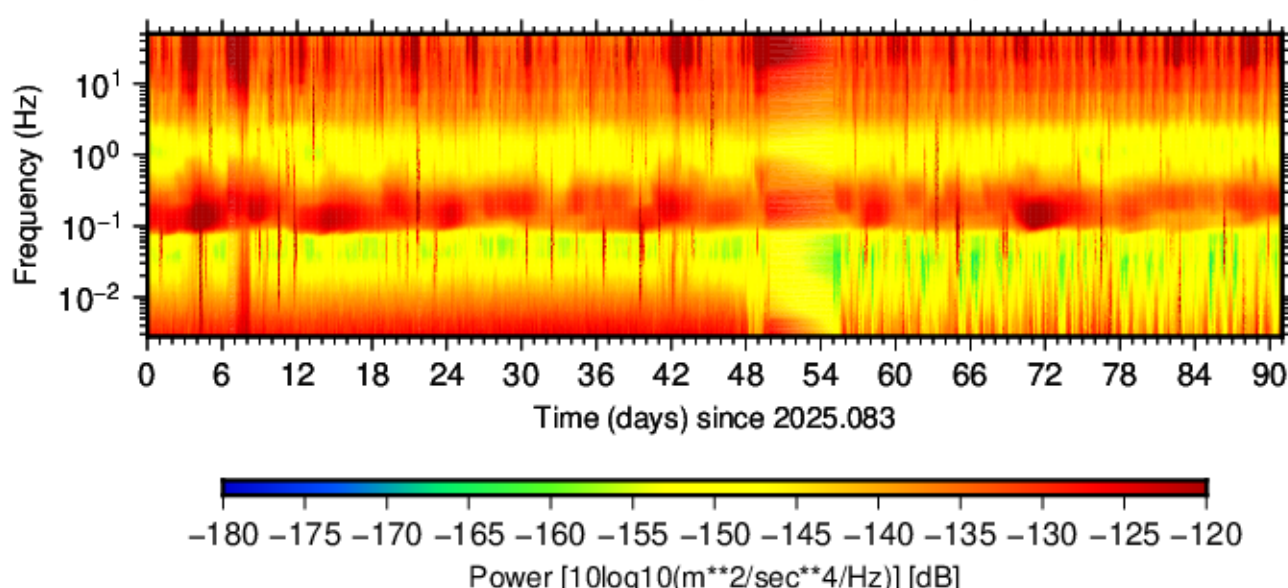
BK.YUBA.HHN.00 (2025.083 - 2025.173)
