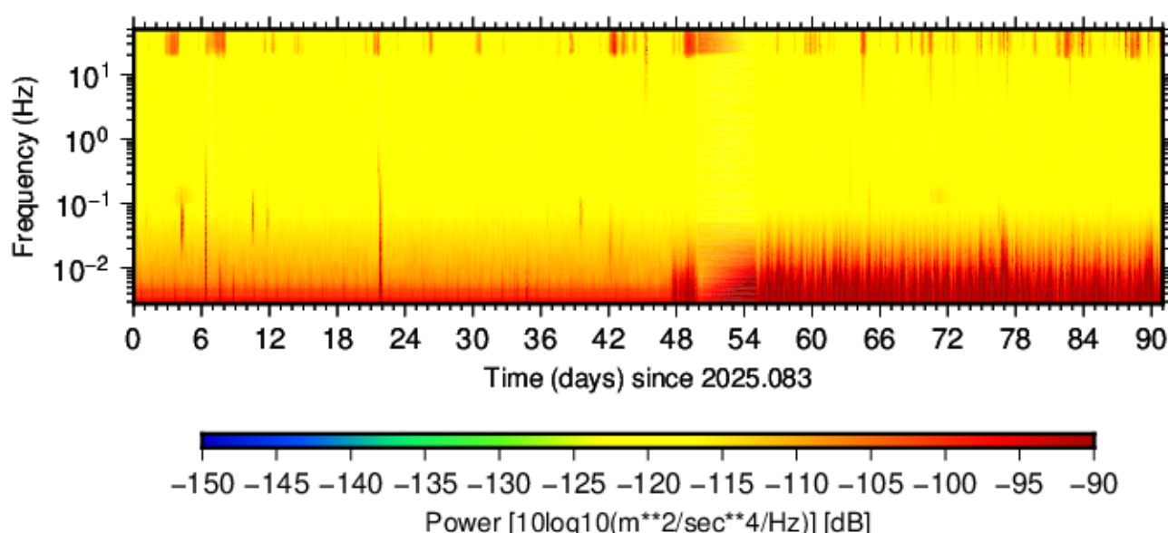
BK.YUBA.HNZ.00 (2025.083 - 2025.173)
