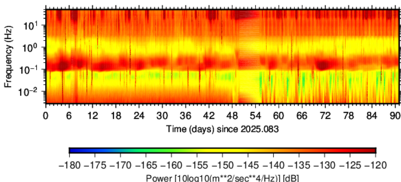
BK.YUBA.HHE.00 (2025.083 - 2025.173)
