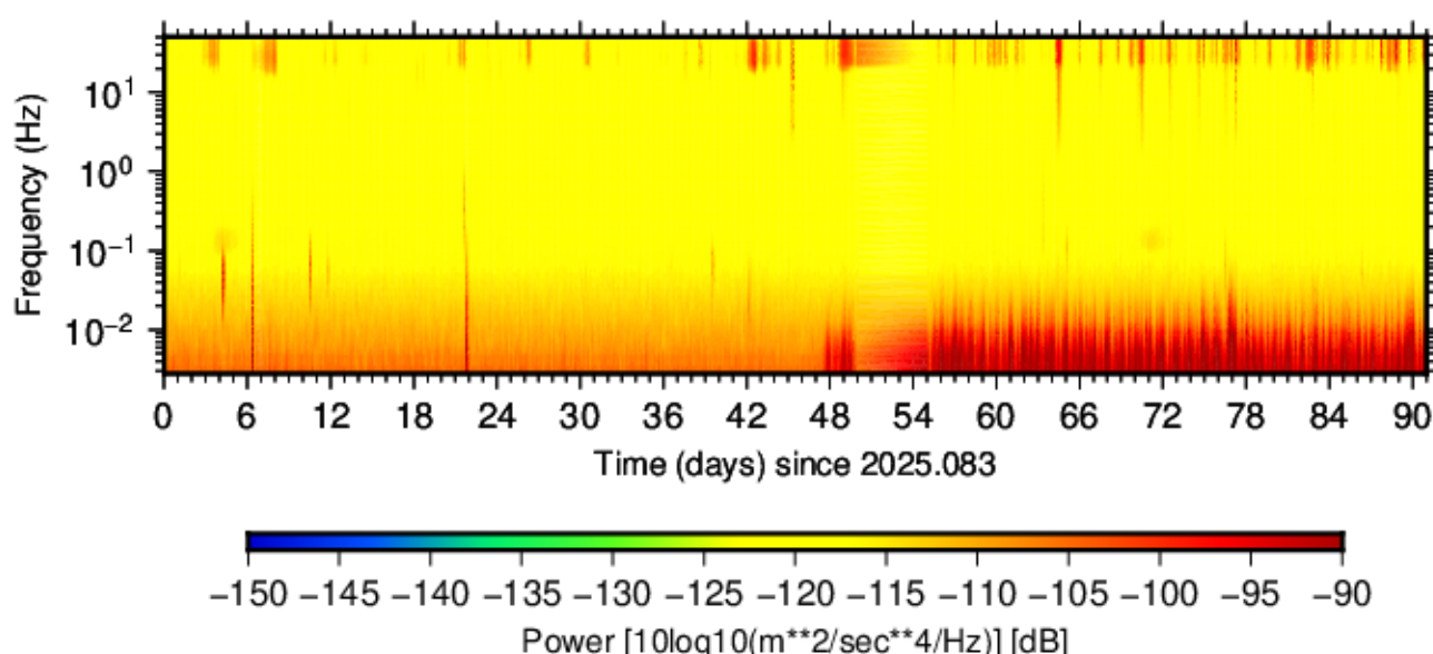
BK.YUBA.HNE.00 (2025.083 - 2025.173)
