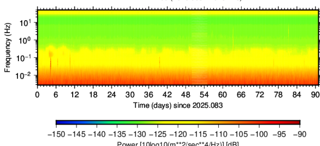
BK.YBH.HNN.00 (2025.083 - 2025.173)
