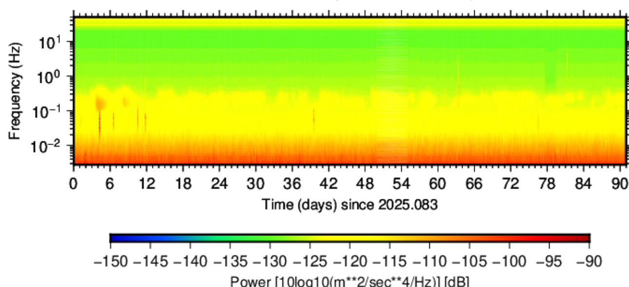
BK.YBH.HNZ.00 (2025.083 - 2025.173)
