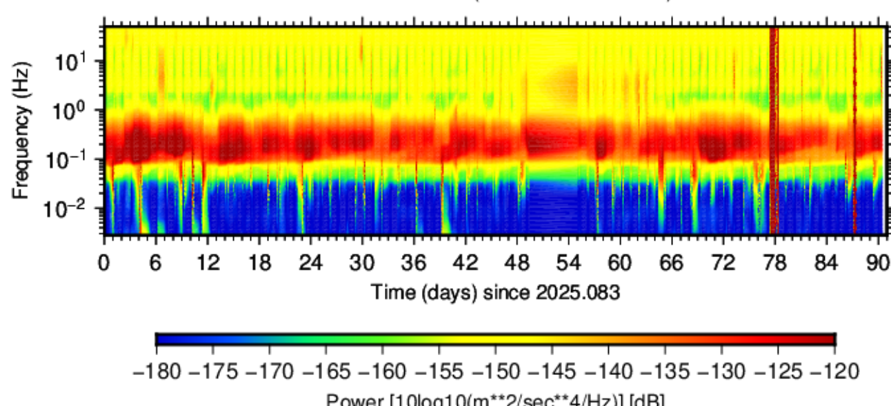
BK.YBH.HHZ.50 (2025.083 - 2025.173)
