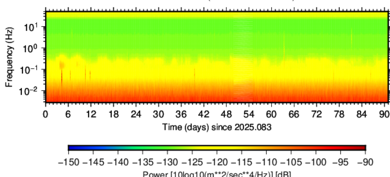
BK.YBH.HNE.00 (2025.083 - 2025.173)
