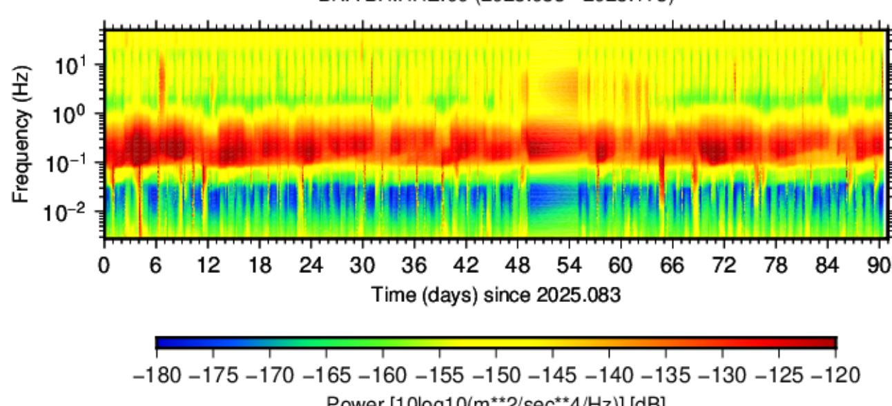
BK.YBH.HHE.00 (2025.083 - 2025.173)
