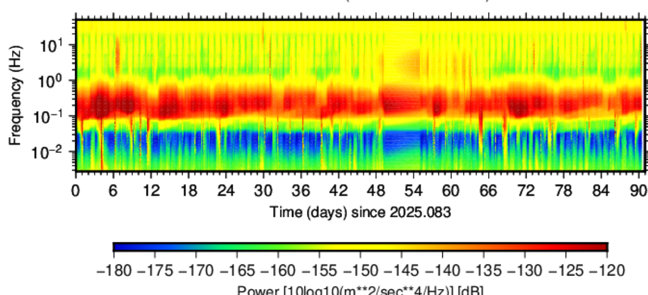
BK.YBH.HHN.00 (2025.083 - 2025.173)
