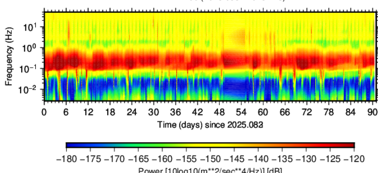
BK.YBH.HHZ.00 (2025.083 - 2025.173)
