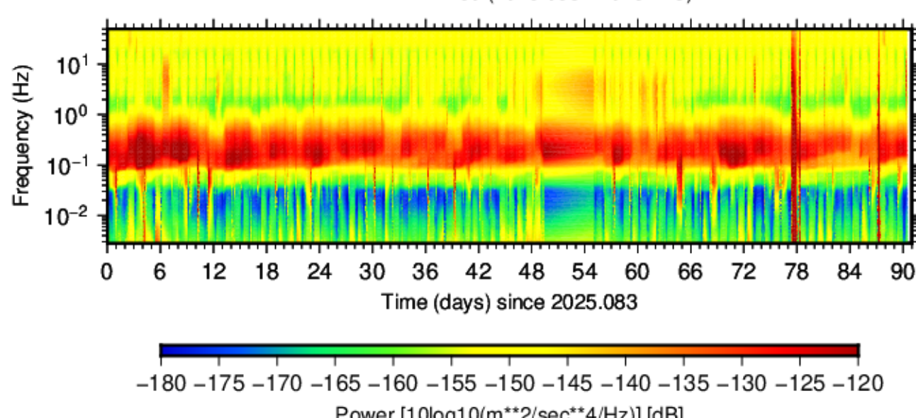
BK.YBH.HHE.50 (2025.083 - 2025.173)
