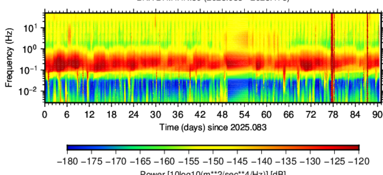
BK.YBH.HHN.50 (2025.083 - 2025.173)
