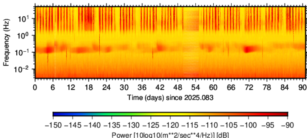
BK.WSRE.HNE.00 (2025.083 - 2025.173)
