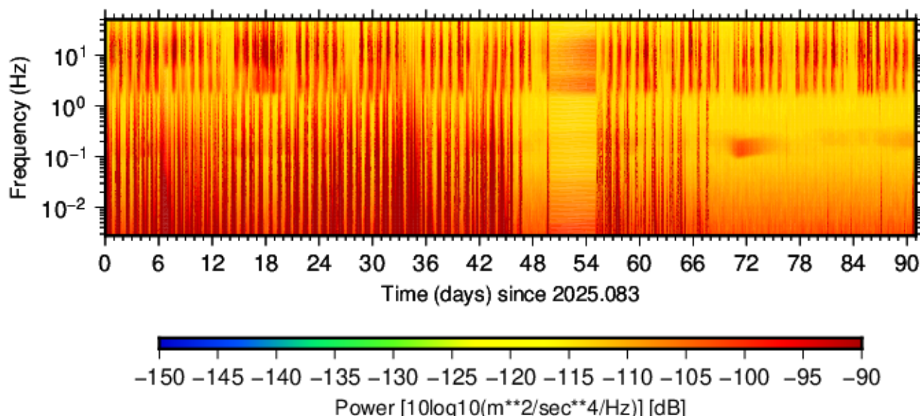
BK.WSRE.HNZ.00 (2025.083 - 2025.173)
