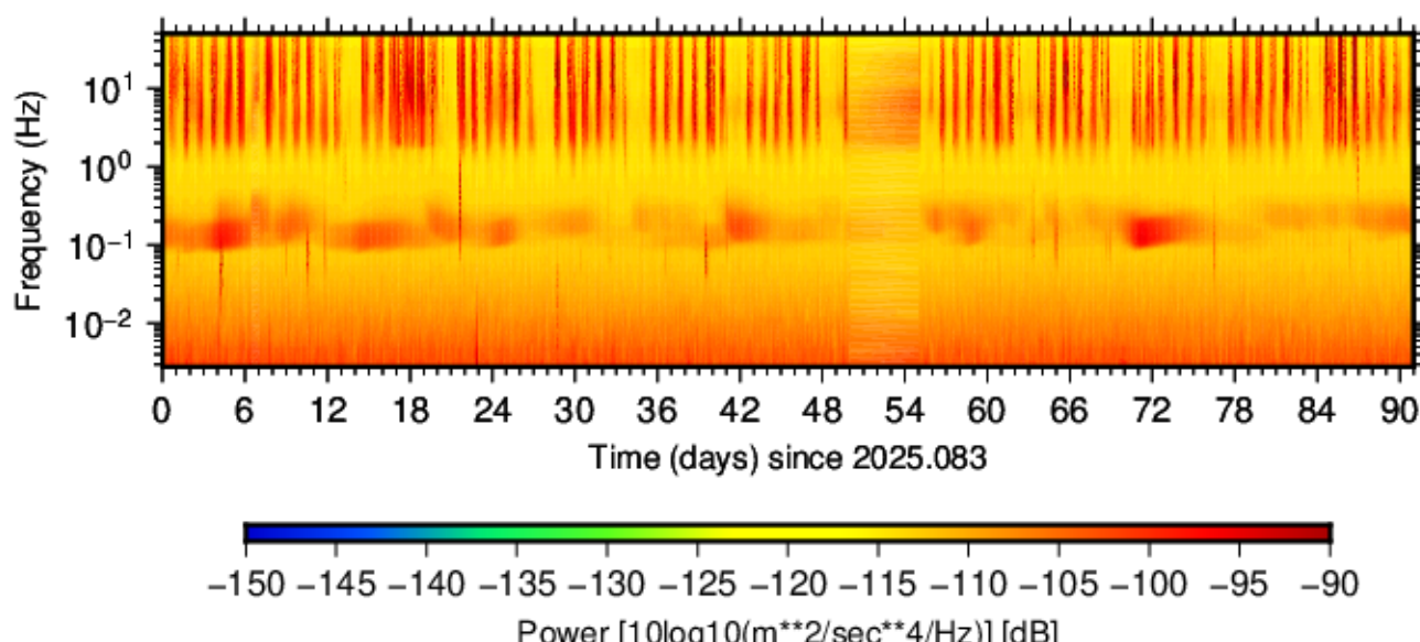
BK.WSRE.HNN.00 (2025.083 - 2025.173)
