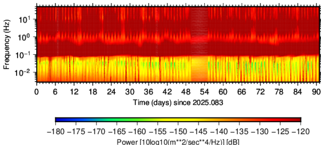
BK.WSRE.HHE.00 (2025.083 - 2025.173)
