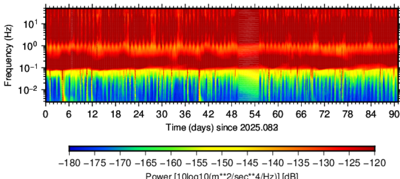
BK.WSRE.HHZ.00 (2025.083 - 2025.173)
