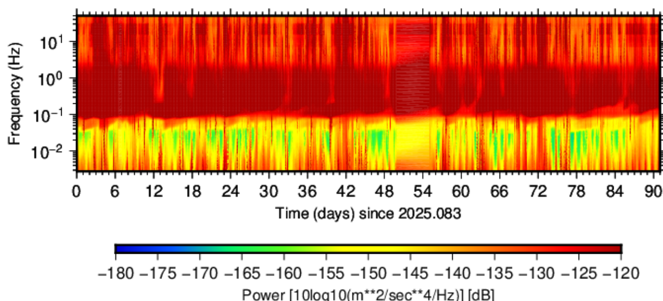
BK.WLKR.HHE.00 (2025.083 - 2025.173)
