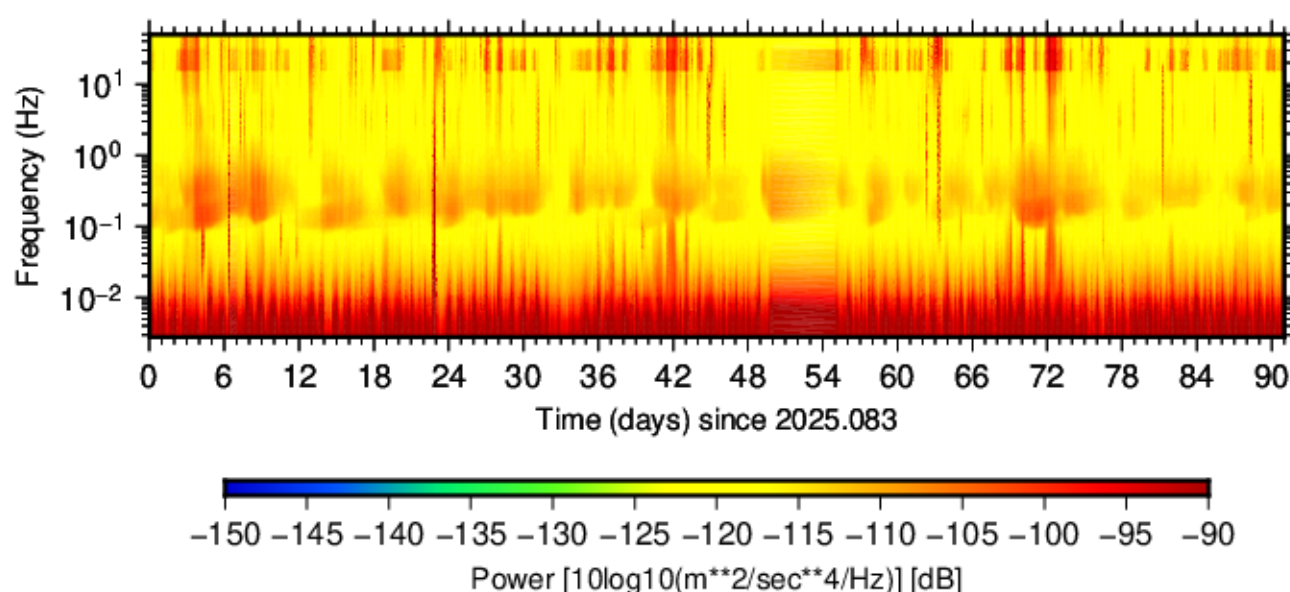
BK.WLKR.HNN.00 (2025.083 - 2025.173)
