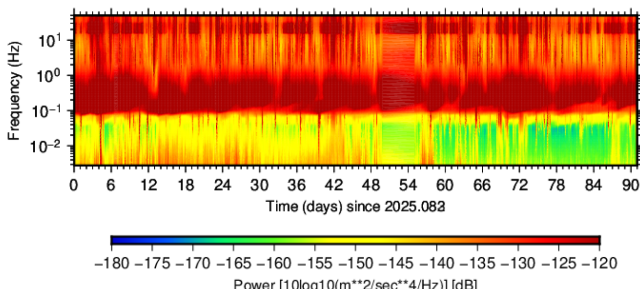
BK.WLKR.HHZ.00 (2025.083 - 2025.173)
