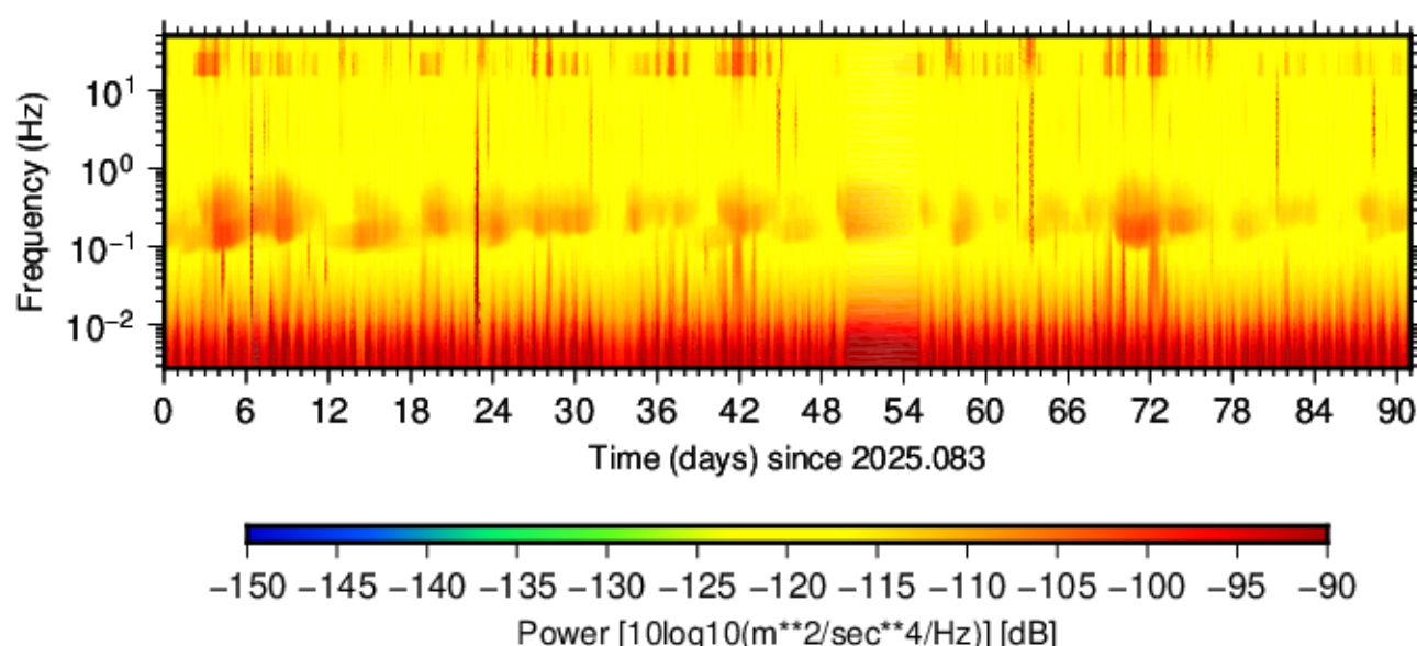
BK.WLKR.HNZ.00 (2025.083 - 2025.173)
