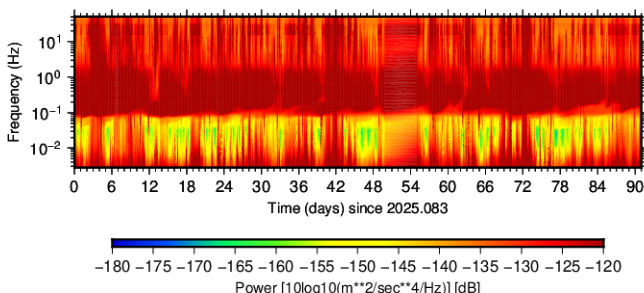
BK.WLKR.HHN.00 (2025.083 - 2025.173)
