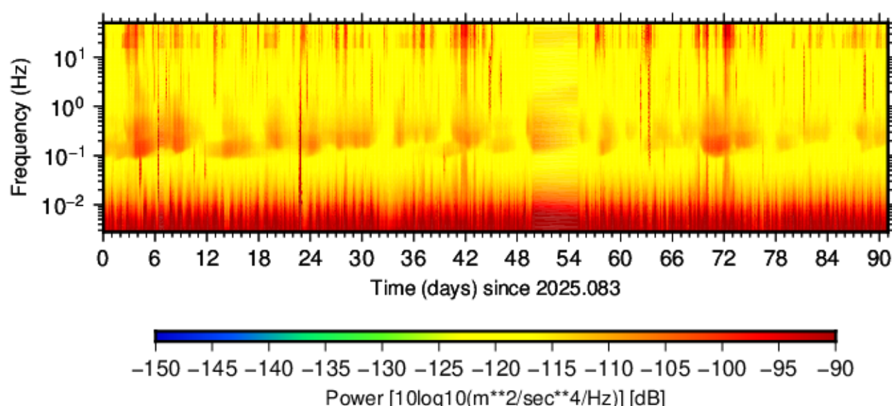
BK.WLKR.HNE.00 (2025.083 - 2025.173)
