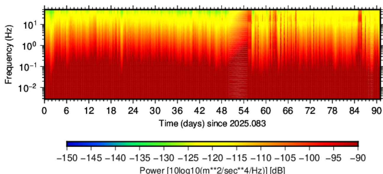
BK.WENL.HNZ.00 (2025.083 - 2025.173)
