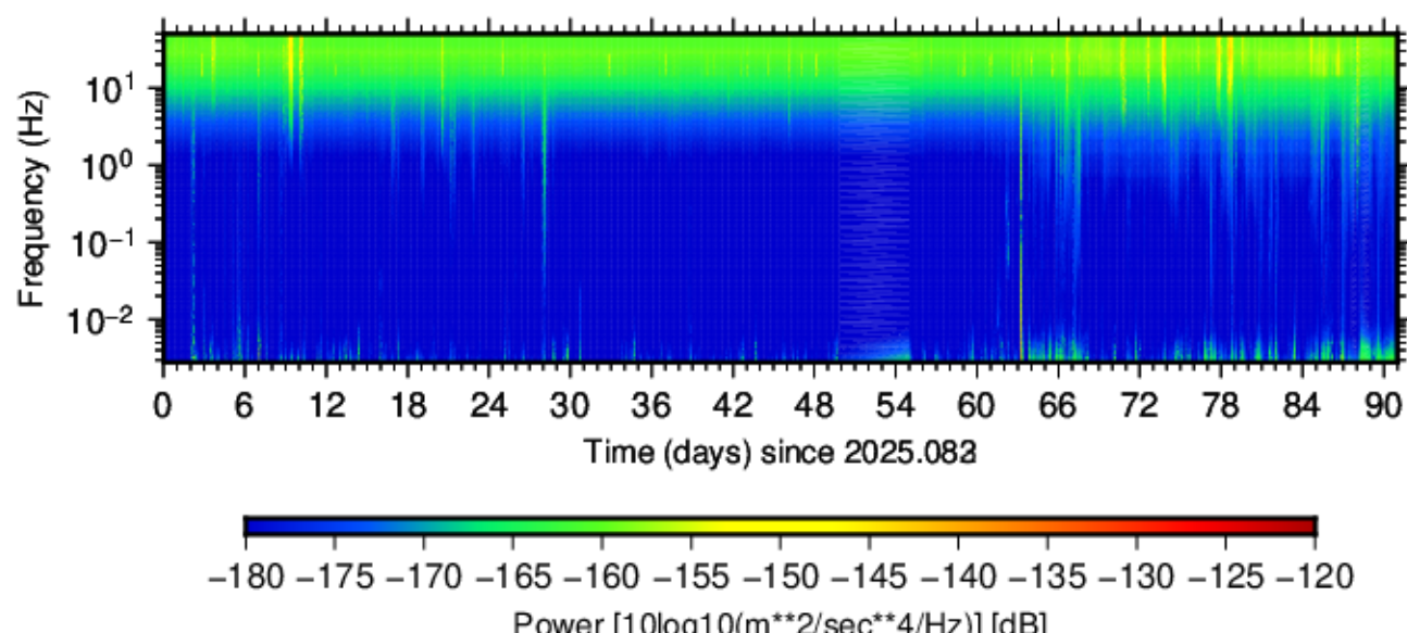
BK.WENL.HHZ.00 (2025.083 - 2025.173)
