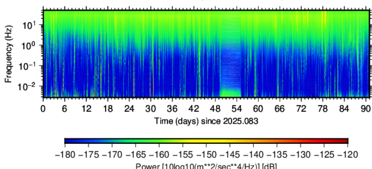
BK.WENL.HHE.00 (2025.083 - 2025.173)
