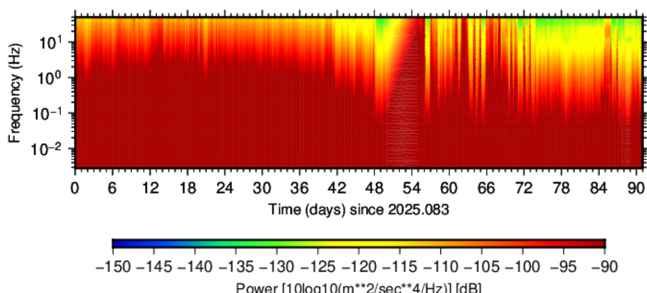
BK.WENL.HNN.00 (2025.083 - 2025.173)
