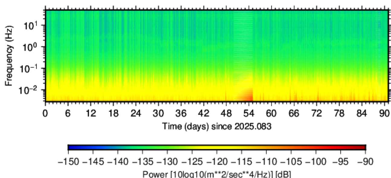
BK.WENL.HNE.00 (2025.083 - 2025.173)
