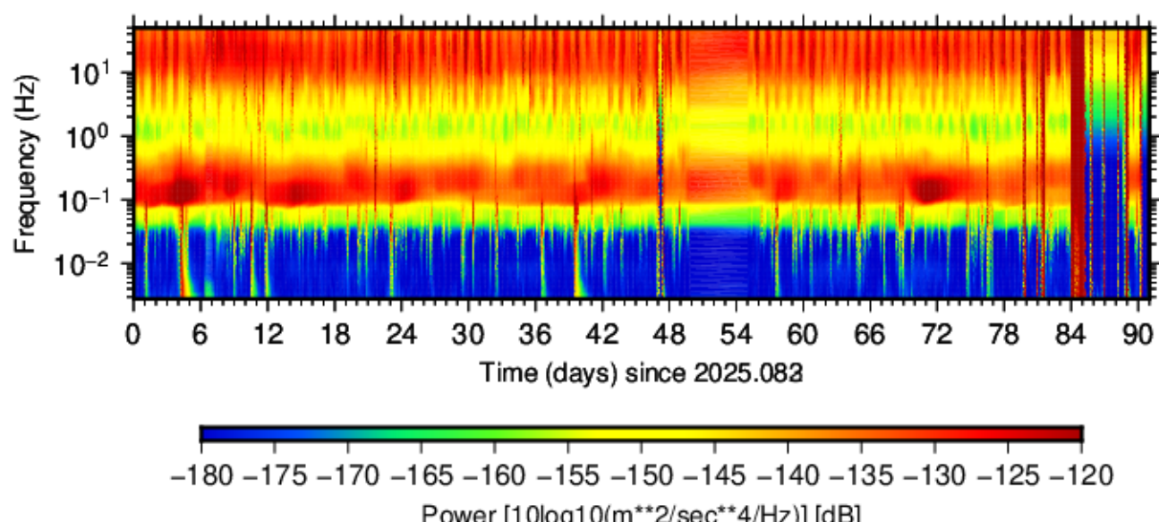
BK.WEBR.HHZ.00 (2025.083 - 2025.173)
