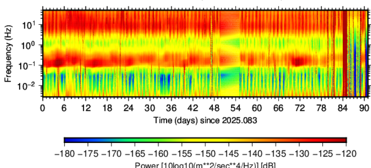
BK.WEBR.HHE.00 (2025.083 - 2025.173)
