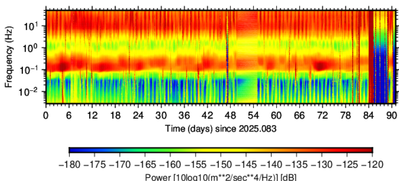
BK.WEBR.HHN.00 (2025.083 - 2025.173)
