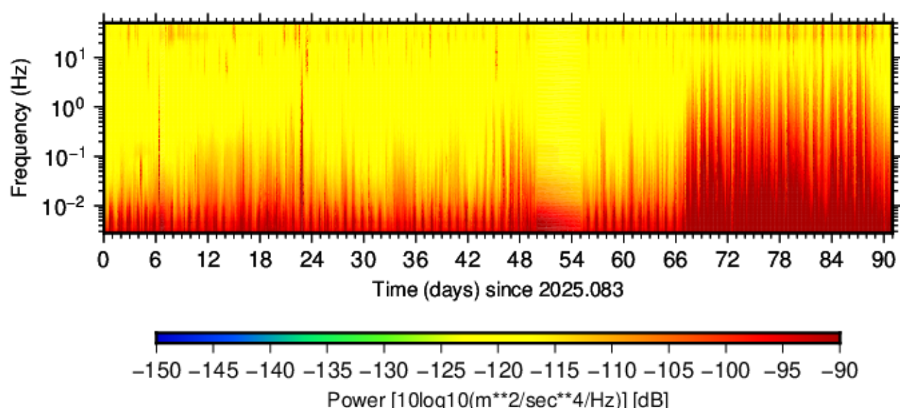
BK.WEBR.HNE.00 (2025.083 - 2025.173)
