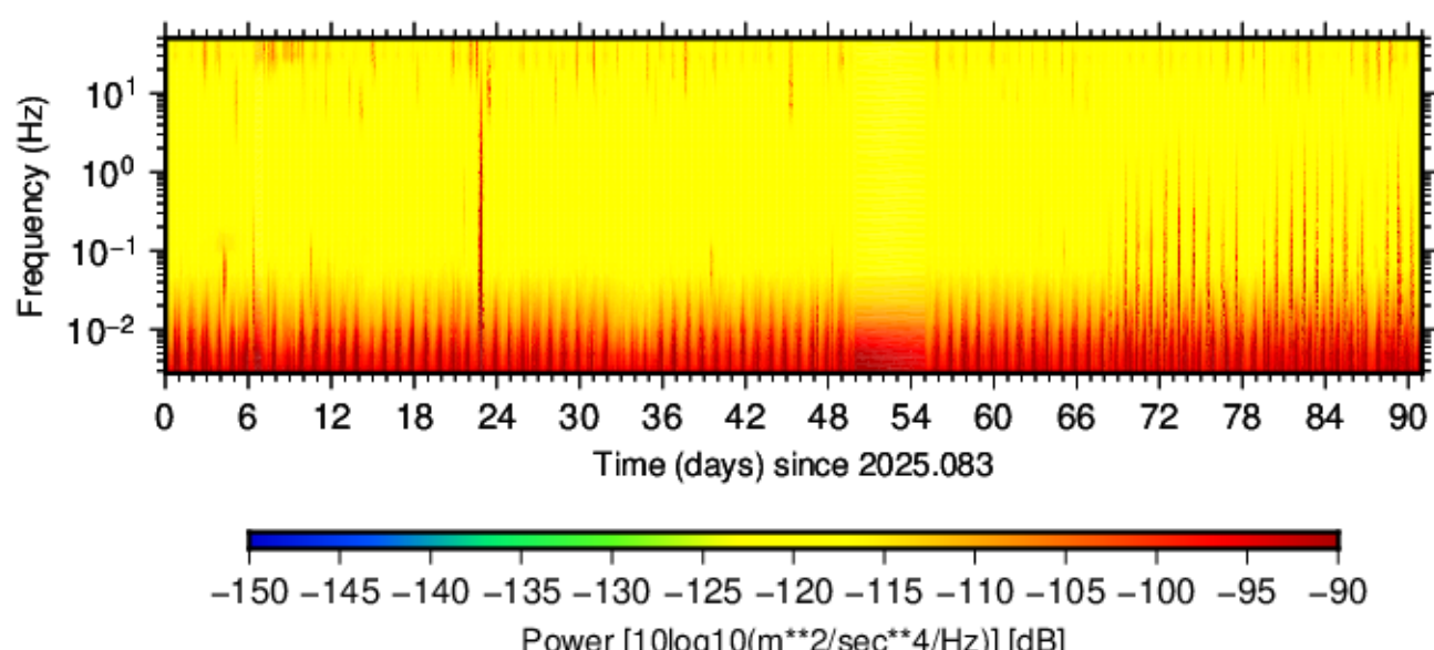
BK.WEBR.HNN.00 (2025.083 - 2025.173)
