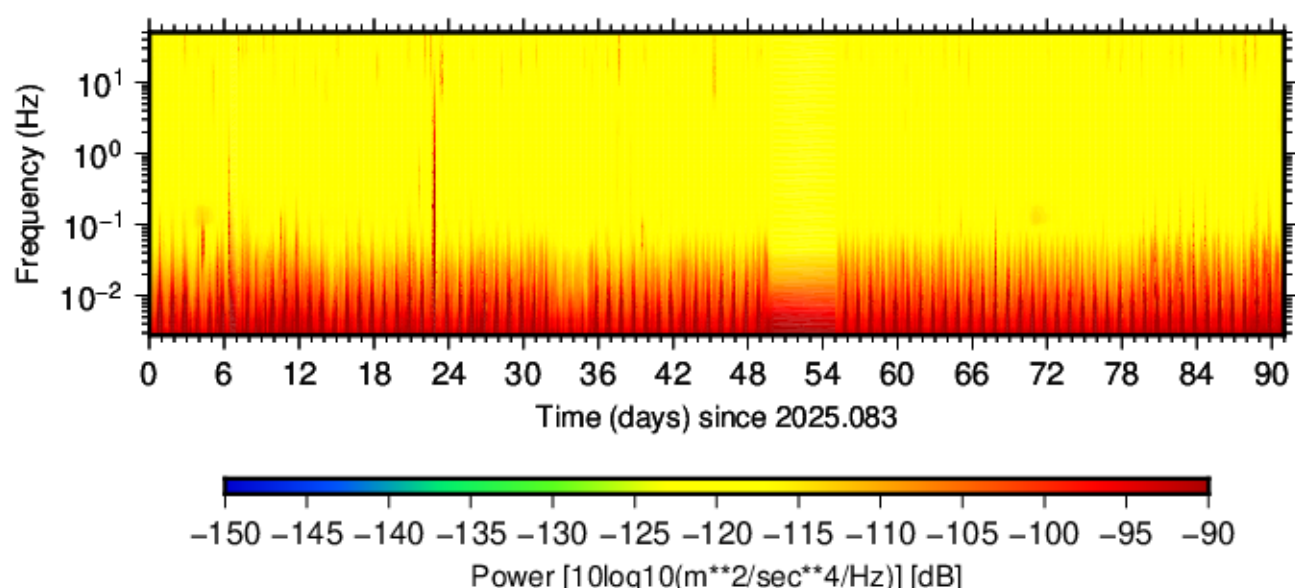
BK.WEBR.HNZ.00 (2025.083 - 2025.173)
