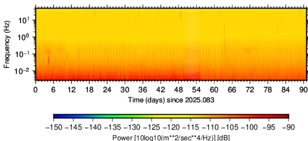
BK.WEAV.HNN.00 (2025.083 - 2025.173)
