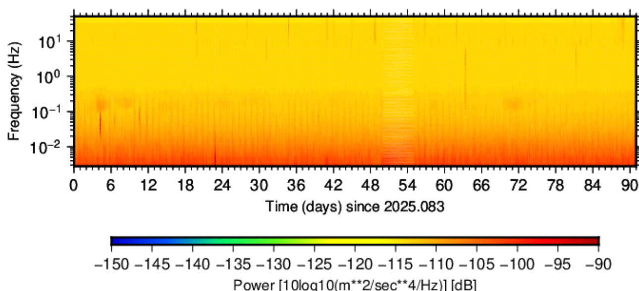
BK.WEAV.HNE.00 (2025.083 - 2025.173)
