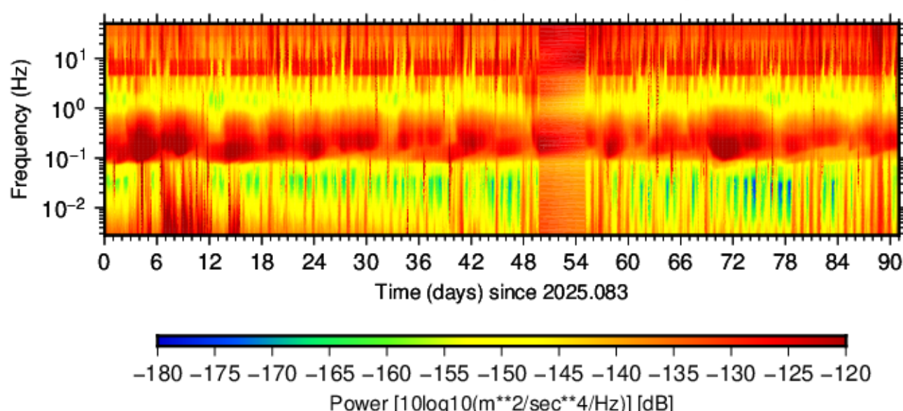
BK.WEAV.HHN.00 (2025.083 - 2025.173)
