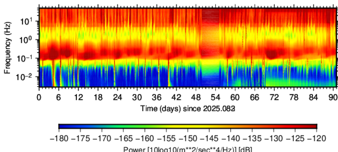
BK.WEAV.HHZ.00 (2025.083 - 2025.173)
