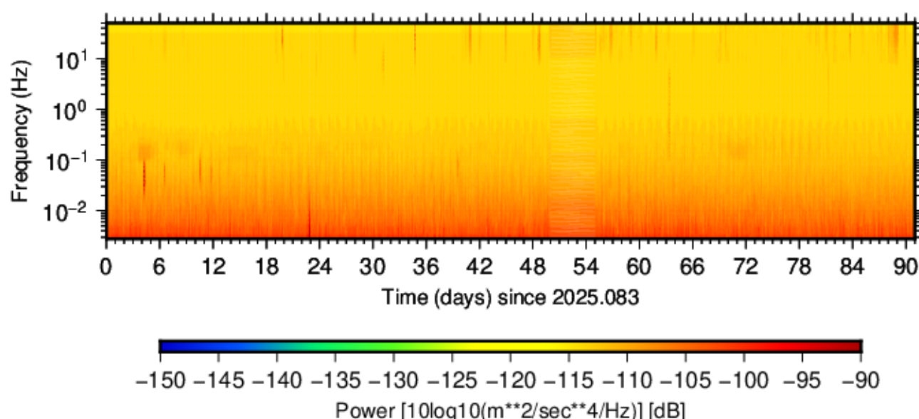
BK.WEAV.HNZ.00 (2025.083 - 2025.173)
