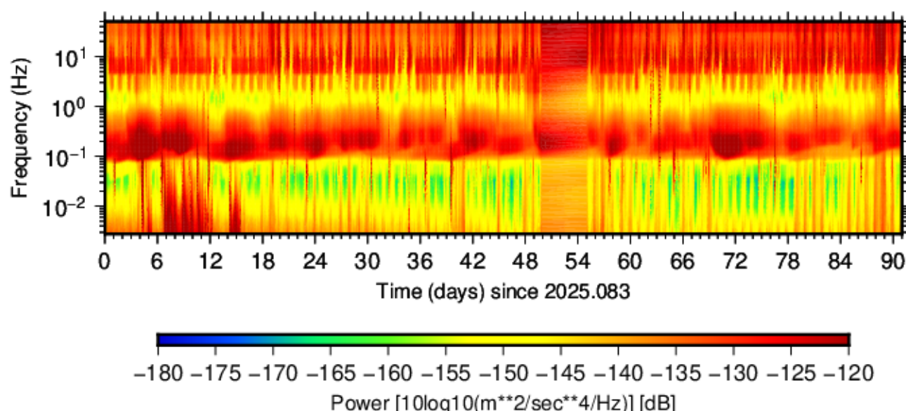
BK.WEAV.HHE.00 (2025.083 - 2025.173)
