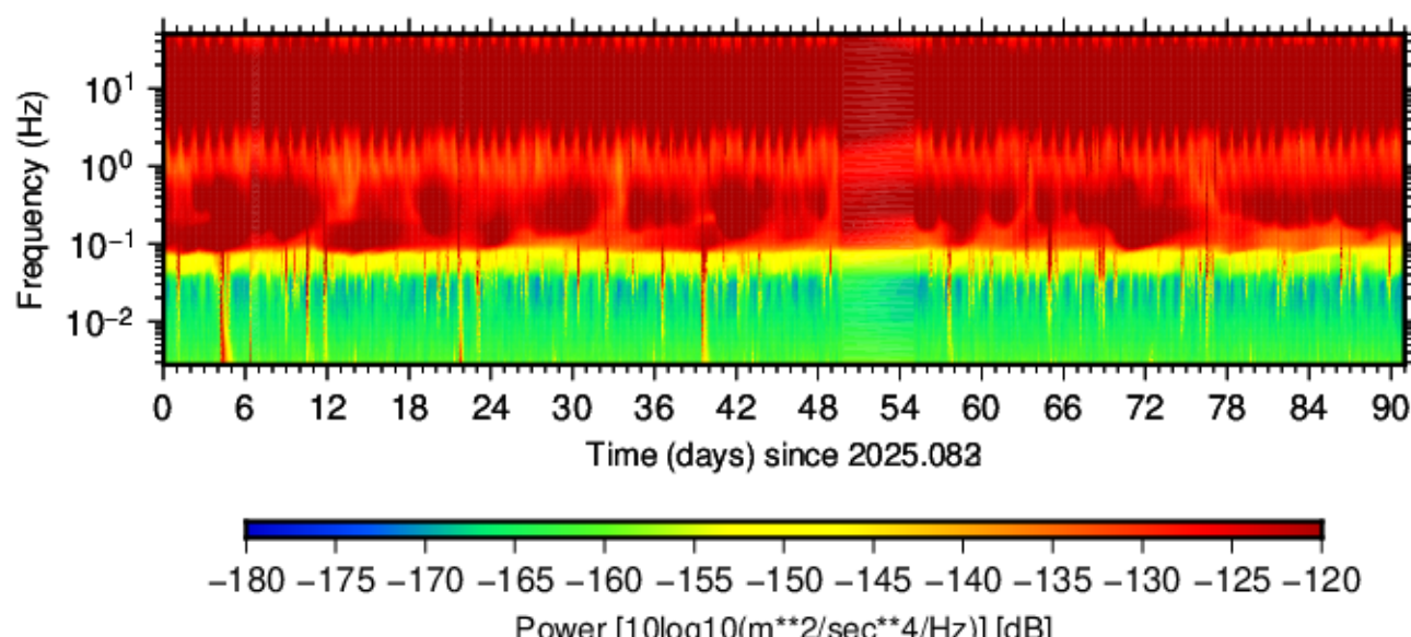
BK.VAK.HHZ.00 (2025.083 - 2025.173)
