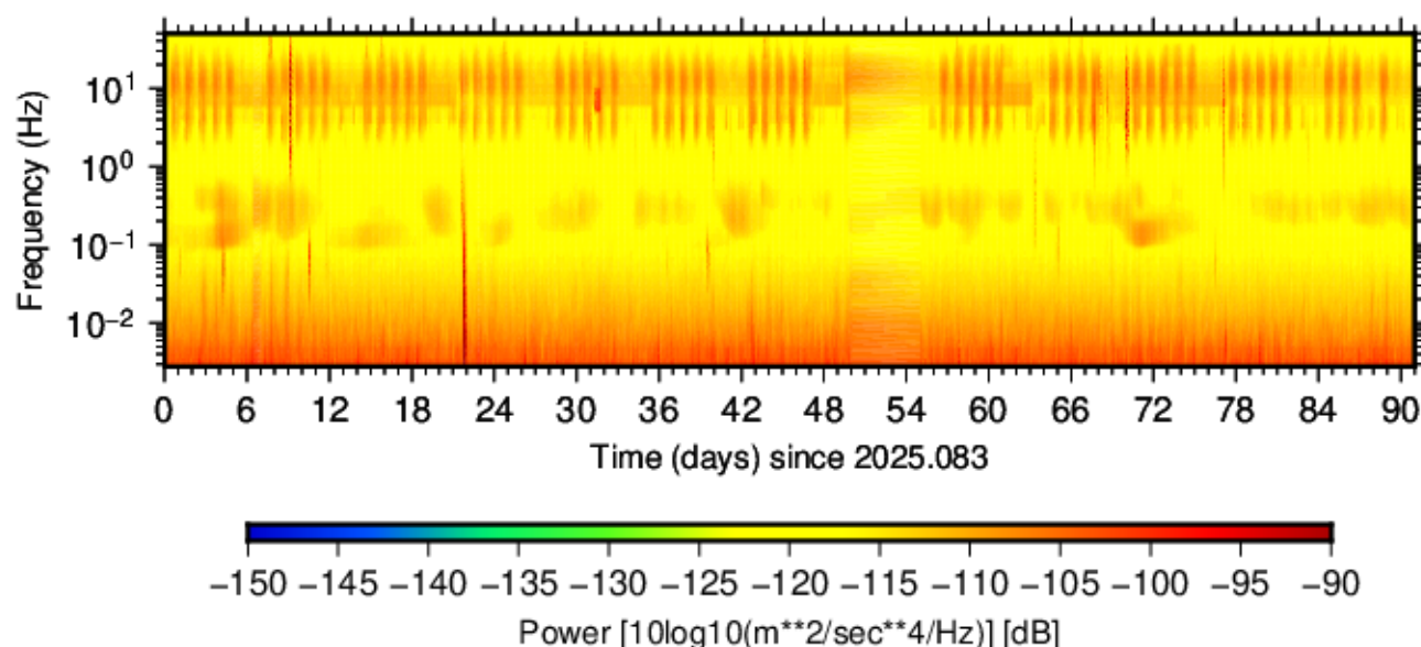
BK.VAK.HNN.00 (2025.083 - 2025.173)
