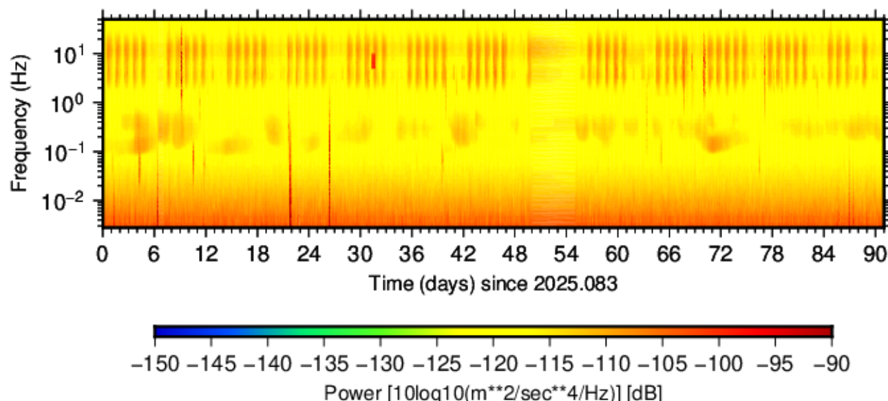
BK.VAK.HNE.00 (2025.083 - 2025.173)
