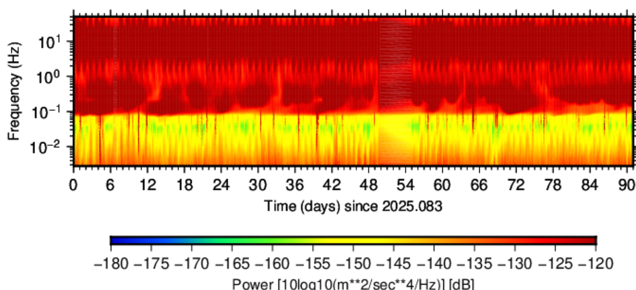
BK.VAK.HHN.00 (2025.083 - 2025.173)
