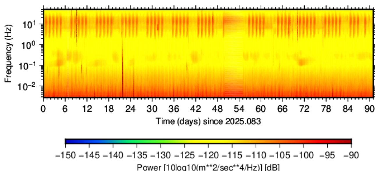
BK.VAK.HNZ.00 (2025.083 - 2025.173)
