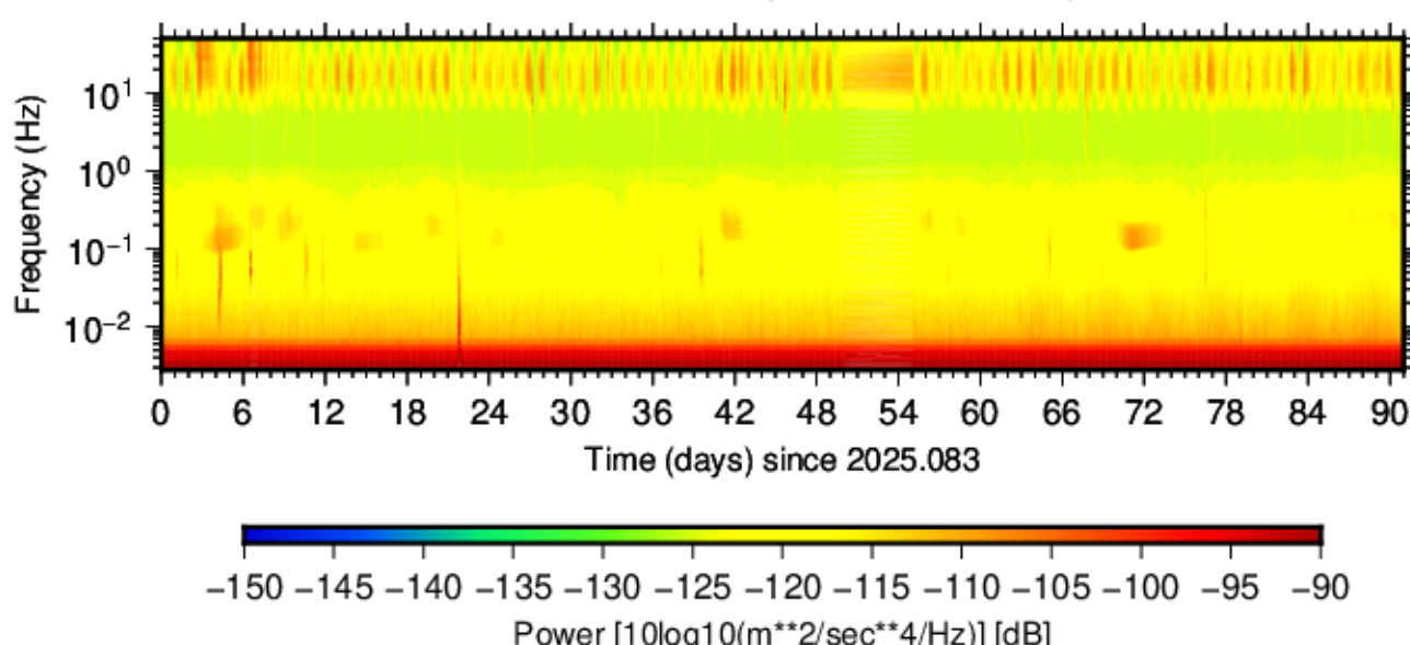
BK.UMUN.HNZ.00 (2025.083 - 2025.173)
