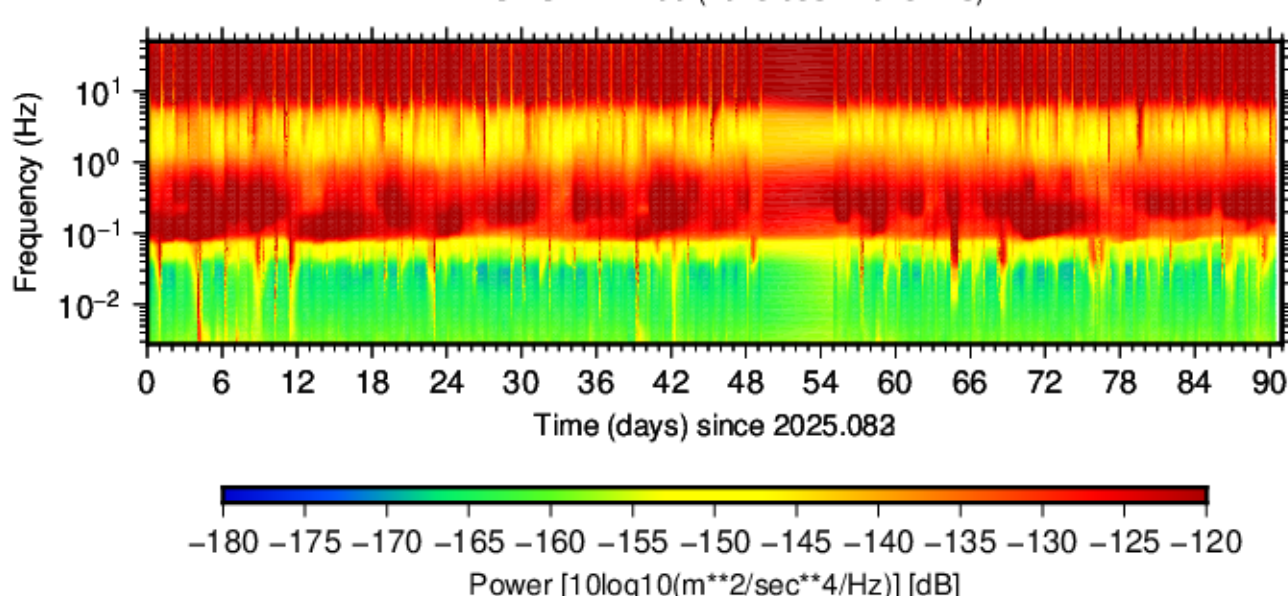
BK.UMUN.HHZ.00 (2025.083 - 2025.173)
