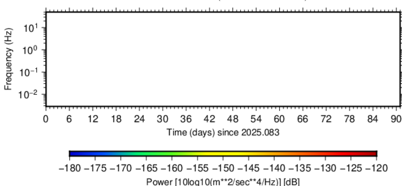
BK.UMUN.HHZ.50 (2025.083 - 2025.173)
