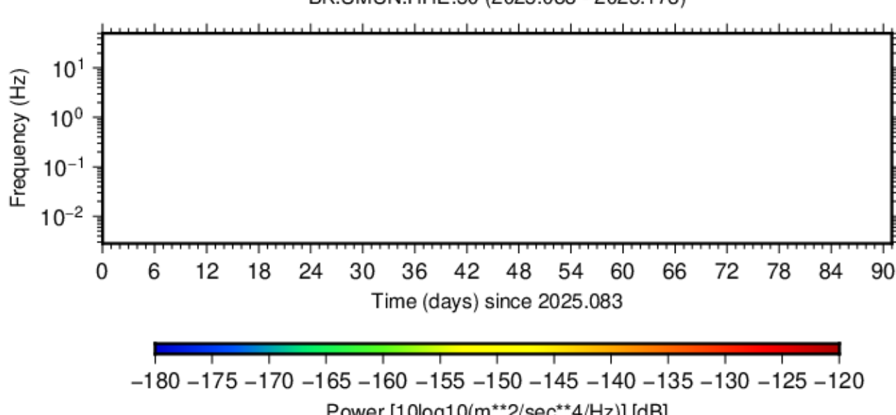
BK.UMUN.HHE.50 (2025.083 - 2025.173)
