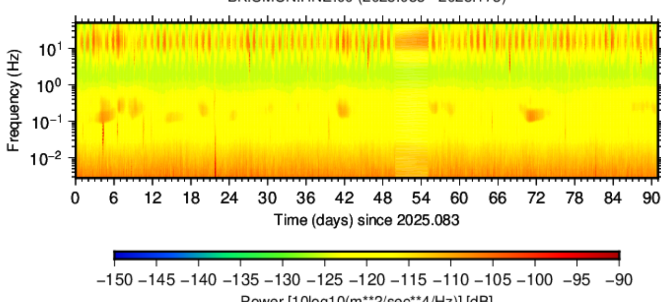
BK.UMUN.HNE.00 (2025.083 - 2025.173)
