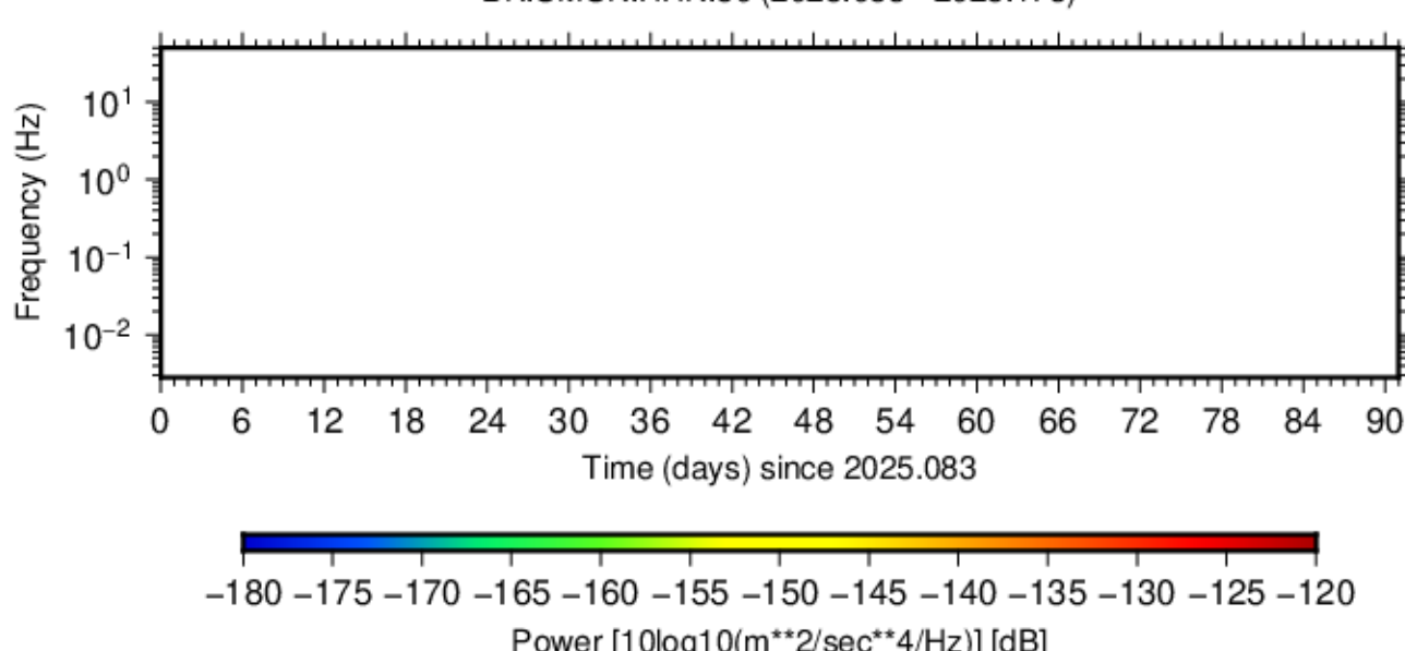
BK.UMUN.HHN.50 (2025.083 - 2025.173)
