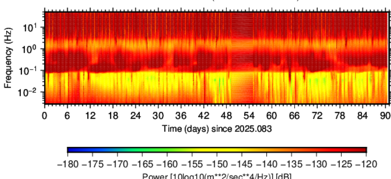
BK.UMUN.HHN.00 (2025.083 - 2025.173)
