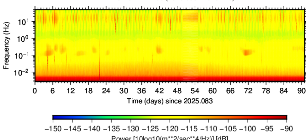
BK.UMUN.HNN.00 (2025.083 - 2025.173)
