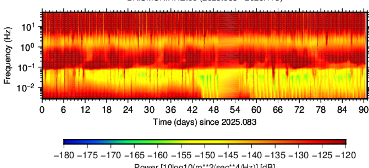
BK.UMUN.HHE.00 (2025.083 - 2025.173)
