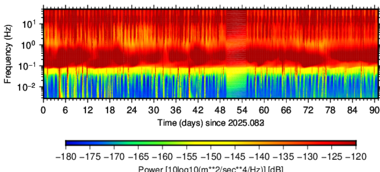
BK.TSCN.HHZ.00 (2025.083 - 2025.173)
