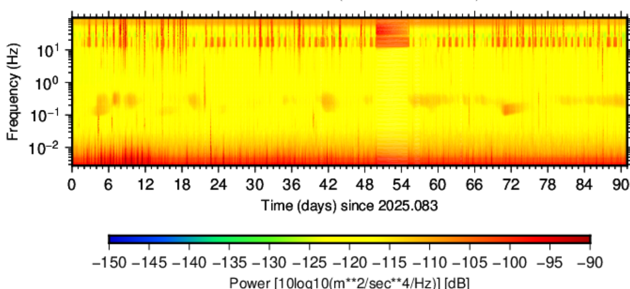
BK.TSCN.HNZ.00 (2025.083 - 2025.173)
