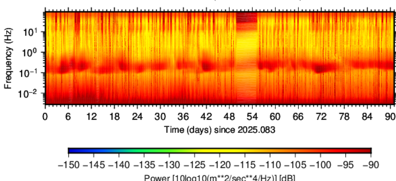
BK.TSCN.HNN.00 (2025.083 - 2025.173)
