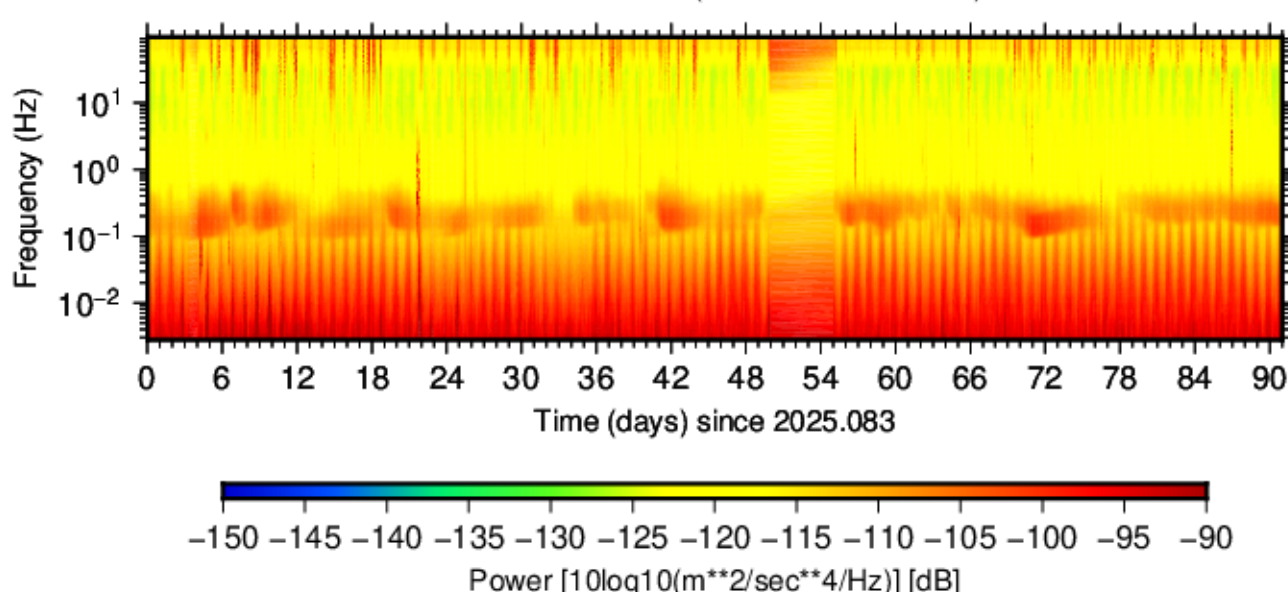
BK.TSCN.HNE.00 (2025.083 - 2025.173)
