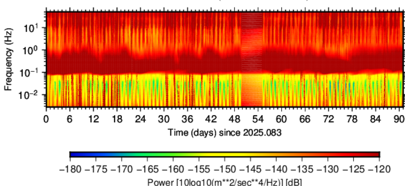
BK.TSCN.HHN.00 (2025.083 - 2025.173)
