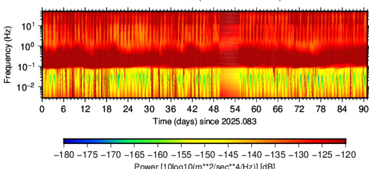
BK.TSCN.HHE.00 (2025.083 - 2025.173)
