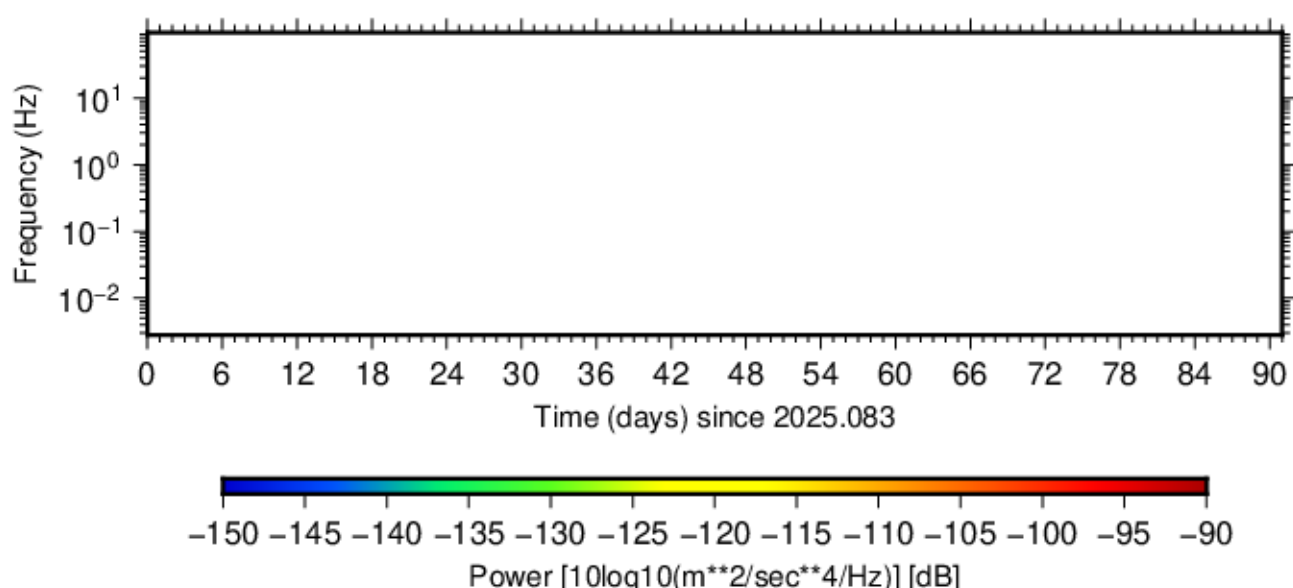
BK.TRAM.HNZ.00 (2025.083 - 2025.173)
