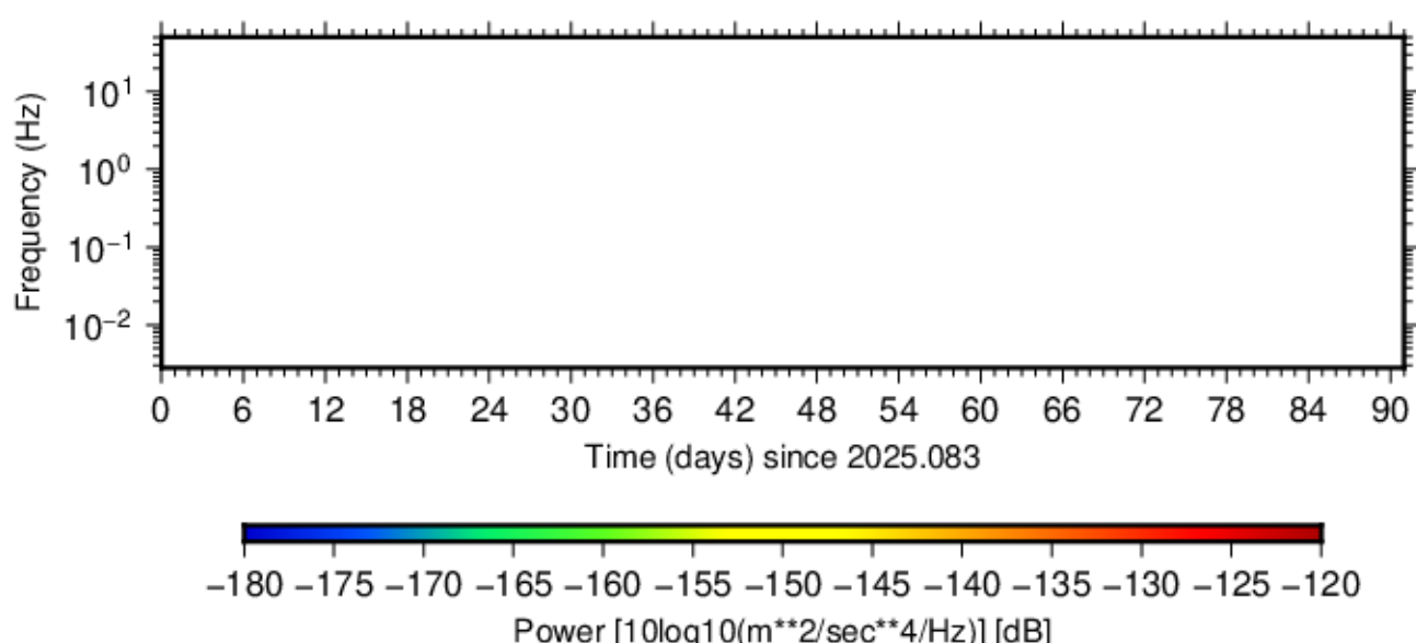
BK.TRAM.HHN.00 (2025.083 - 2025.173)
