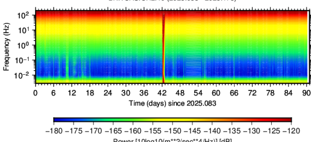
BK.TCAS.CH2.40 (2025.083 - 2025.173)
