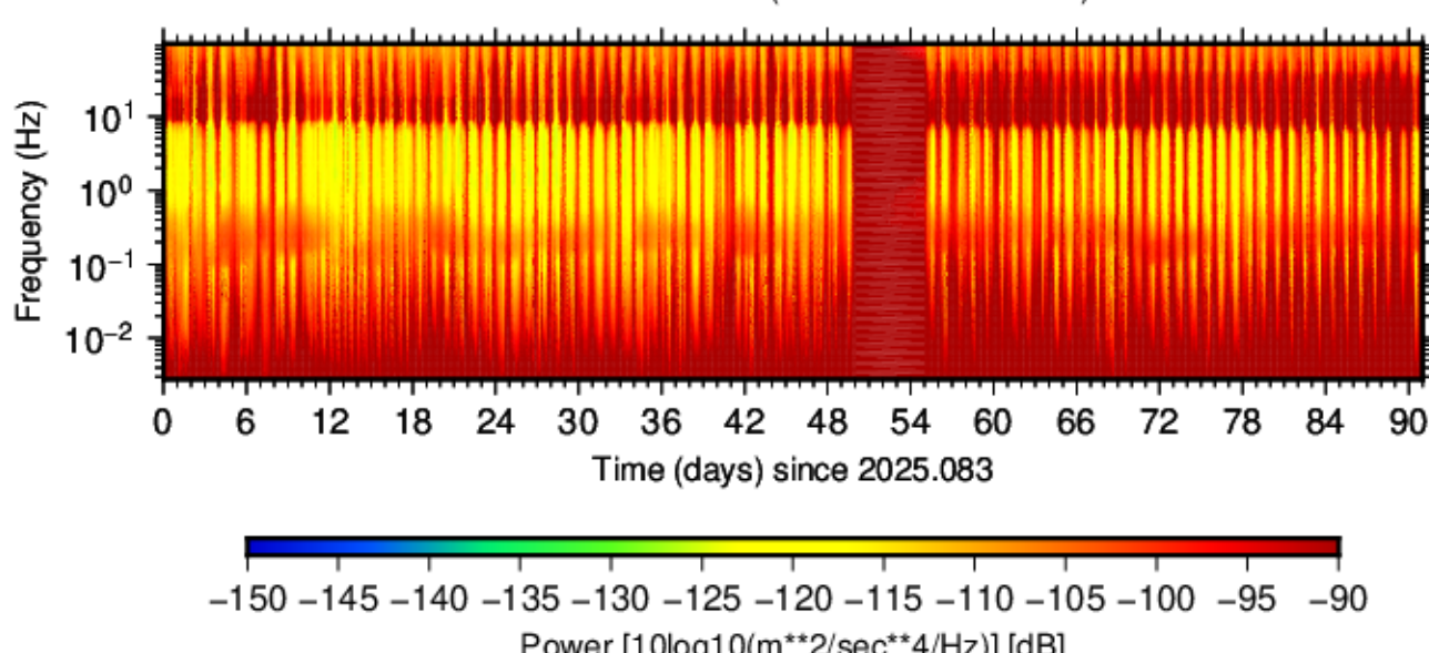
BK.TCAS.HNN.00 (2025.083 - 2025.173)
