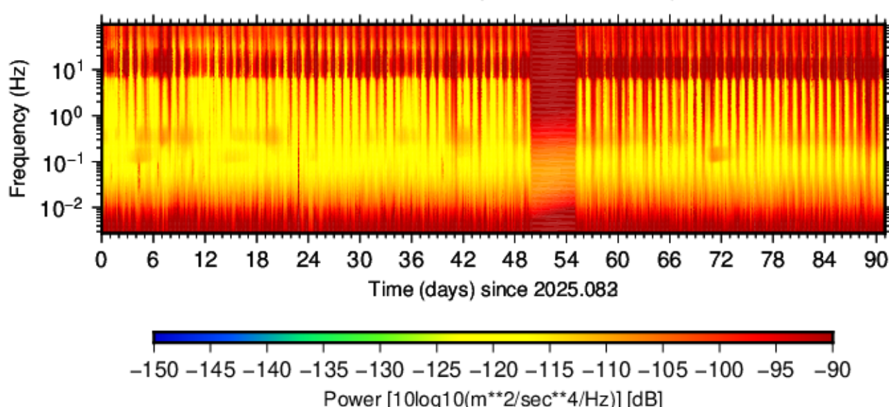
BK.TCAS.HNZ.00 (2025.083 - 2025.173)
