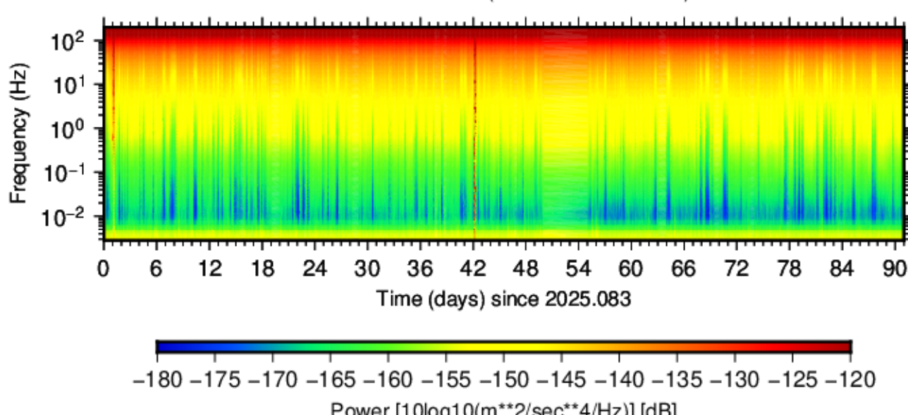
BK.TCAS.CH1.40 (2025.083 - 2025.173)
