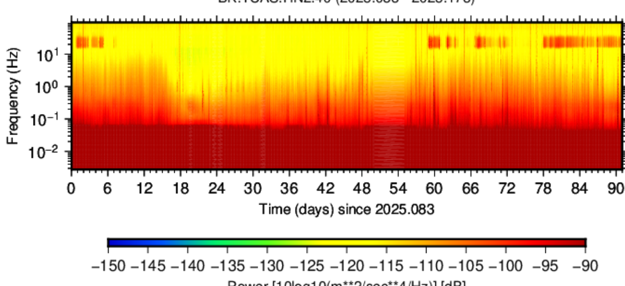
BK.TCAS.HN2.40 (2025.083 - 2025.173)
