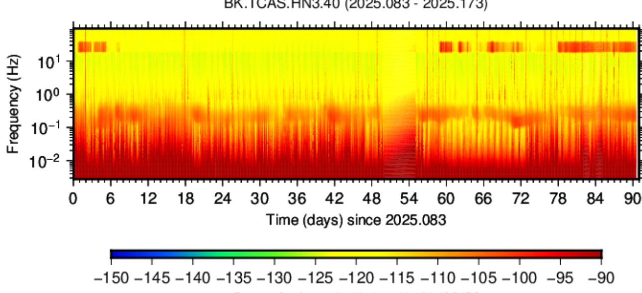
BK.TCAS.HN3.40 (2025.083 - 2025.173)
