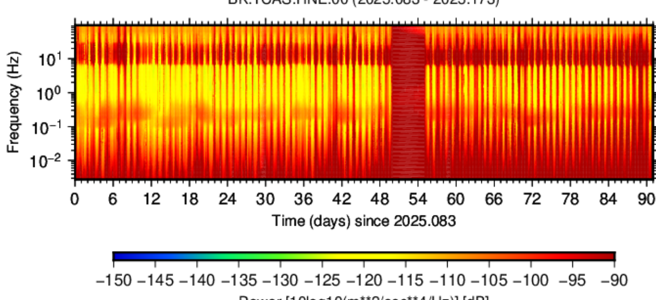
BK.TCAS.HNE.00 (2025.083 - 2025.173)
