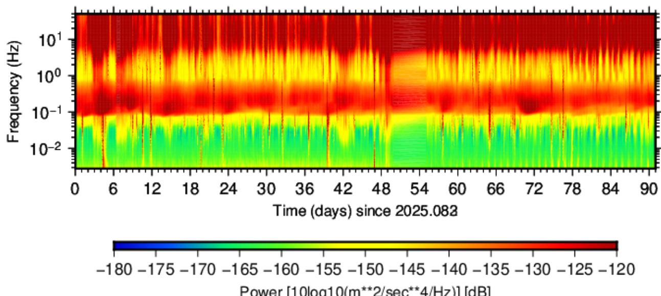
BK.SWNM.HHZ.00 (2025.083 - 2025.173)
