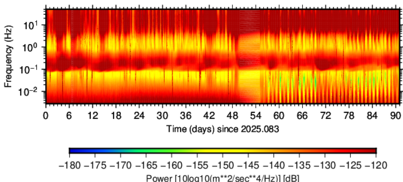
BK.SWNM.HHN.00 (2025.083 - 2025.173)
