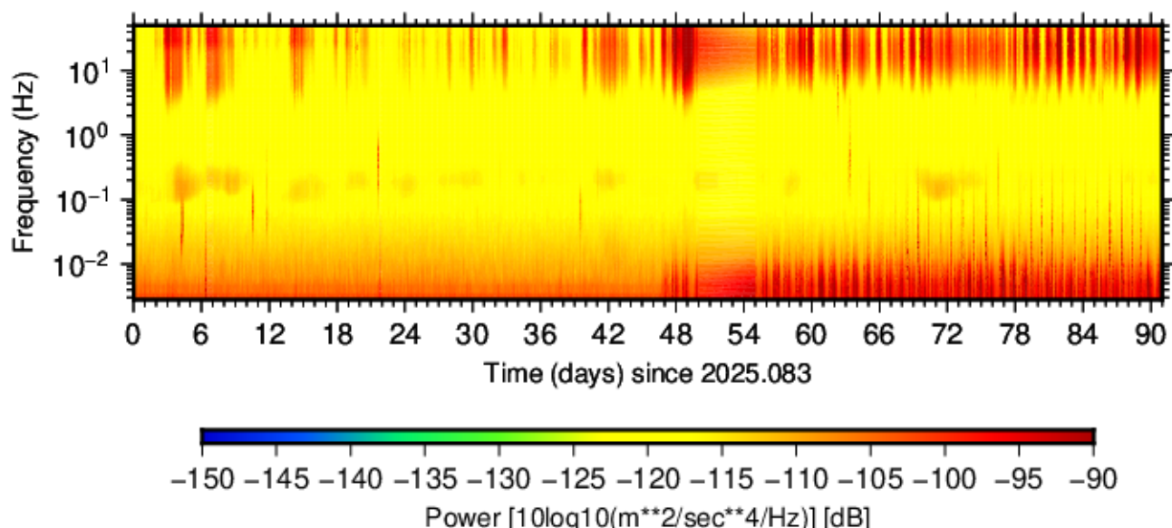
BK.SWNM.HNE.00 (2025.083 - 2025.173)
