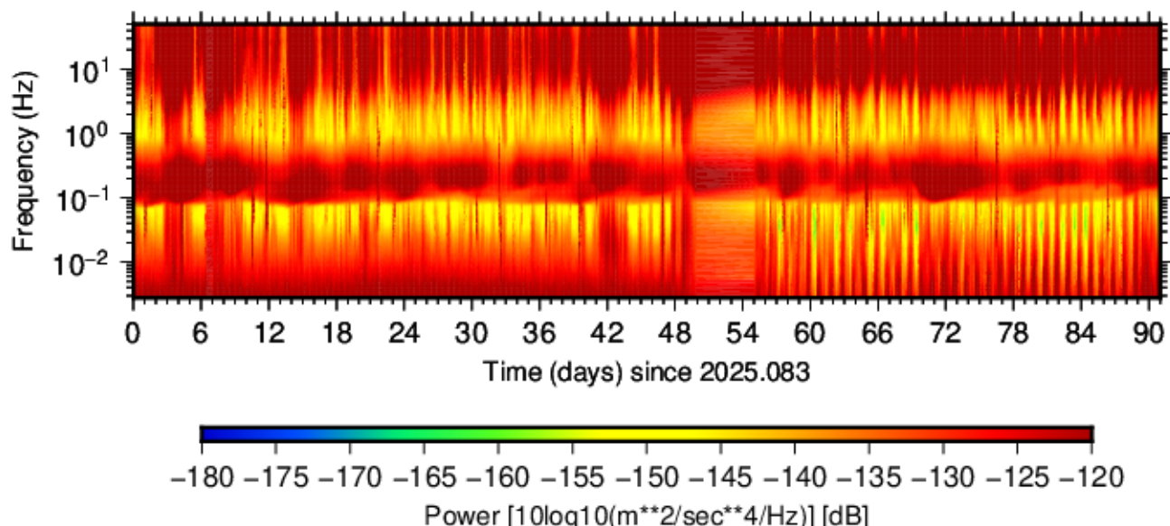
BK.SWNM.HHE.00 (2025.083 - 2025.173)
