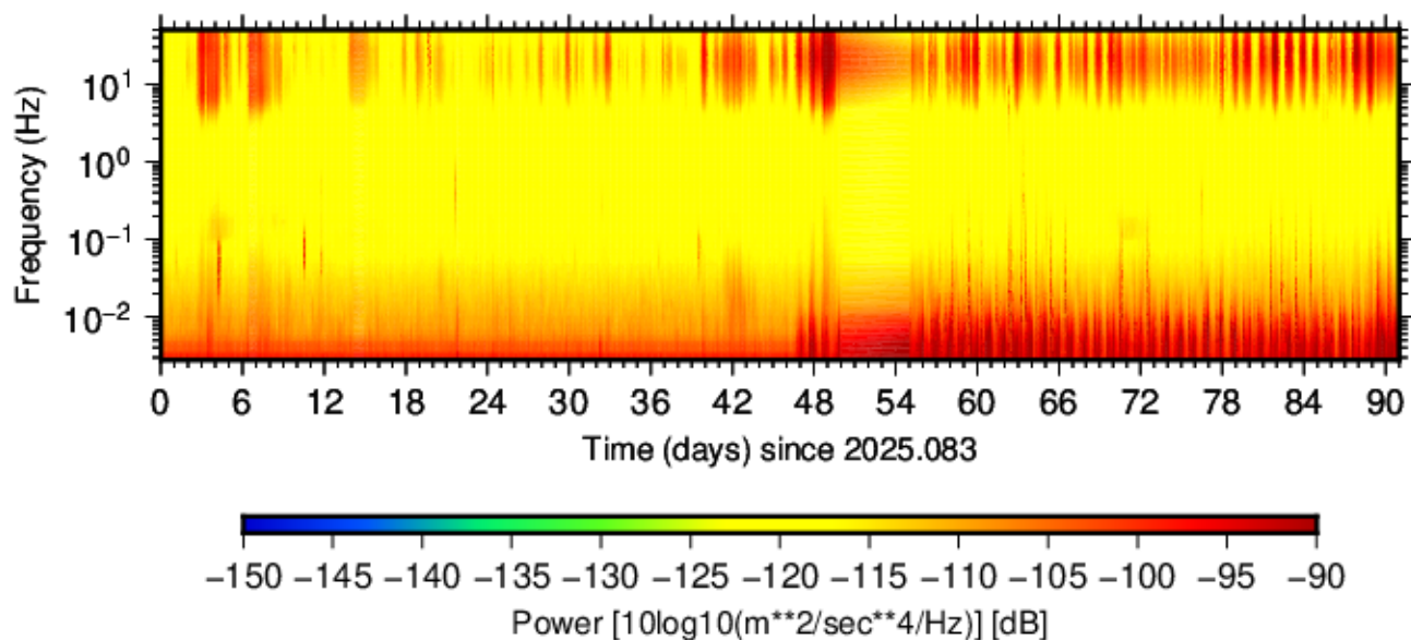
BK.SWNM.HNZ.00 (2025.083 - 2025.173)
