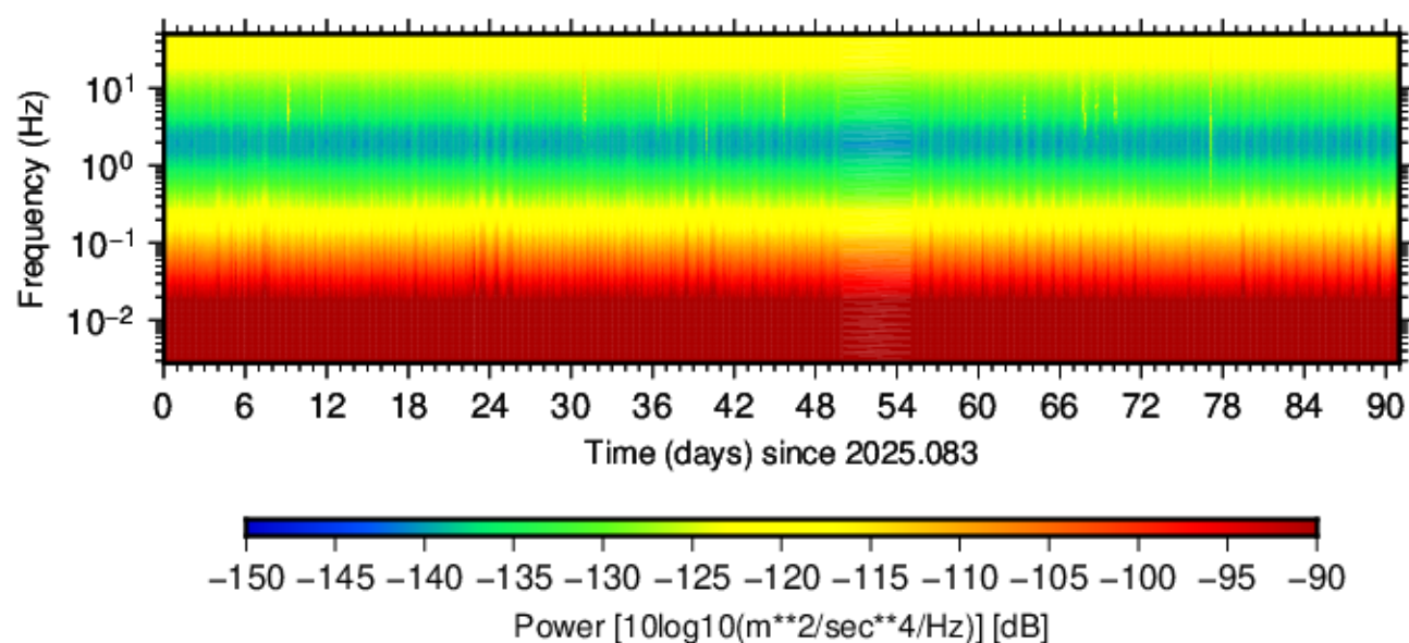
BK.SVIN.EP3.40 (2025.083 - 2025.173)
