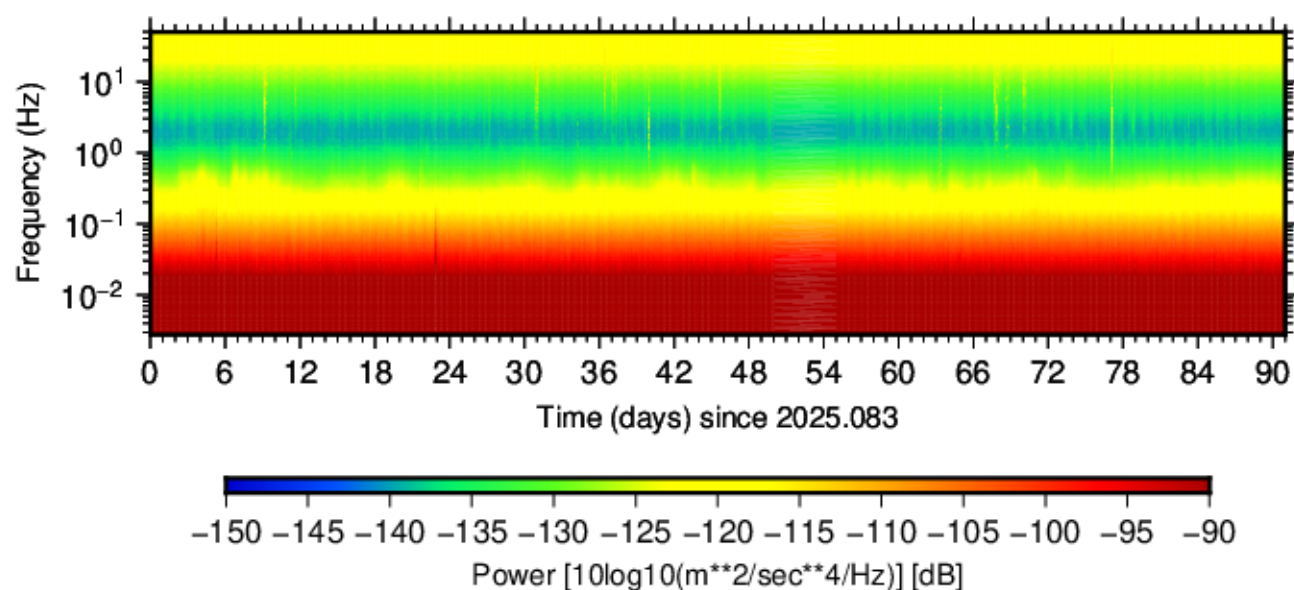
BK.SVIN.EP2.40 (2025.083 - 2025.173)
