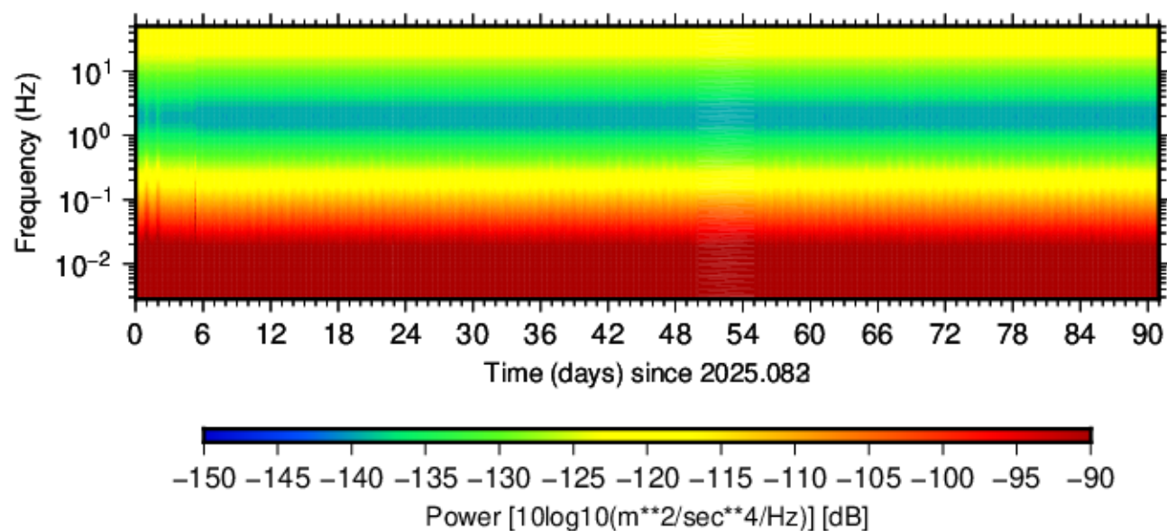
BK.SVIN.EP1.40 (2025.083 - 2025.173)
