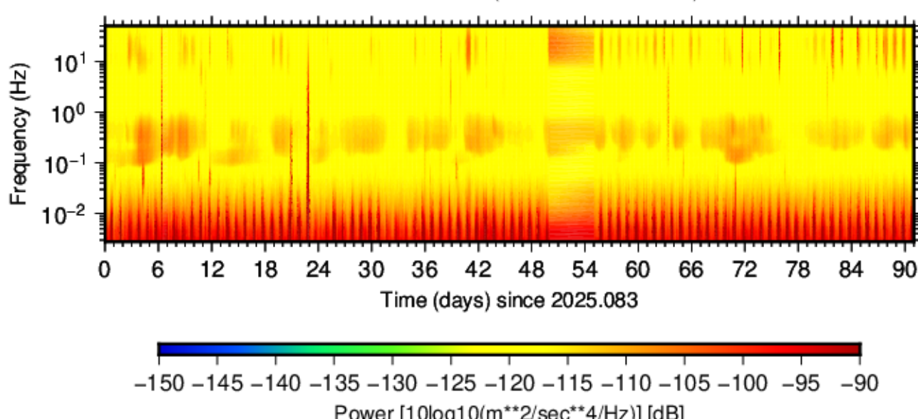
BK.SPAN.HNZ.00 (2025.083 - 2025.173)
