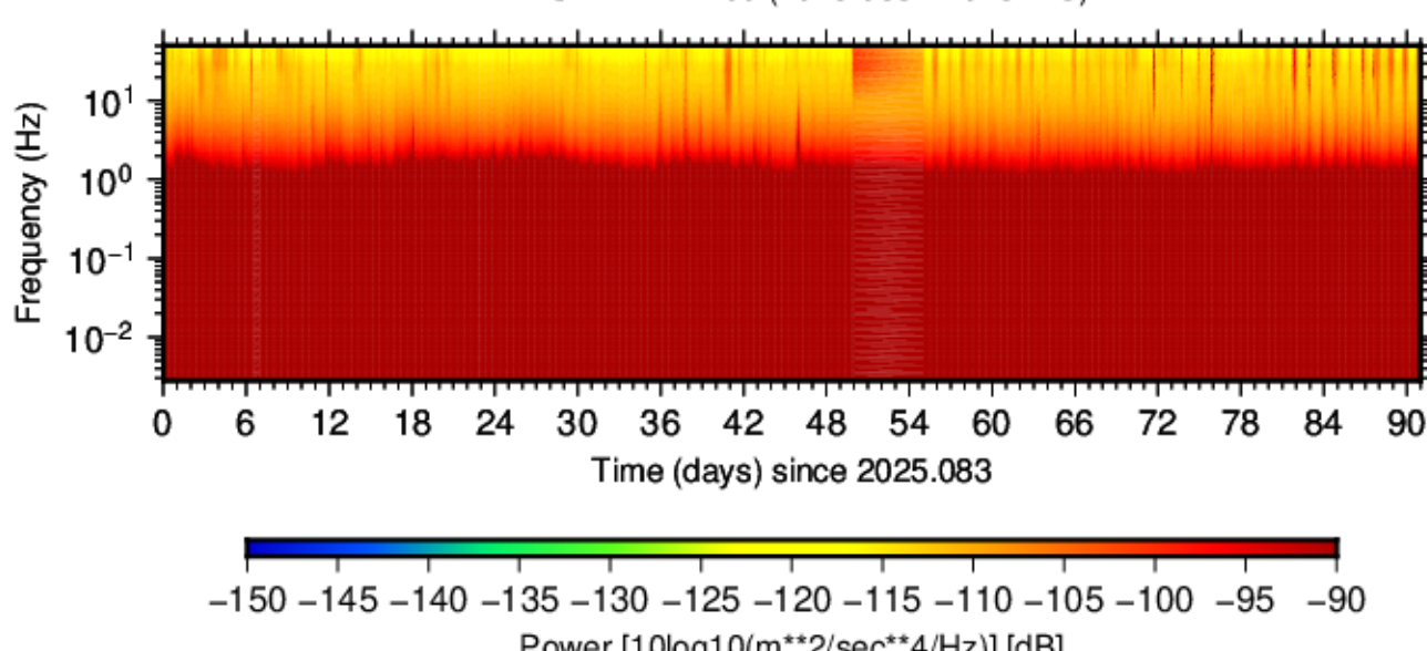
BK.SPAN.HNE.00 (2025.083 - 2025.173)
