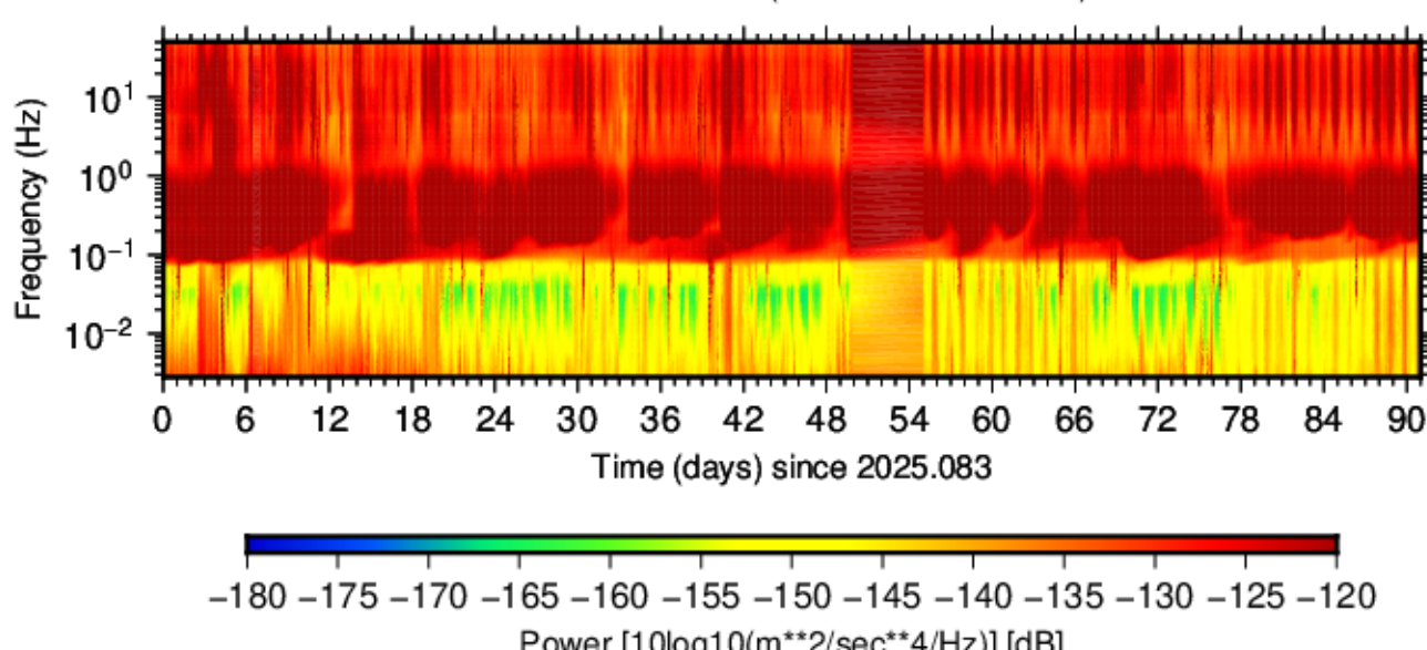
BK.SPAN.HHN.00 (2025.083 - 2025.173)
