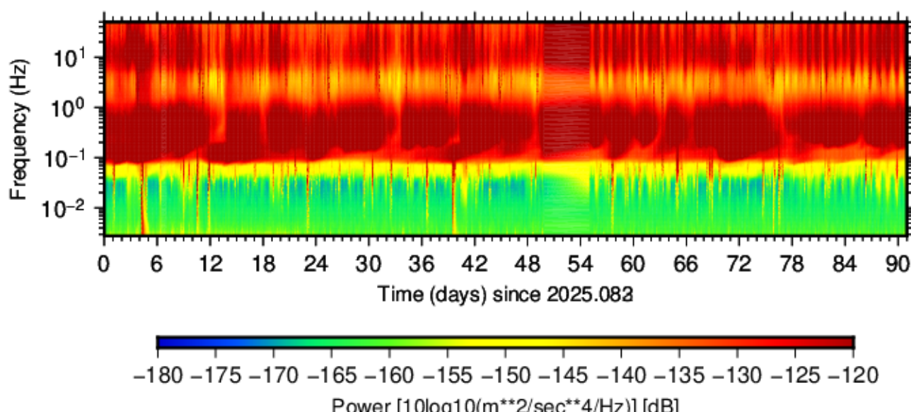
BK.SPAN.HHZ.00 (2025.083 - 2025.173)
