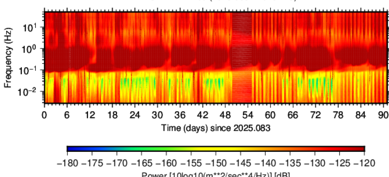
BK.SPAN.HHE.00 (2025.083 - 2025.173)
