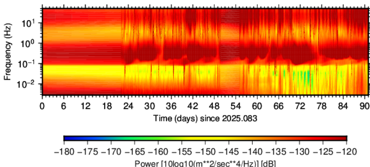
BK.SKGS.HHN.00 (2025.083 - 2025.173)
