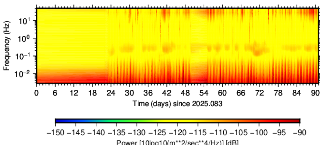
BK.SKGS.HNE.00 (2025.083 - 2025.173)
