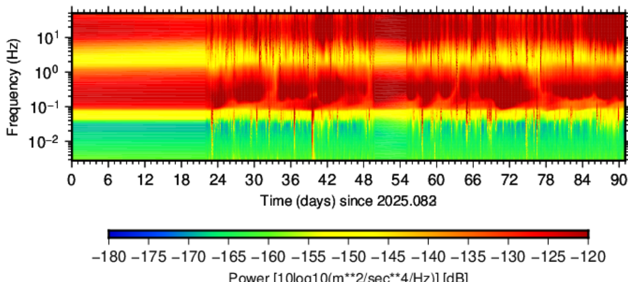
BK.SKGS.HHZ.00 (2025.083 - 2025.173)
