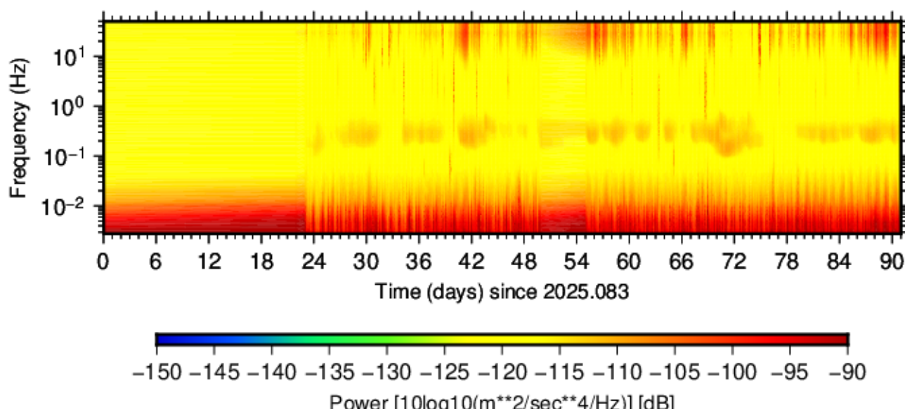
BK.SKGS.HNN.00 (2025.083 - 2025.173)
