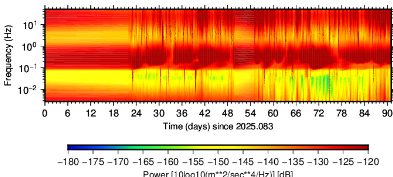
BK.SKGS.HHE.00 (2025.083 - 2025.173)
