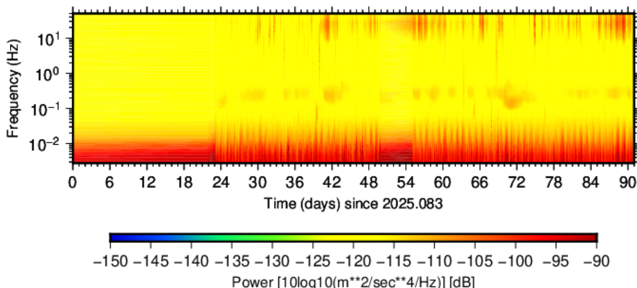
BK.SKGS.HNZ.00 (2025.083 - 2025.173)
