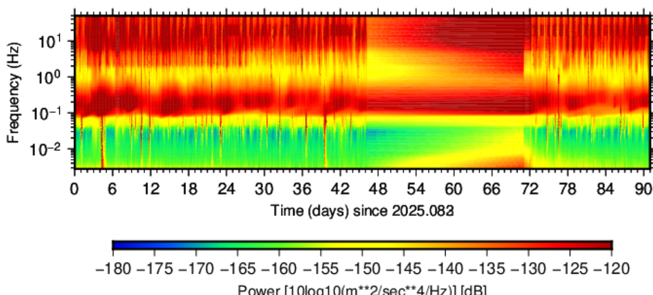
BK.SHEP.HHZ.01 (2025.083 - 2025.173)
