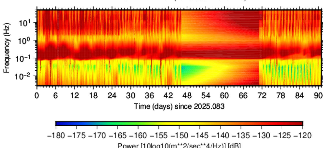
BK.SHEP.HHE.01 (2025.083 - 2025.173)
