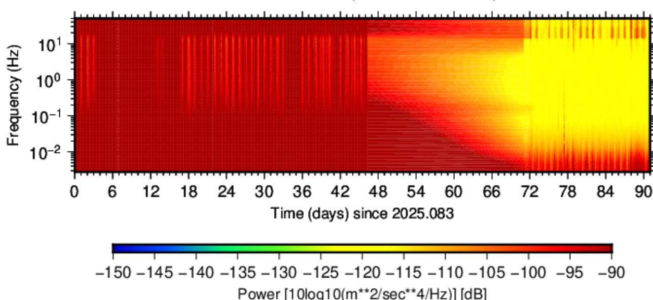
BK.SHEP.HNZ.01 (2025.083 - 2025.173)
