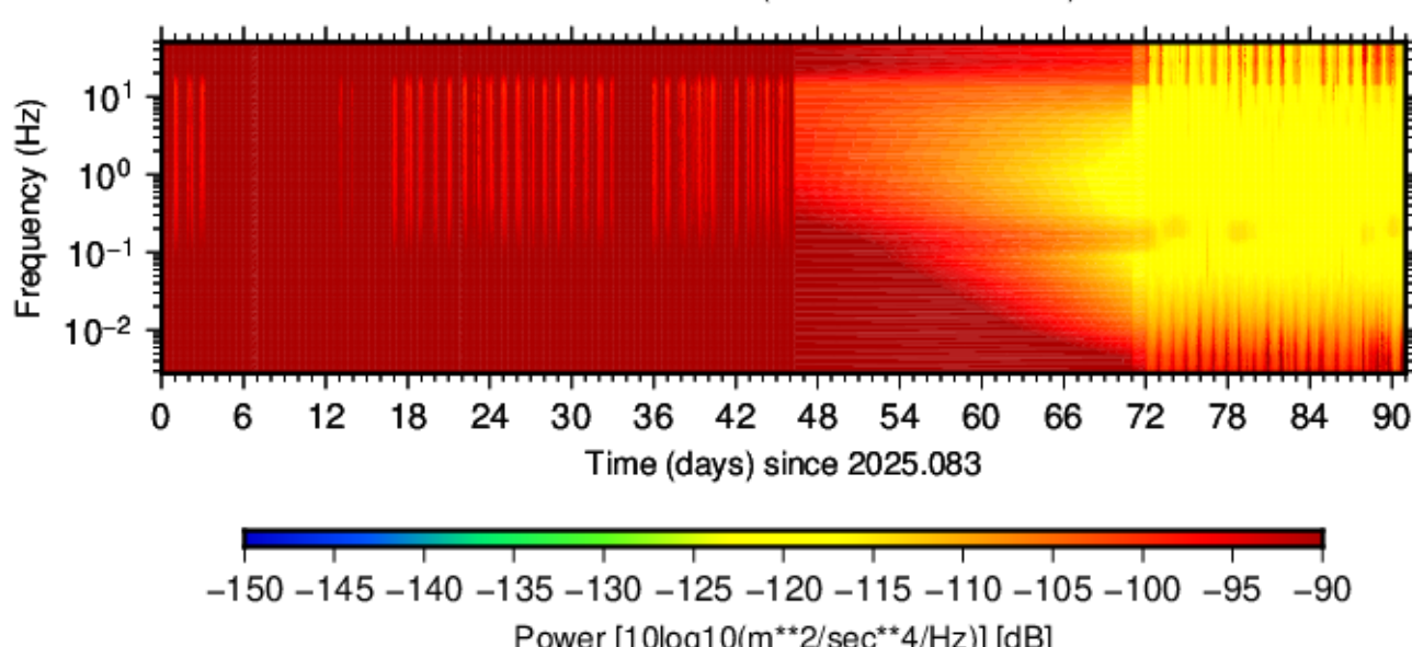
BK.SHEP.HNN.01 (2025.083 - 2025.173)
