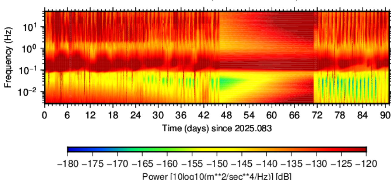
BK.SHEP.HHN.01 (2025.083 - 2025.173)
