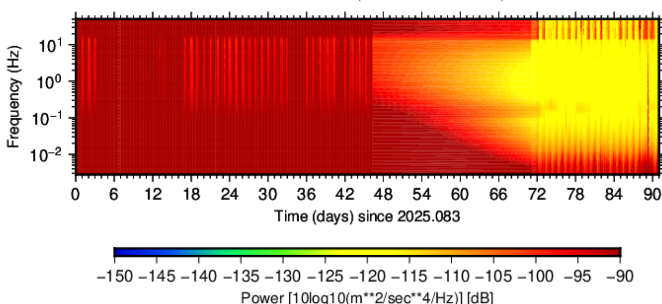
BK.SHEP.HNE.01 (2025.083 - 2025.173)
