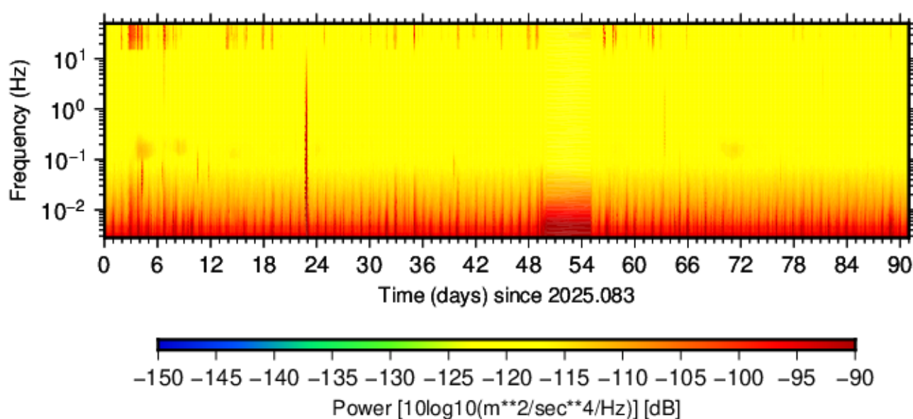
BK.SCOT.HNE.01 (2025.083 - 2025.173)
