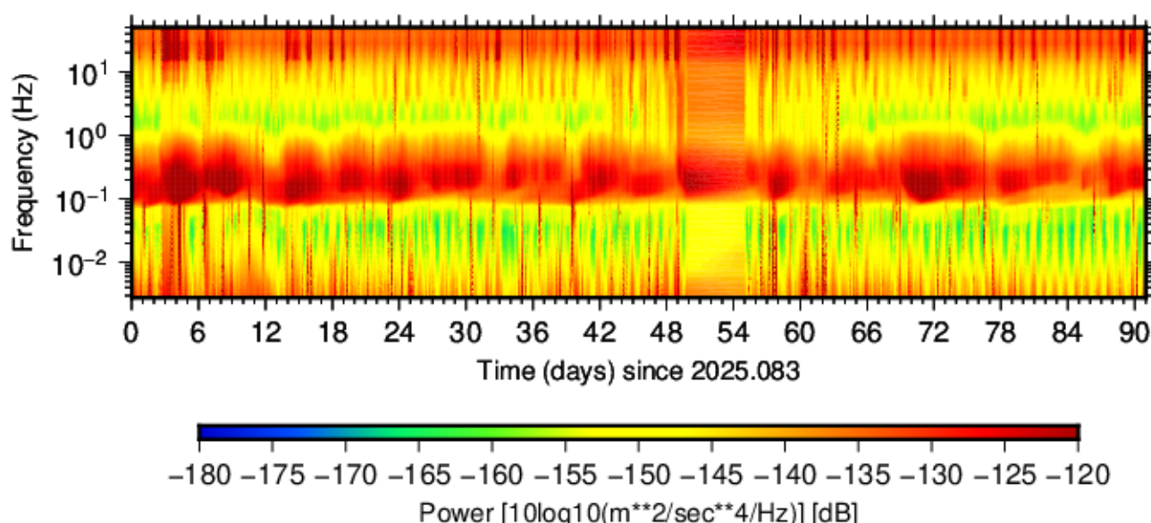
BK.SCOT.HHE.01 (2025.083 - 2025.173)
