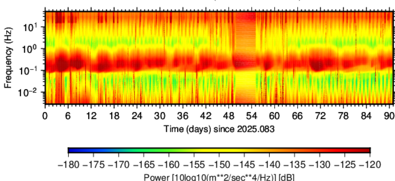
BK.SCOT.HHN.01 (2025.083 - 2025.173)
