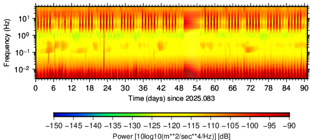
BK.SCCB.HNE.00 (2025.083 - 2025.173)
