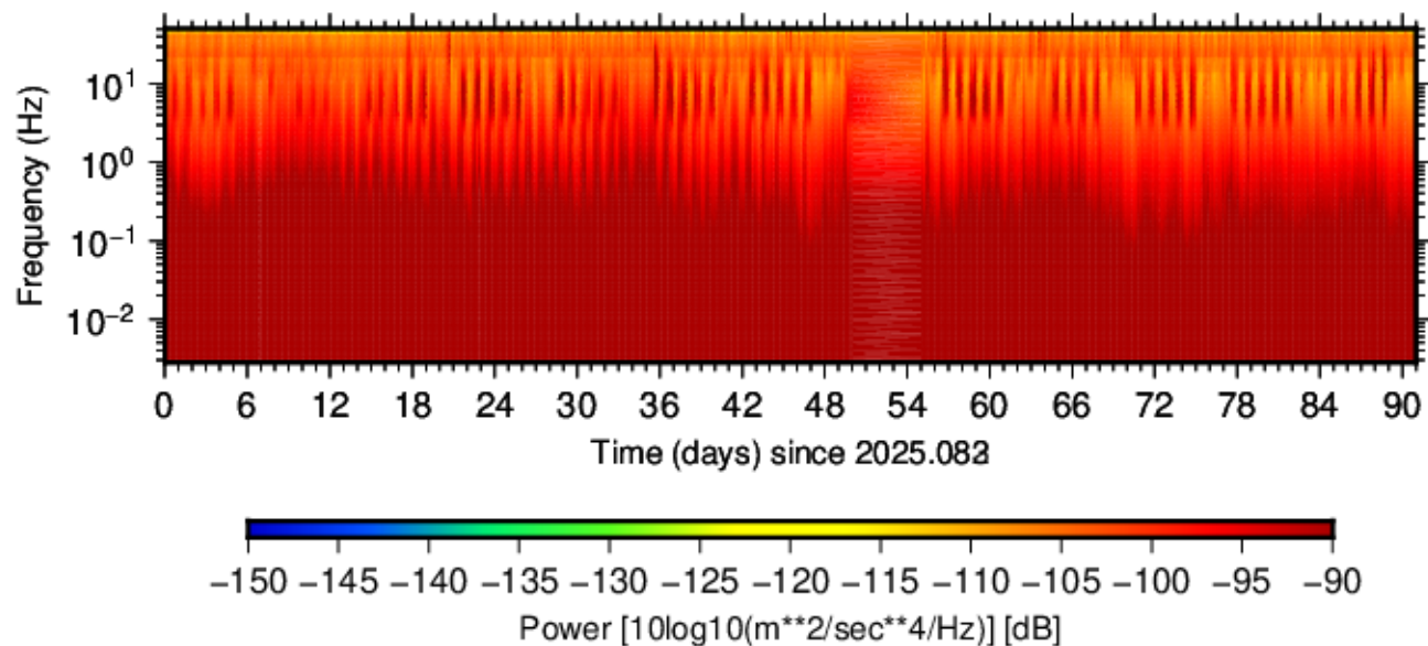
BK.SCCB.HNZ.00 (2025.083 - 2025.173)
