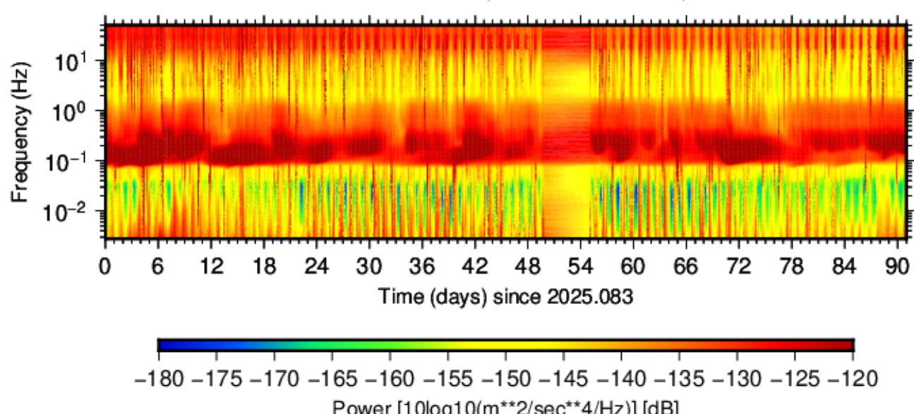
BK.SAO.HHE.00 (2025.083 - 2025.173)
