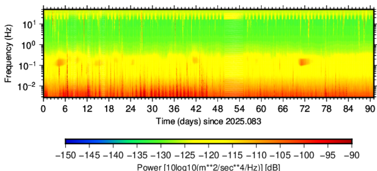
BK.SAO.HNZ.00 (2025.083 - 2025.173)
