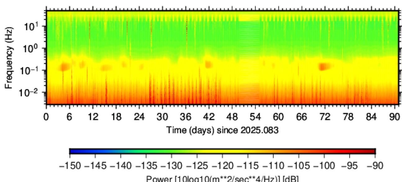
BK.SAO.HNN.00 (2025.083 - 2025.173)
