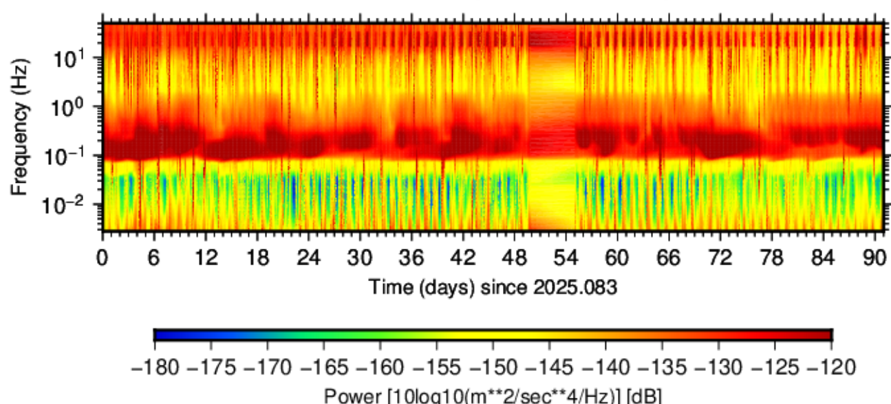
BK.SAO.HHN.00 (2025.083 - 2025.173)
