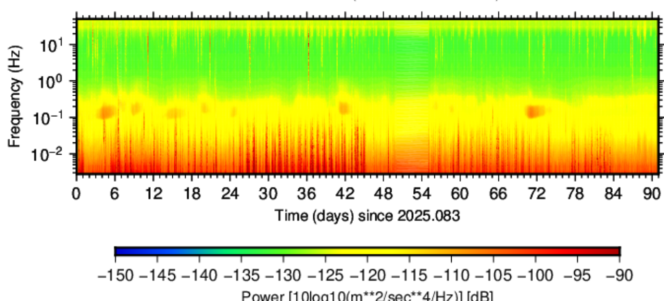
BK.SAO.HNE.00 (2025.083 - 2025.173)
