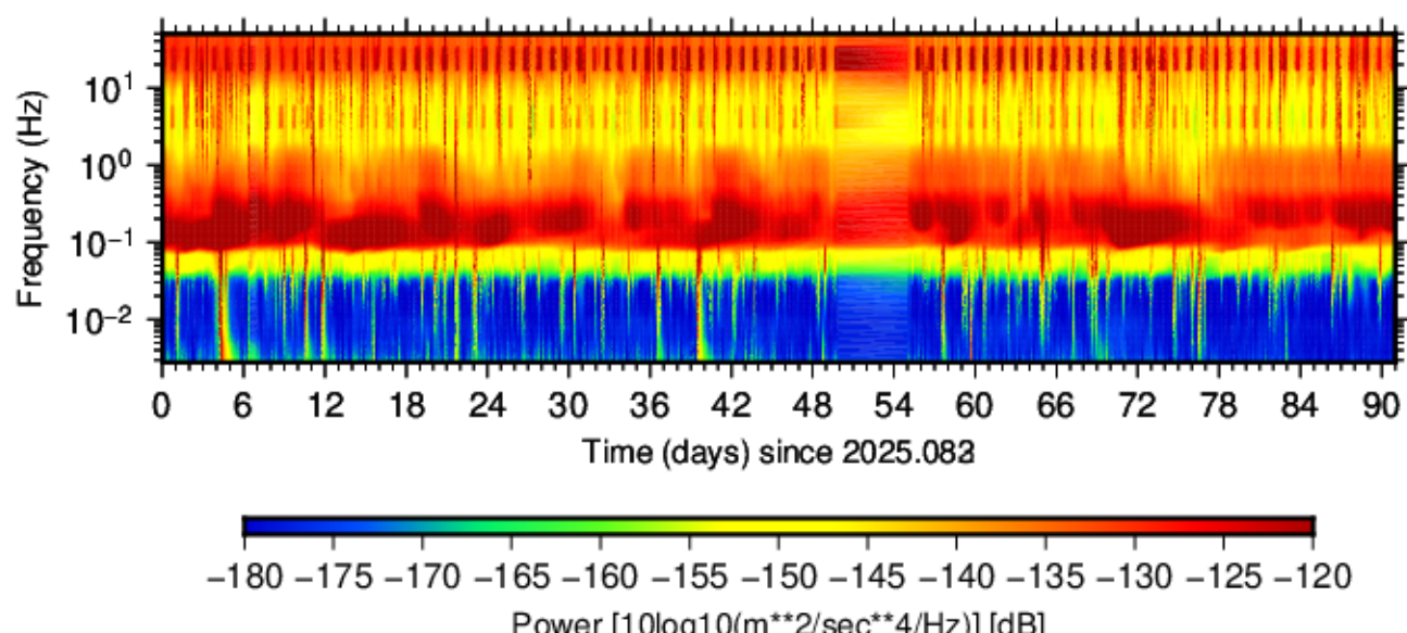
BK.SAO.HHZ.00 (2025.083 - 2025.173)
