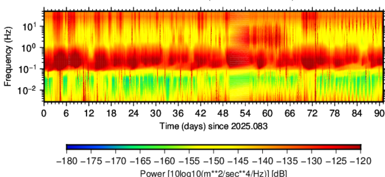
BK.SANG.HHN.00 (2025.083 - 2025.173)
