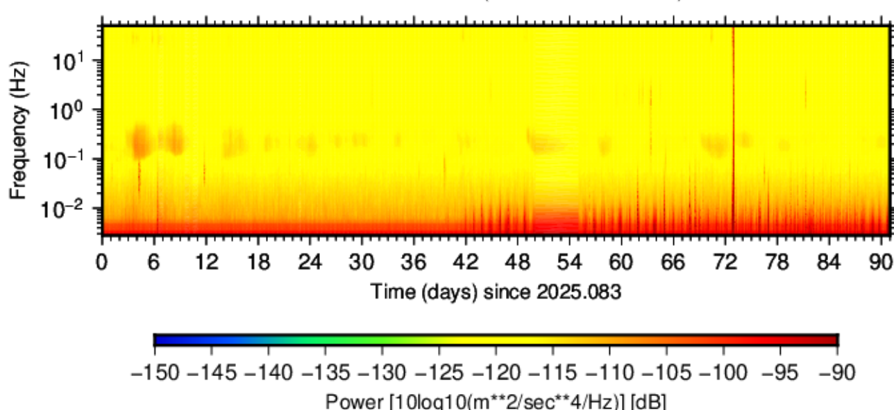
BK.SANG.HNE.00 (2025.083 - 2025.173)
