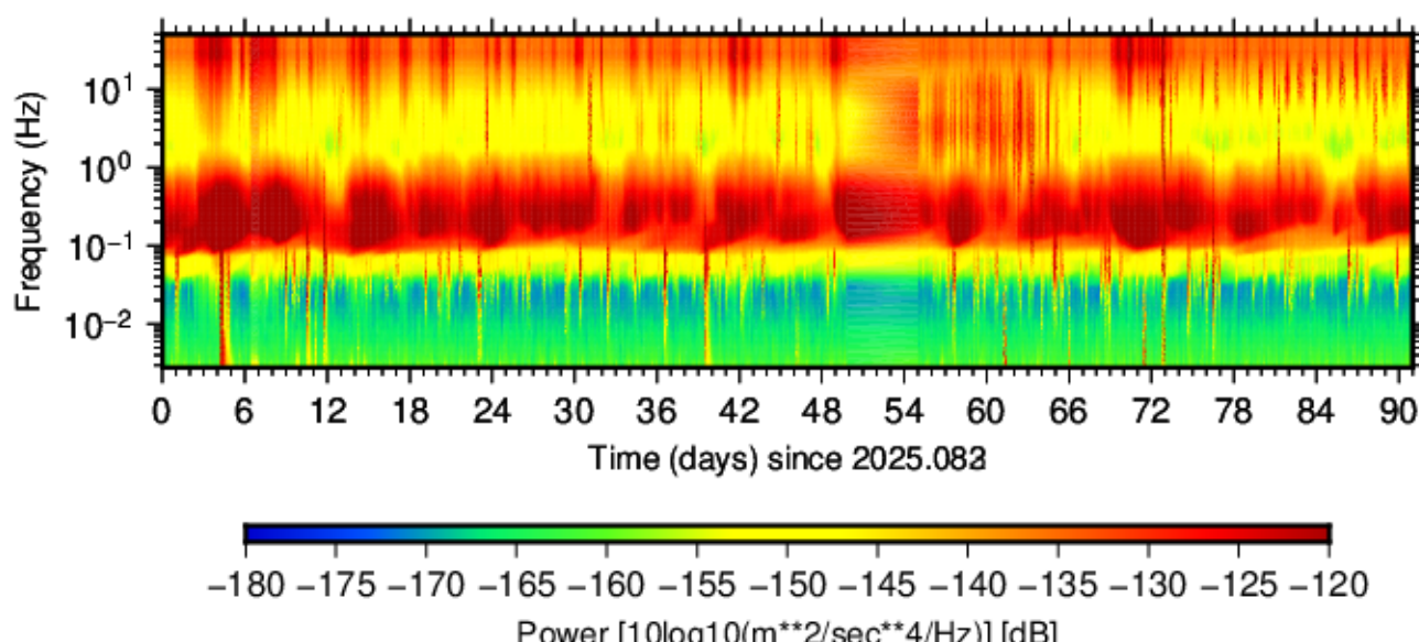
BK.SANG.HHZ.00 (2025.083 - 2025.173)
