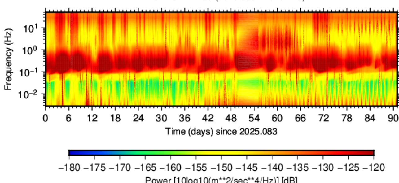
BK.SANG.HHE.00 (2025.083 - 2025.173)
