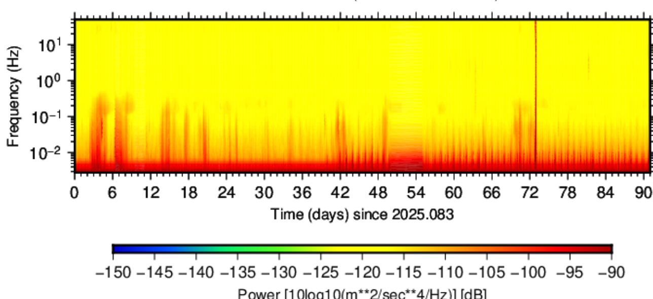
BK.SANG.HNN.00 (2025.083 - 2025.173)
