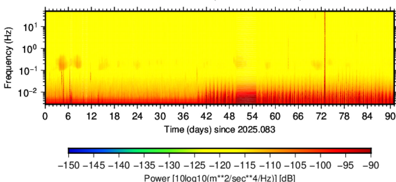
BK.SANG.HNZ.00 (2025.083 - 2025.173)
