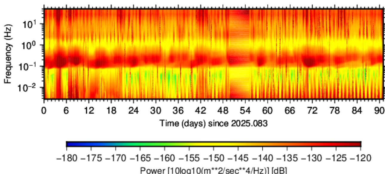
BK.SAGE.HHN.00 (2025.083 - 2025.173)
