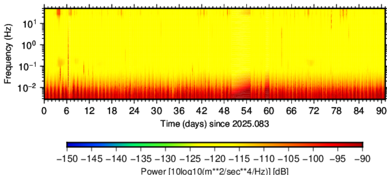
BK.SAGE.HNE.00 (2025.083 - 2025.173)
