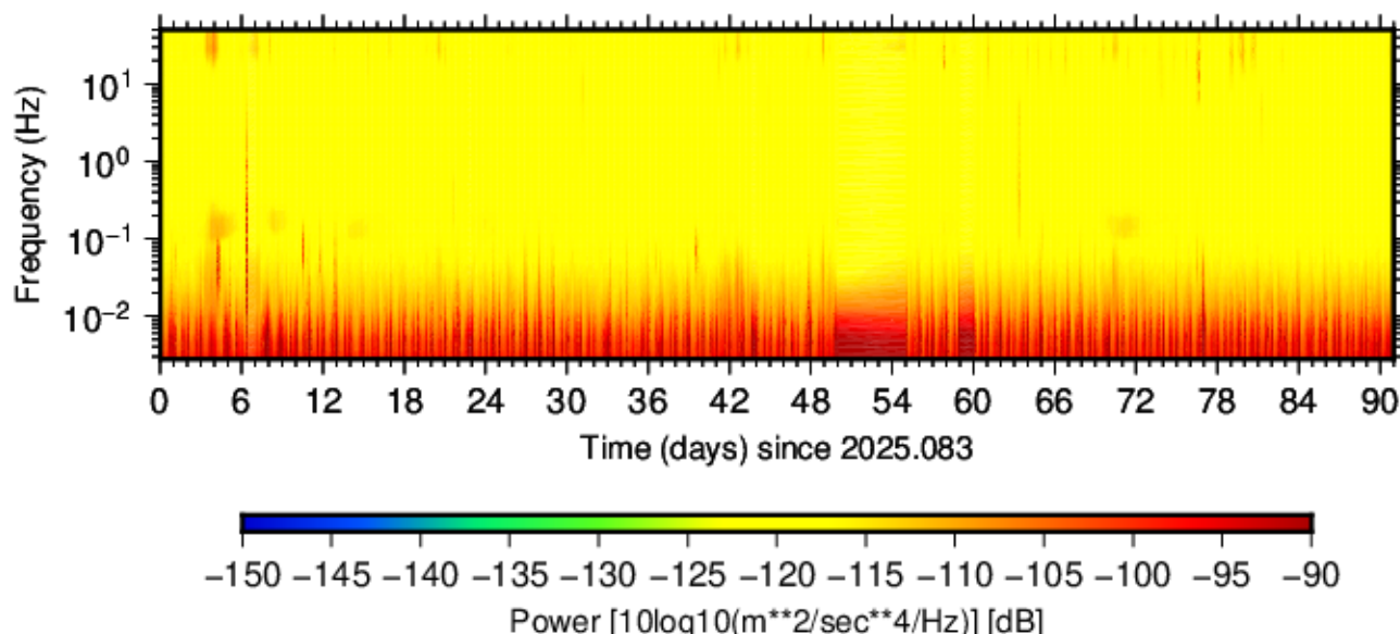
BK.SAGE.HNZ.00 (2025.083 - 2025.173)
