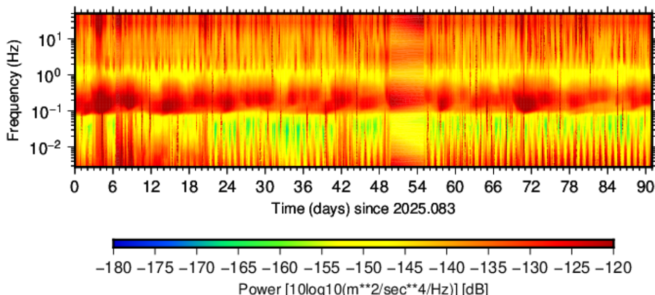
BK.SAGE.HHE.00 (2025.083 - 2025.173)
