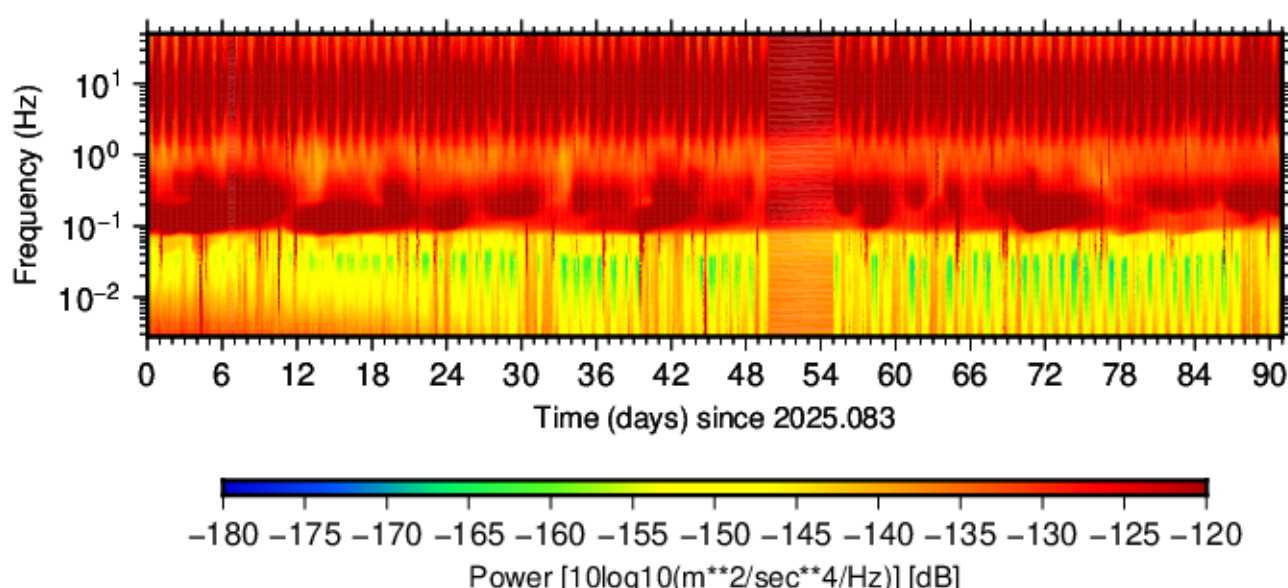
BK.RVRP.HHN.00 (2025.083 - 2025.173)
