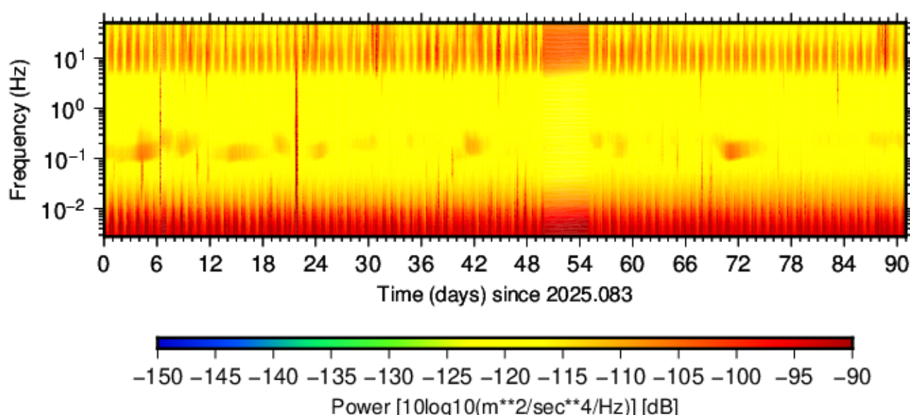
BK.RVRP.HNZ.00 (2025.083 - 2025.173)
