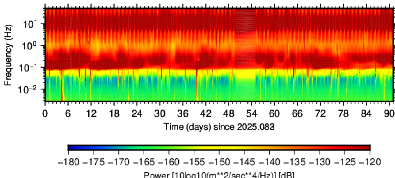
BK.RVRP.HHZ.00 (2025.083 - 2025.173)
