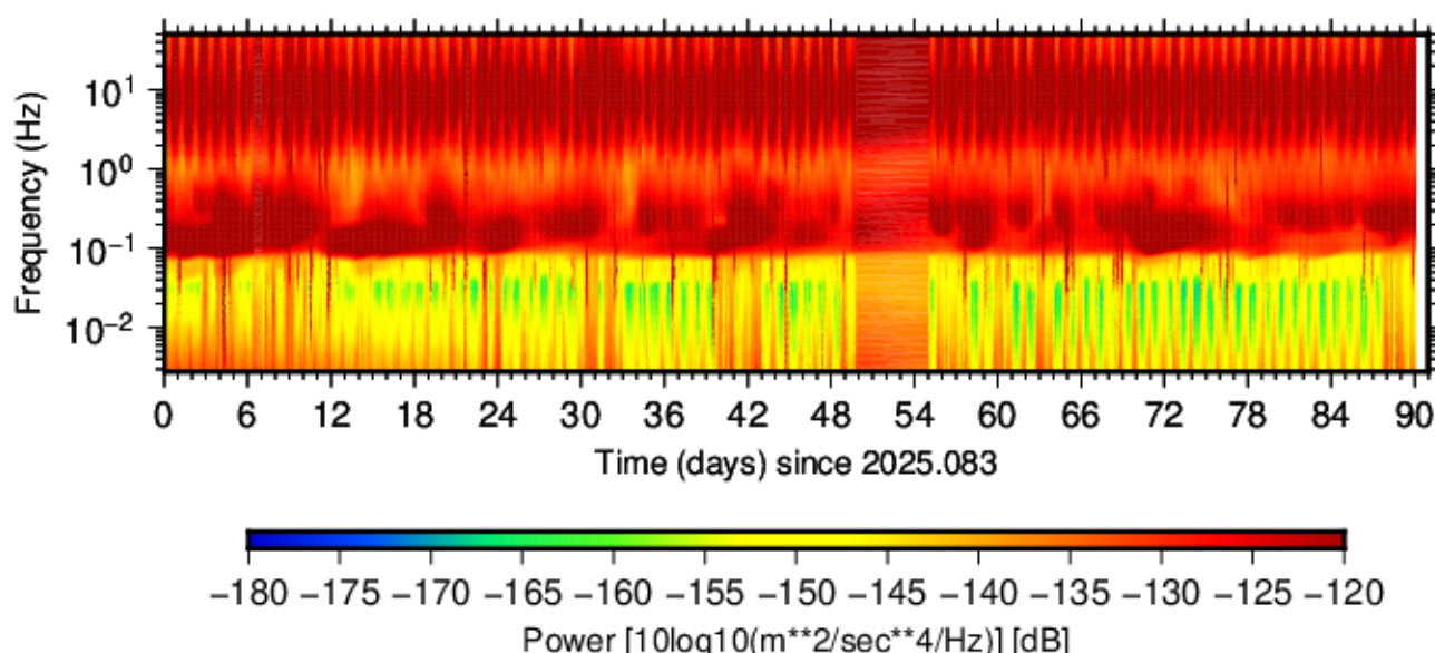
BK.RVRP.HHE.00 (2025.083 - 2025.173)
