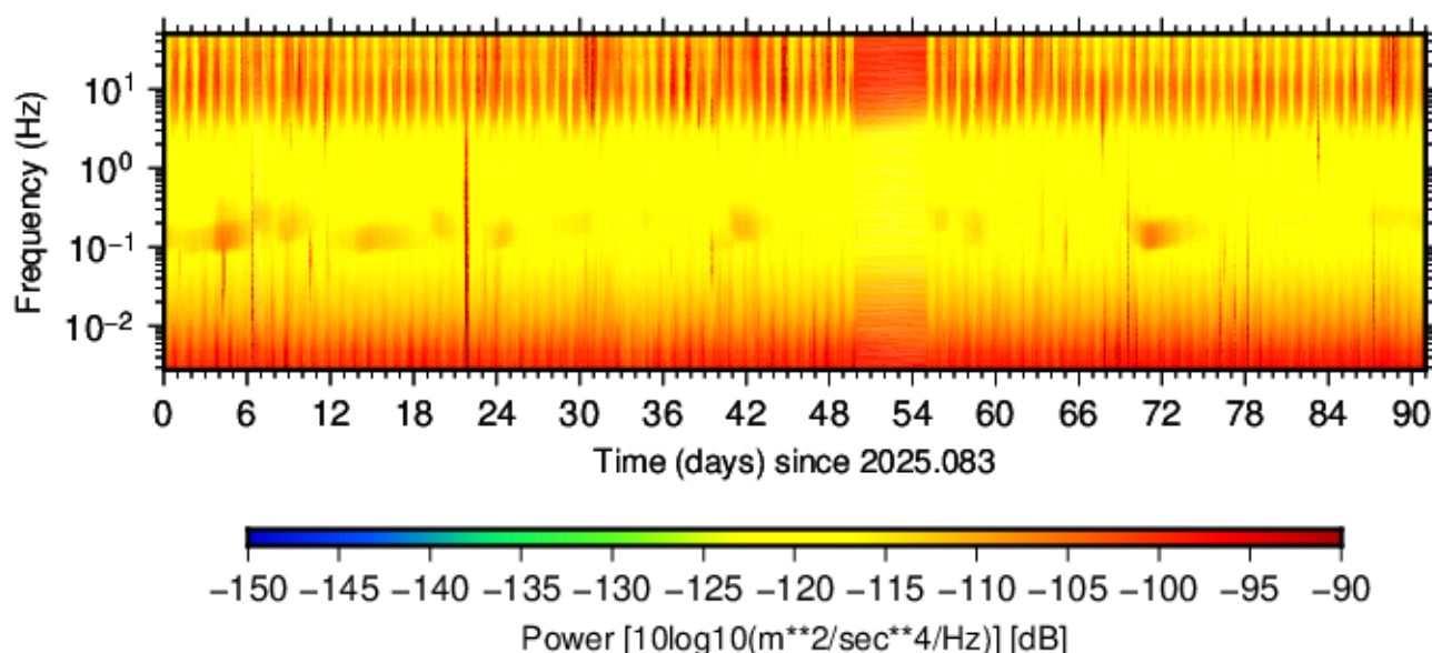
BK.RVRP.HNN.00 (2025.083 - 2025.173)
