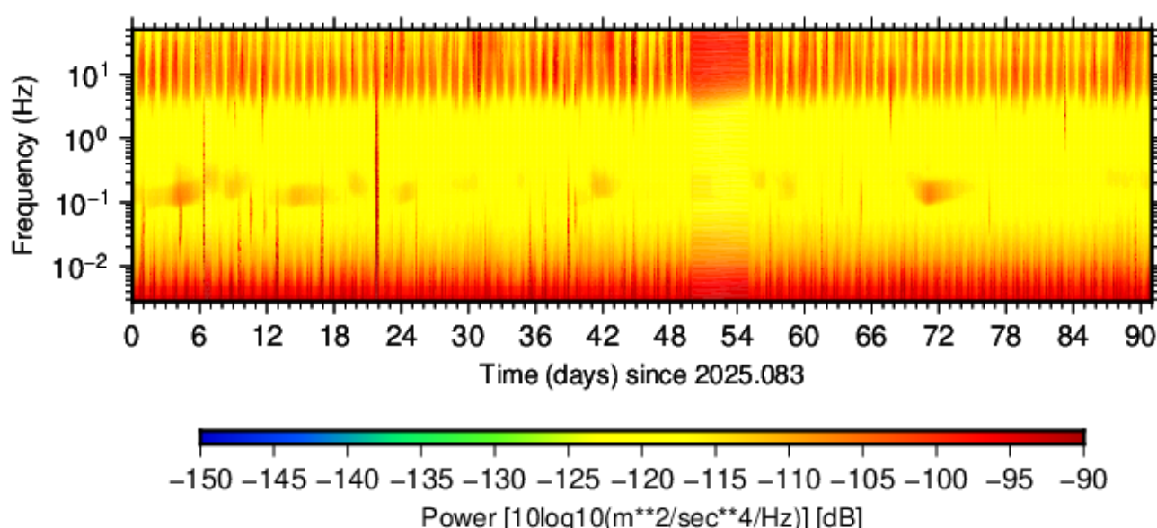
BK.RVRP.HNE.00 (2025.083 - 2025.173)
