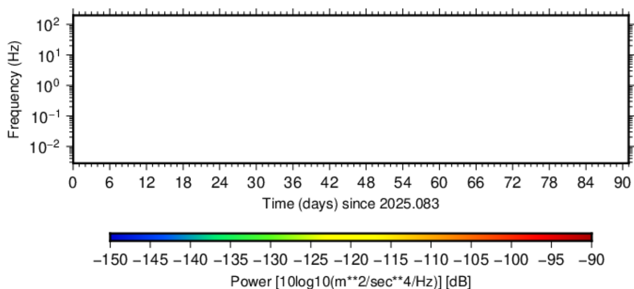
BG.RTB.DPE. (2025.083 - 2025.173)
