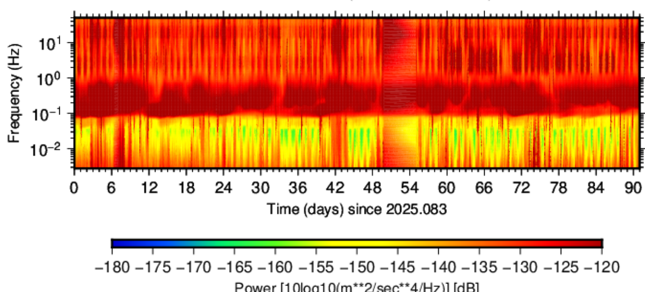
BK.ROMB.HHE.00 (2025.083 - 2025.173)
