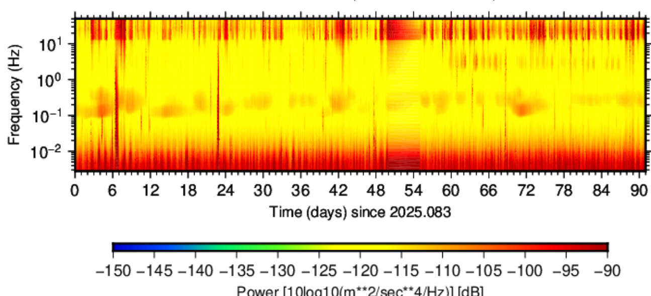
BK.ROMB.HNE.00 (2025.083 - 2025.173)
