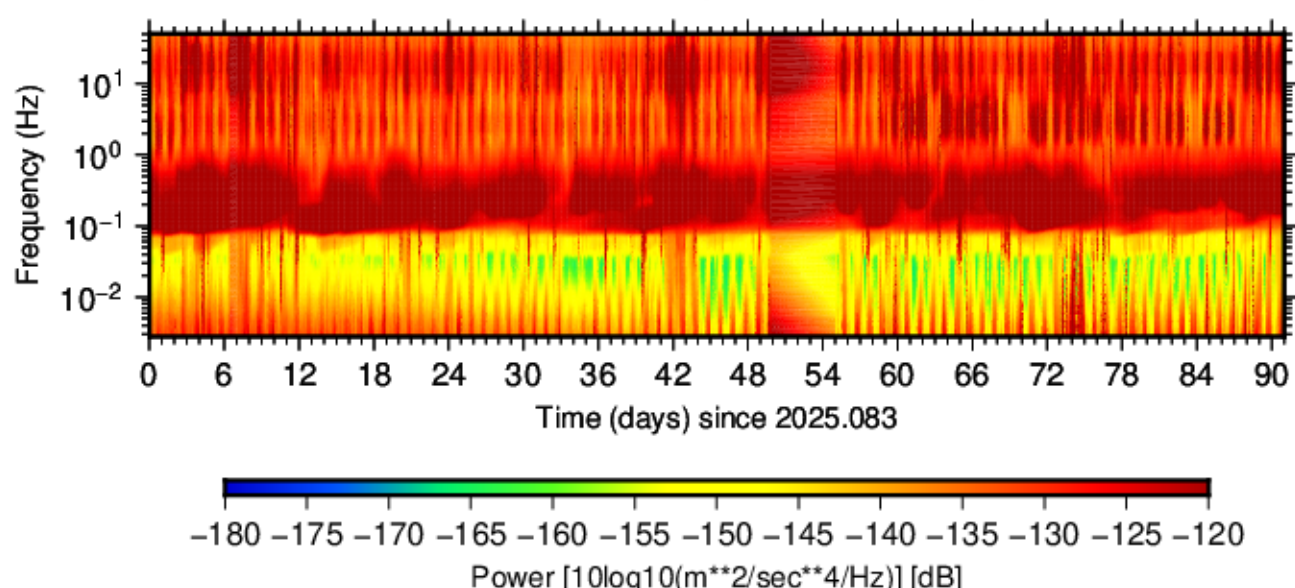
BK.ROMB.HHN.00 (2025.083 - 2025.173)
