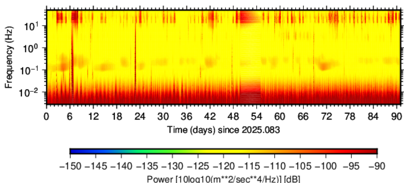
BK.ROMB.HNZ.00 (2025.083 - 2025.173)
