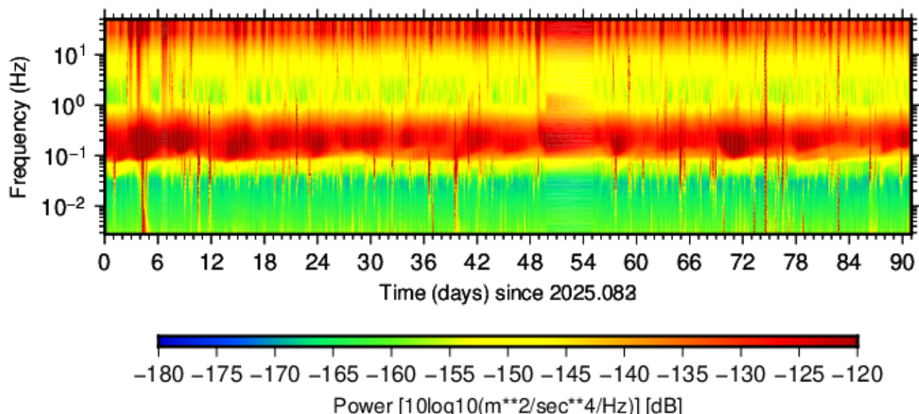
BK.RIMR.HHZ.00 (2025.083 - 2025.173)
