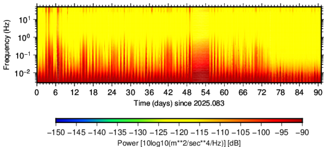
BK.RIMR.HNZ.00 (2025.083 - 2025.173)
