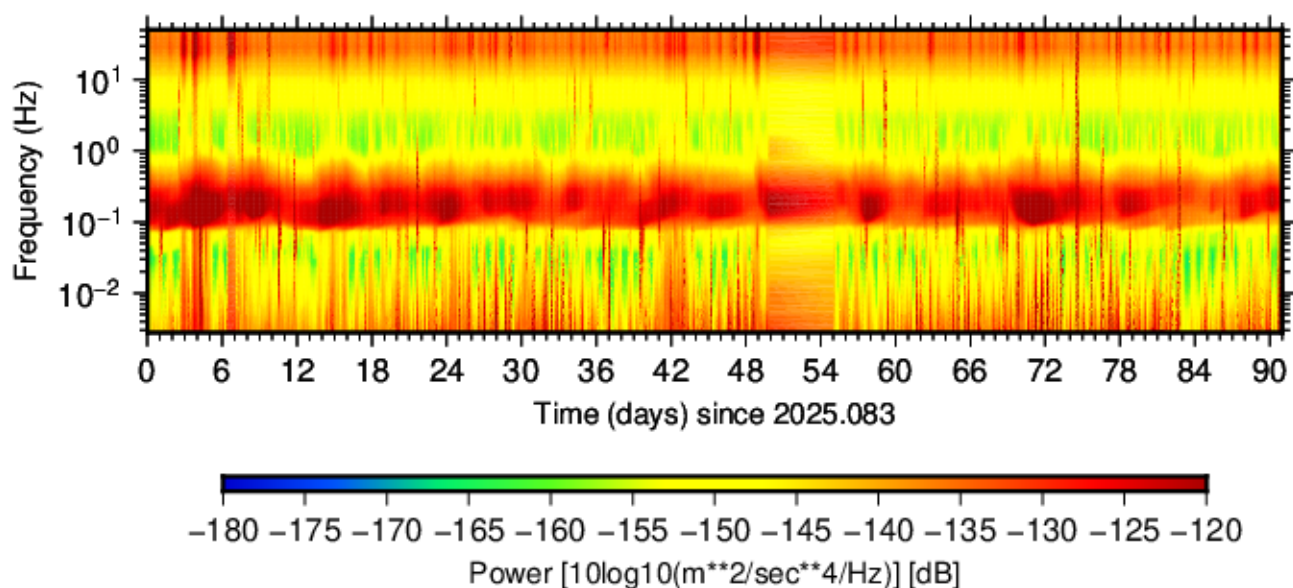
BK.RIMR.HHN.00 (2025.083 - 2025.173)
