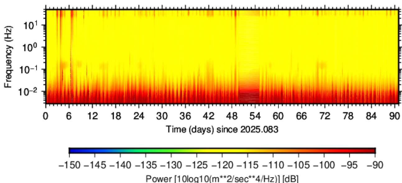
BK.RIMR.HNN.00 (2025.083 - 2025.173)
