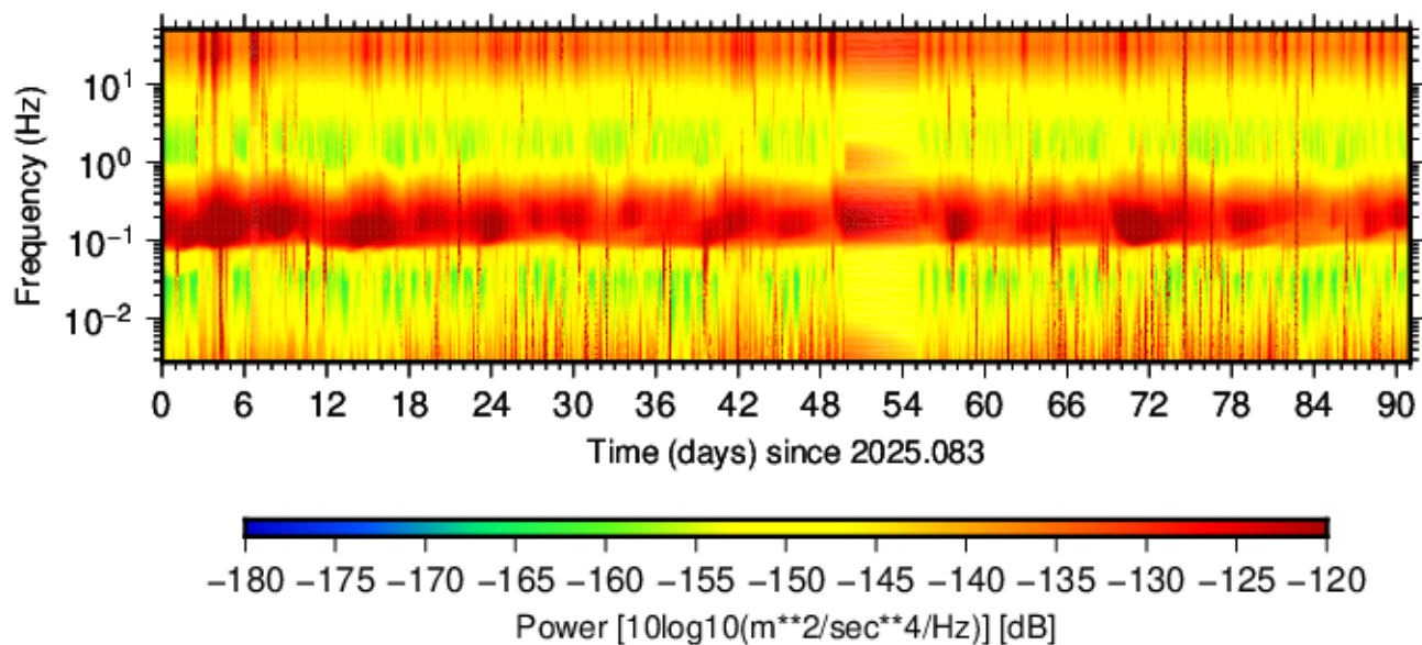
BK.RIMR.HHE.00 (2025.083 - 2025.173)
