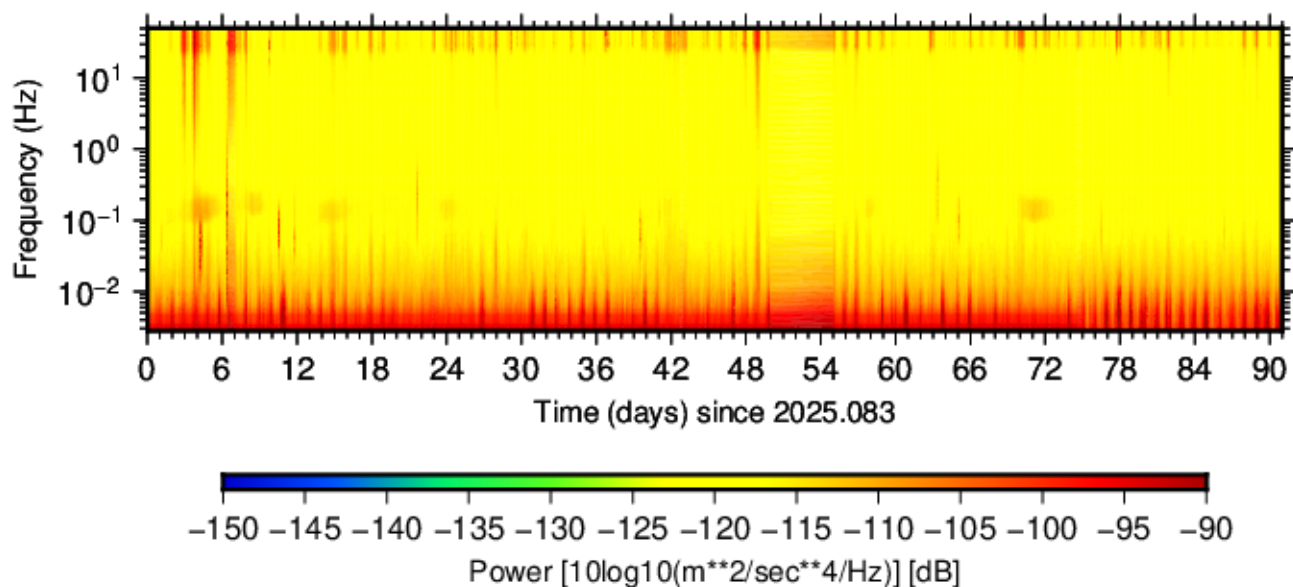
BK.RIMR.HNE.00 (2025.083 - 2025.173)
