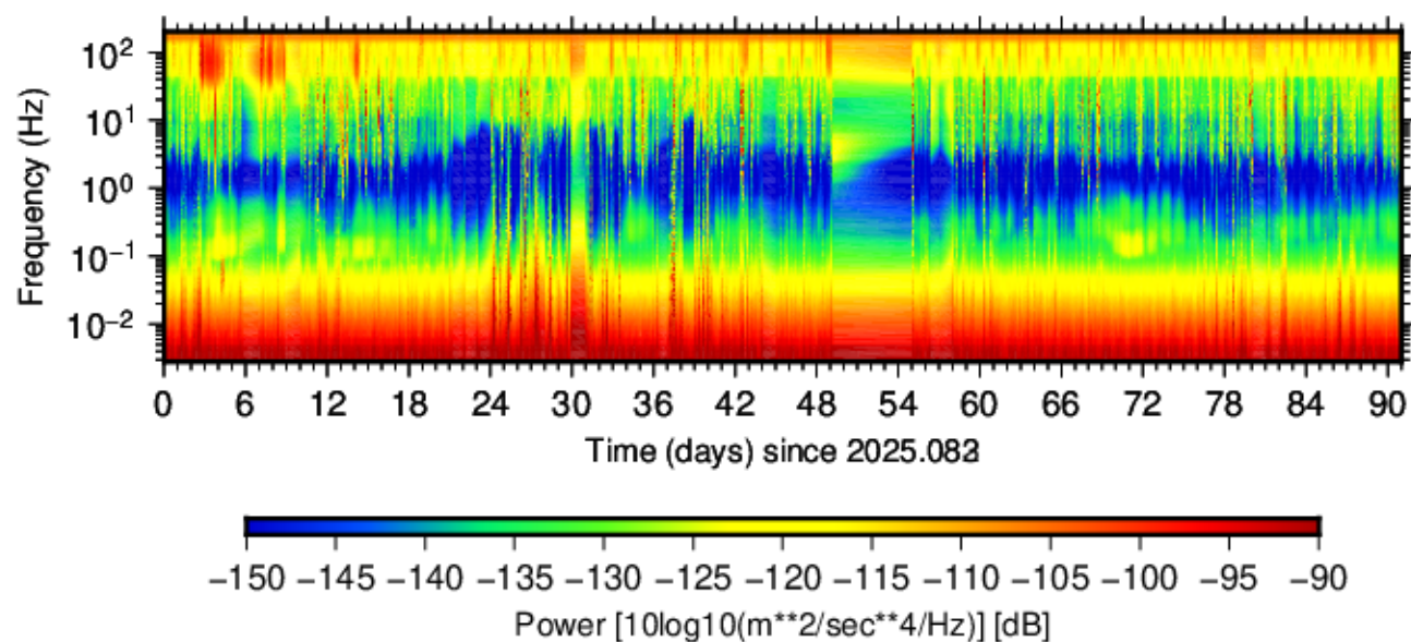
BG.RGP.DPZ. (2025.083 - 2025.173)
