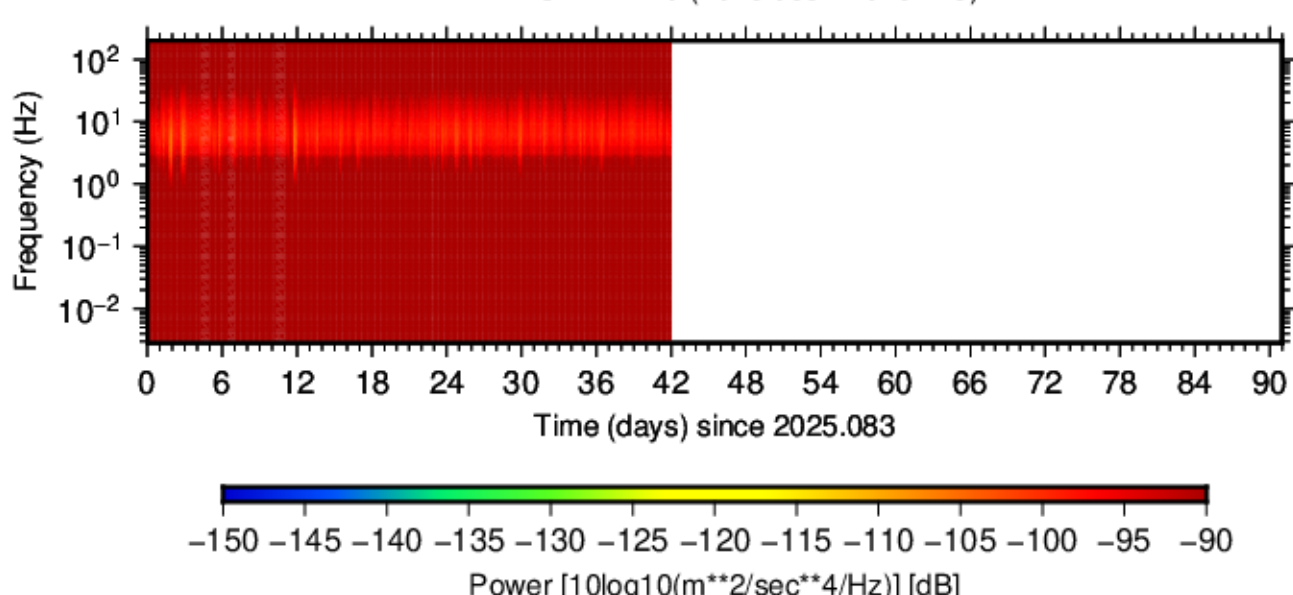
BK.RFSB.DP1.40 (2025.083 - 2025.173)
