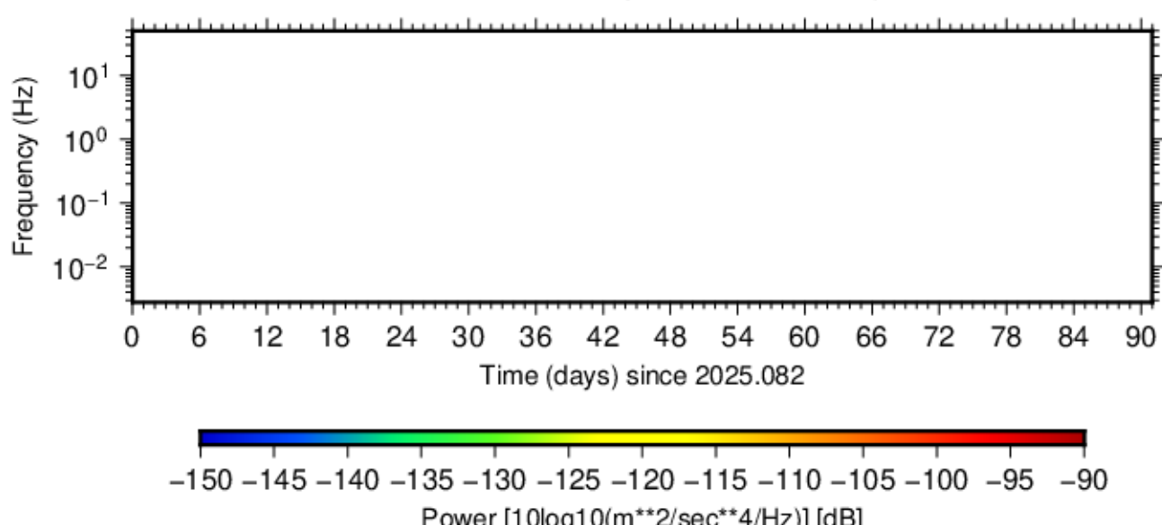
BK.RFSB.HNZ.00 (2025.083 - 2025.173)
