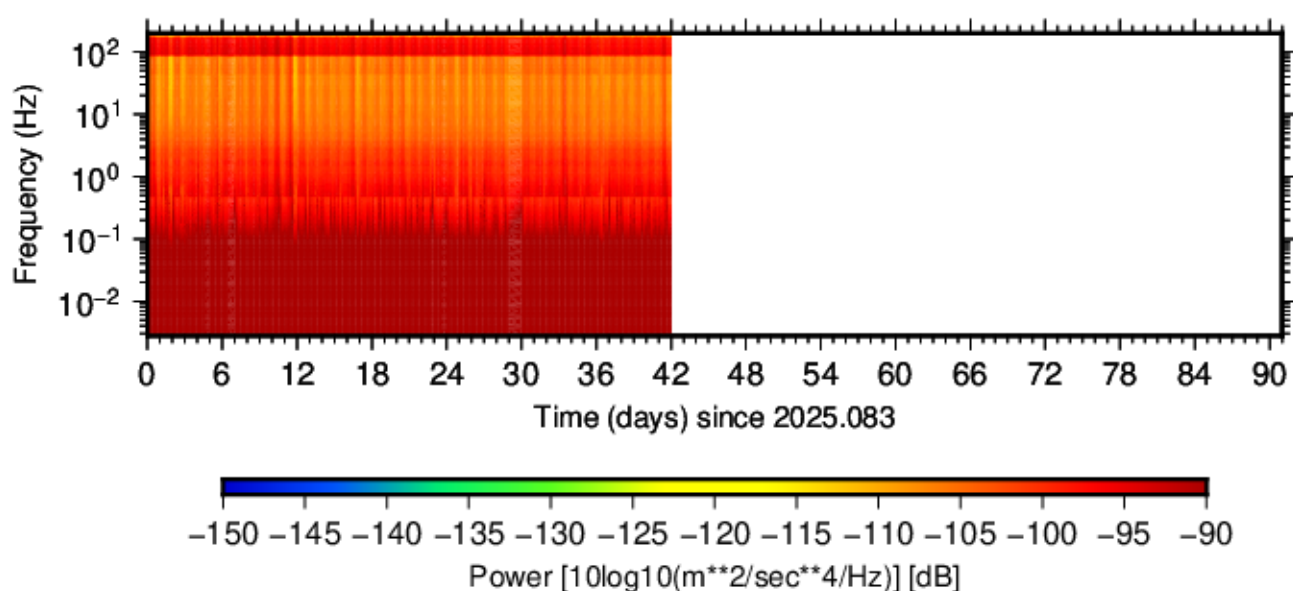
BK.RFSB.CN3.40 (2025.083 - 2025.173)
