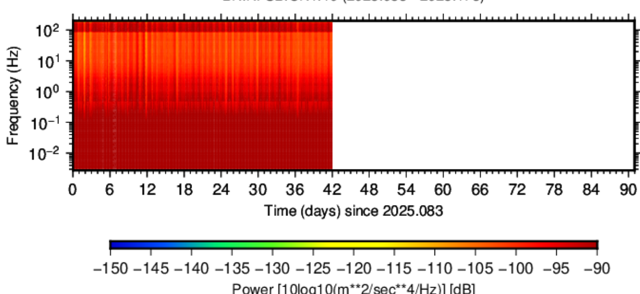
BK.RFSB.CN1.40 (2025.083 - 2025.173)
