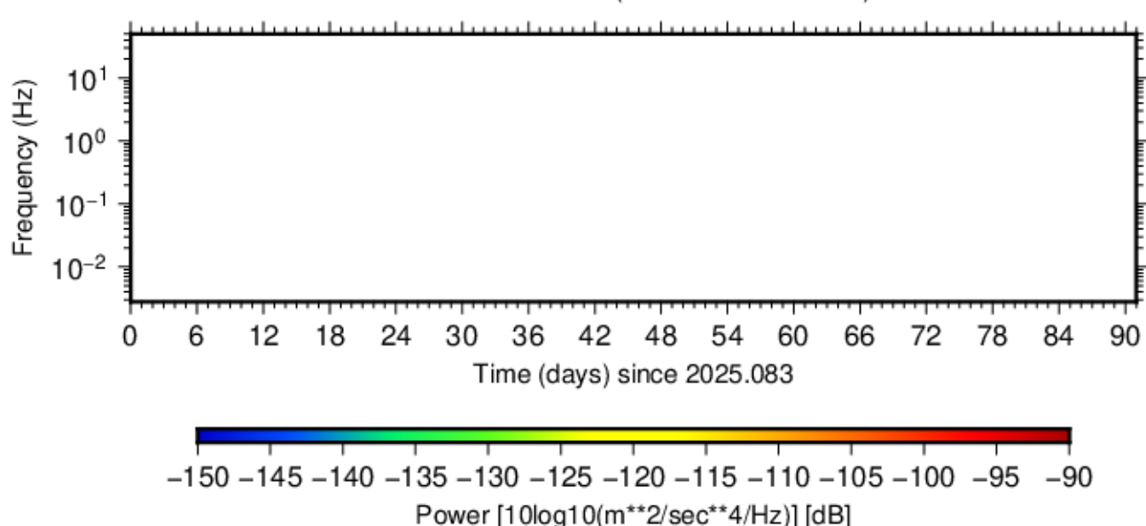
BK.RFSB.HNN.00 (2025.083 - 2025.173)
