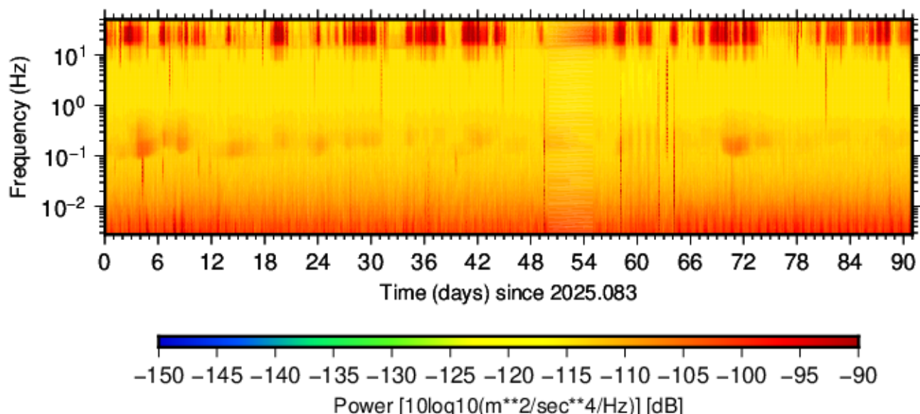
BK.RBOW.HNZ.00 (2025.083 - 2025.173)
