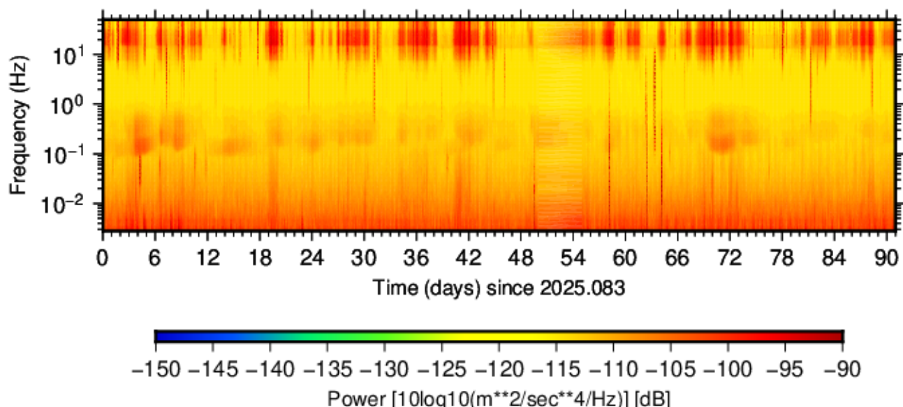
BK.RBOW.HNE.00 (2025.083 - 2025.173)
