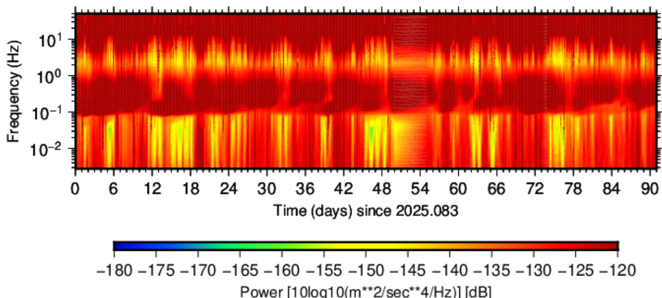
BK.RBOW.HHE.00 (2025.083 - 2025.173)
