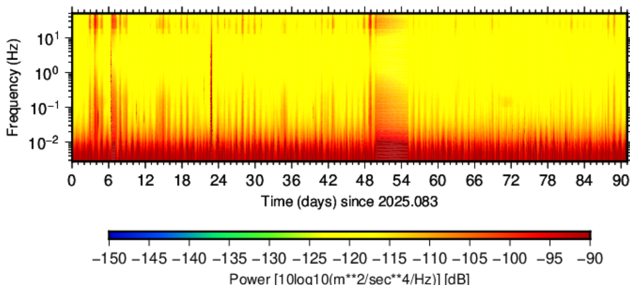
BK.RAVE.HNZ.00 (2025.083 - 2025.173)
