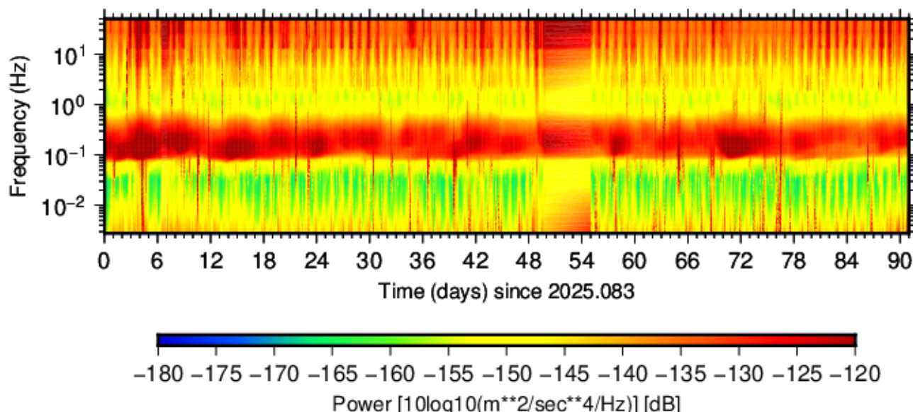
BK.RAVE.HHE.00 (2025.083 - 2025.173)
