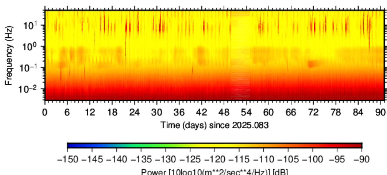
BK.RAMR.HNN.00 (2025.083 - 2025.173)
