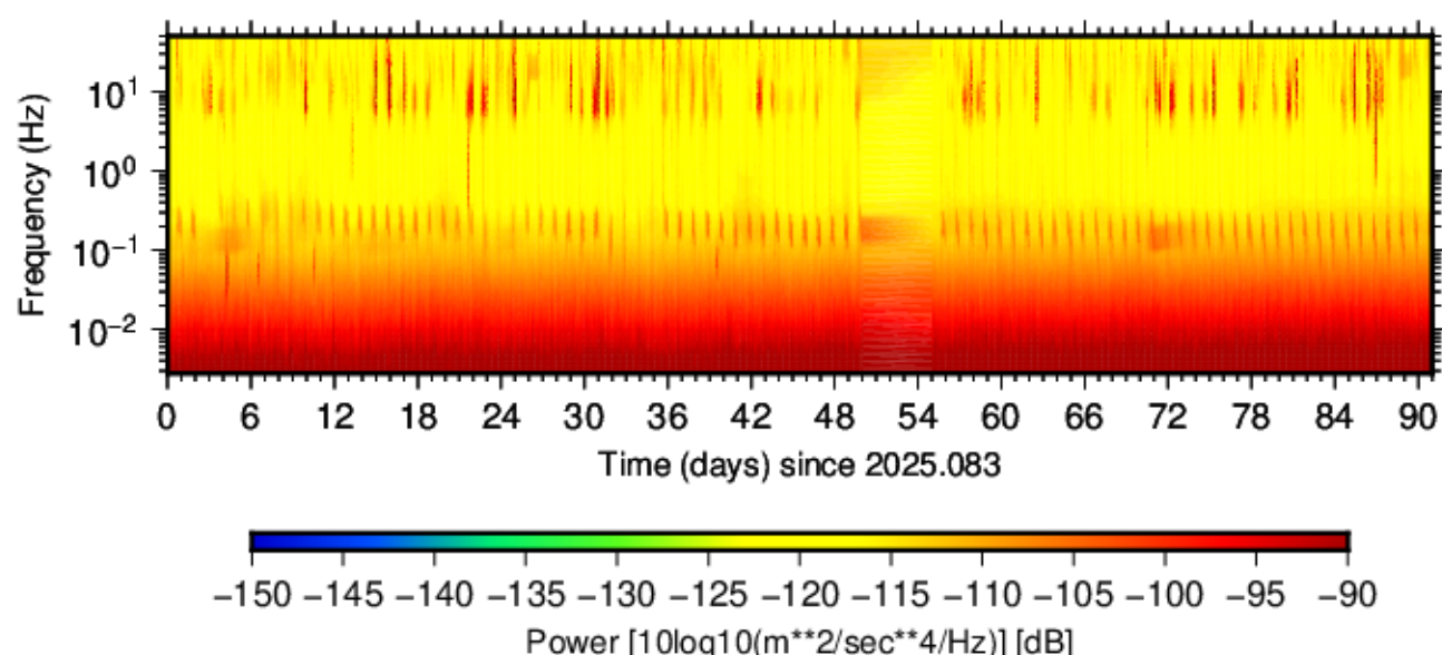
BK.RAMR.HNZ.00 (2025.083 - 2025.173)
