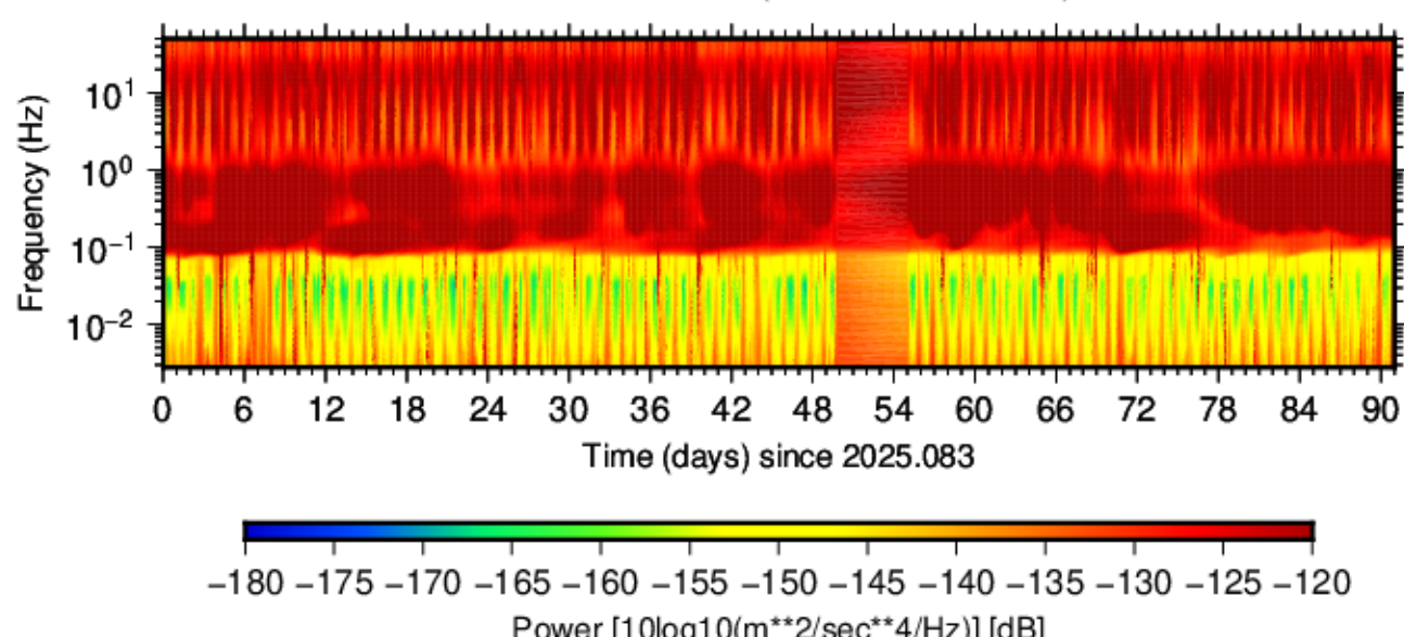
BK.RAMR.HHE.00 (2025.083 - 2025.173)
