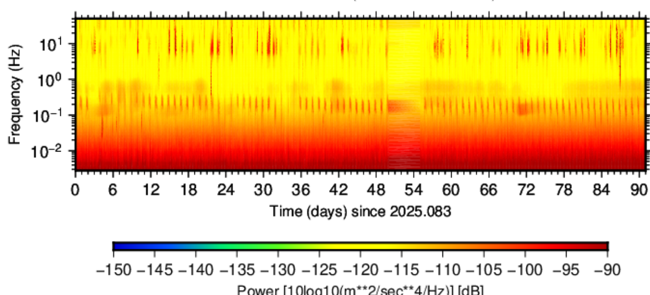
BK.RAMR.HNE.00 (2025.083 - 2025.173)
