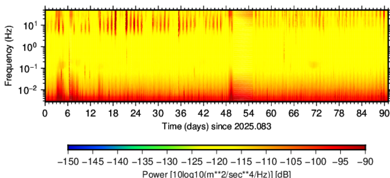
BK.PWAY.HNE.00 (2025.083 - 2025.173)
