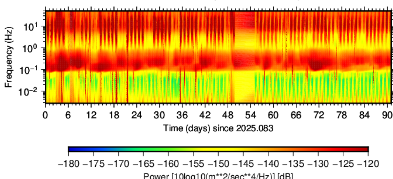
BK.PWAY.HHE.00 (2025.083 - 2025.173)
