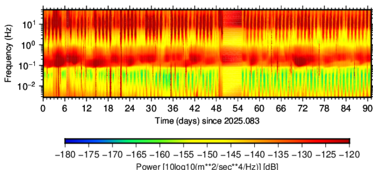
BK.PWAY.HHN.00 (2025.083 - 2025.173)
