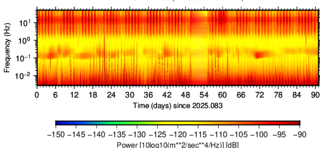
BK.PVSP.HNE.00 (2025.083 - 2025.173)
