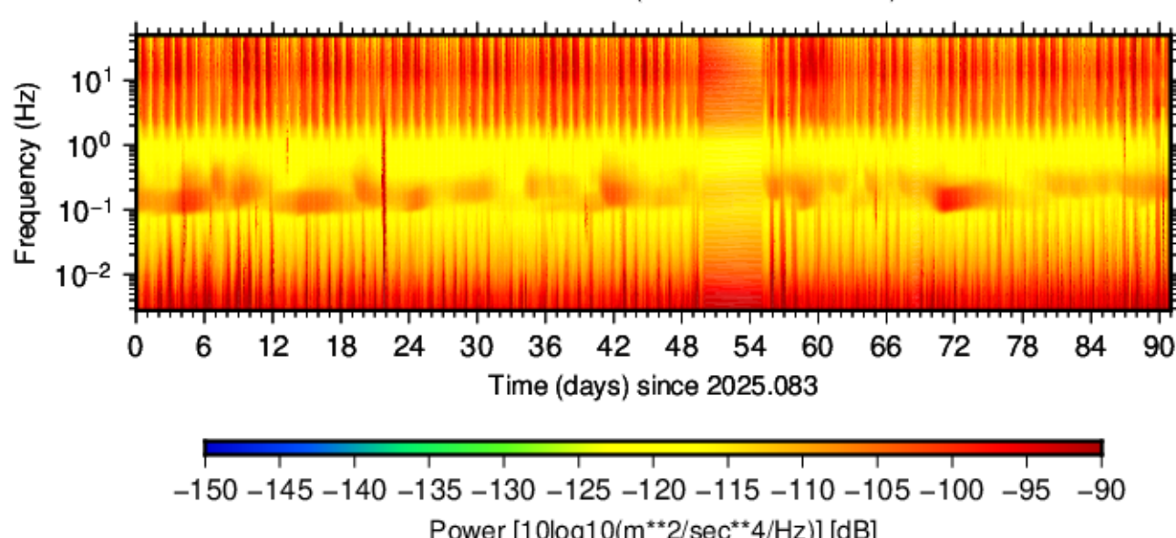
BK.PVSP.HNN.00 (2025.083 - 2025.173)
