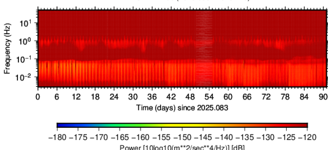
BK.PVSP.HHE.00 (2025.083 - 2025.173)
