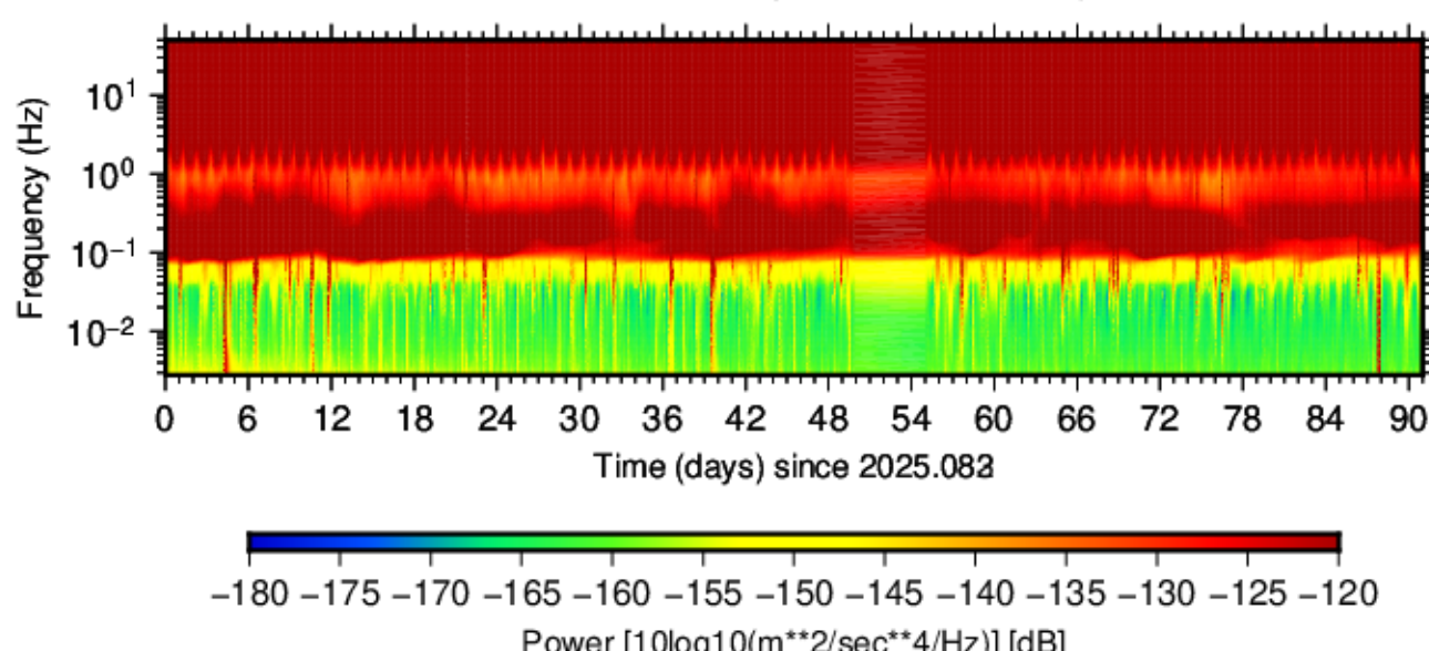
BK.PVSP.HHZ.00 (2025.083 - 2025.173)
