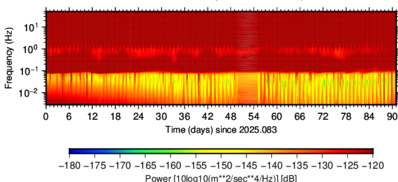
BK.PVSP.HHN.00 (2025.083 - 2025.173)
