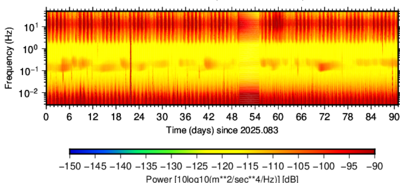
BK.PVSP.HNZ.00 (2025.083 - 2025.173)
