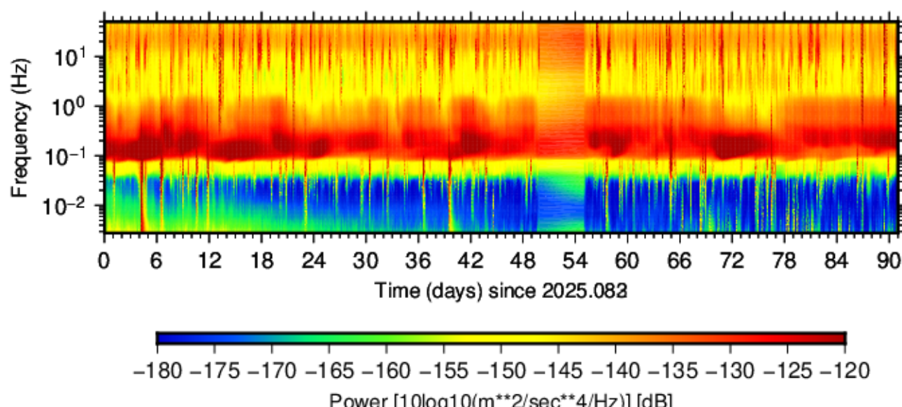
BK.PKD.HHZ.00 (2025.083 - 2025.173)
