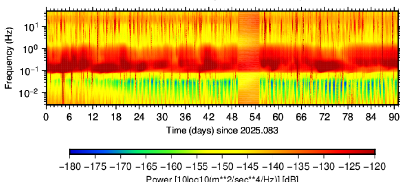
BK.PKD.HHE.00 (2025.083 - 2025.173)
