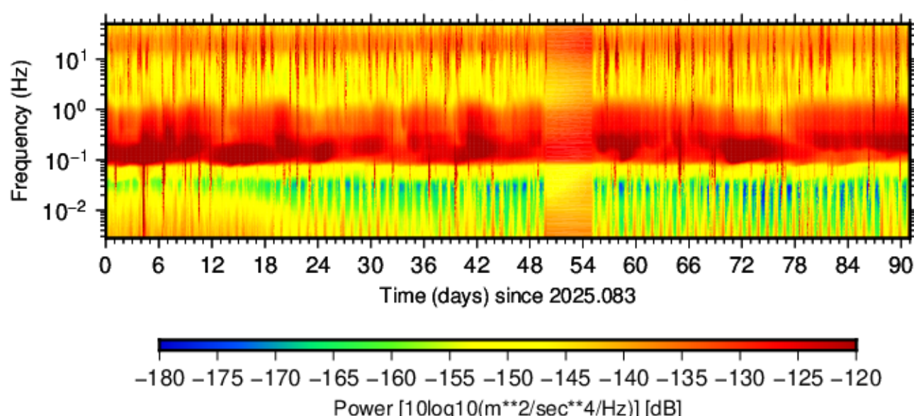
BK.PKD.HHN.00 (2025.083 - 2025.173)
