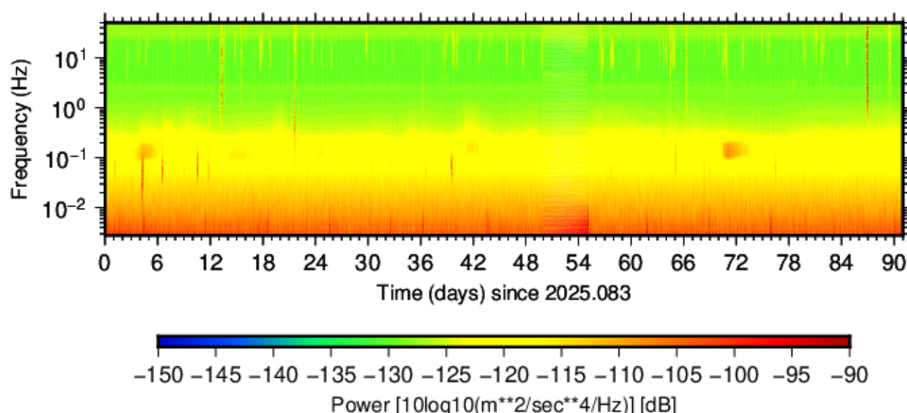
BK.PKD.HNZ.00 (2025.083 - 2025.173)
