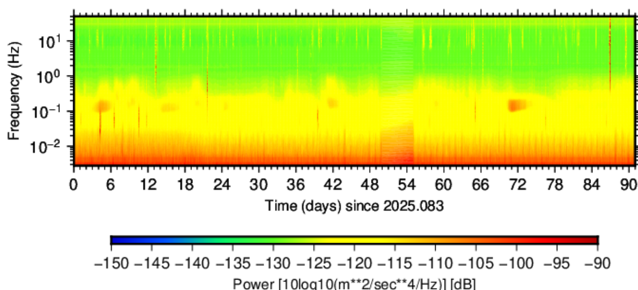
BK.PKD.HNE.00 (2025.083 - 2025.173)
