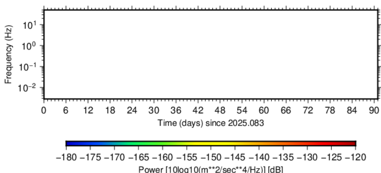
BK.PIT6.HHN.00 (2025.083 - 2025.173)
