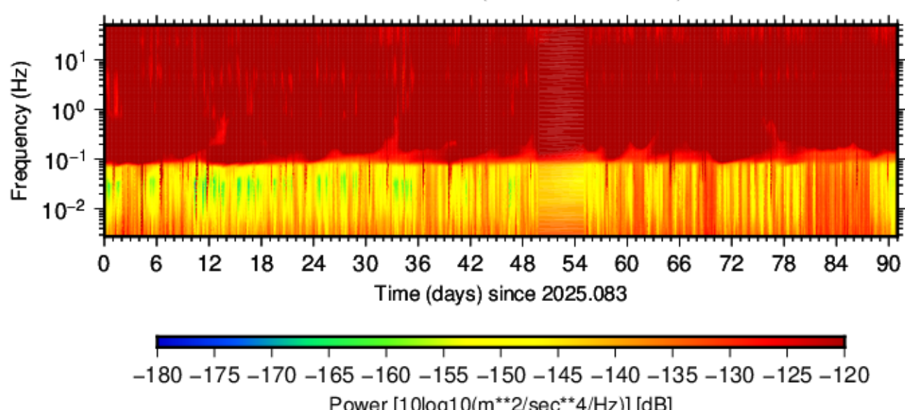
BK.PINL.HHE.00 (2025.083 - 2025.173)
