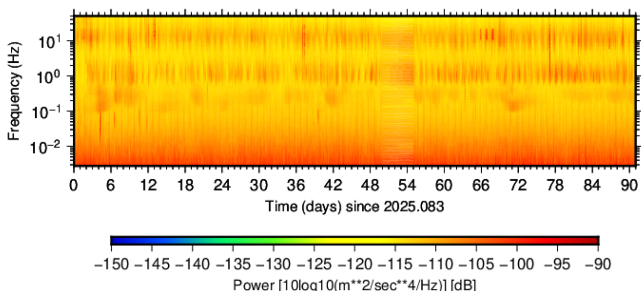
BK.PINL.HNZ.00 (2025.083 - 2025.173)
