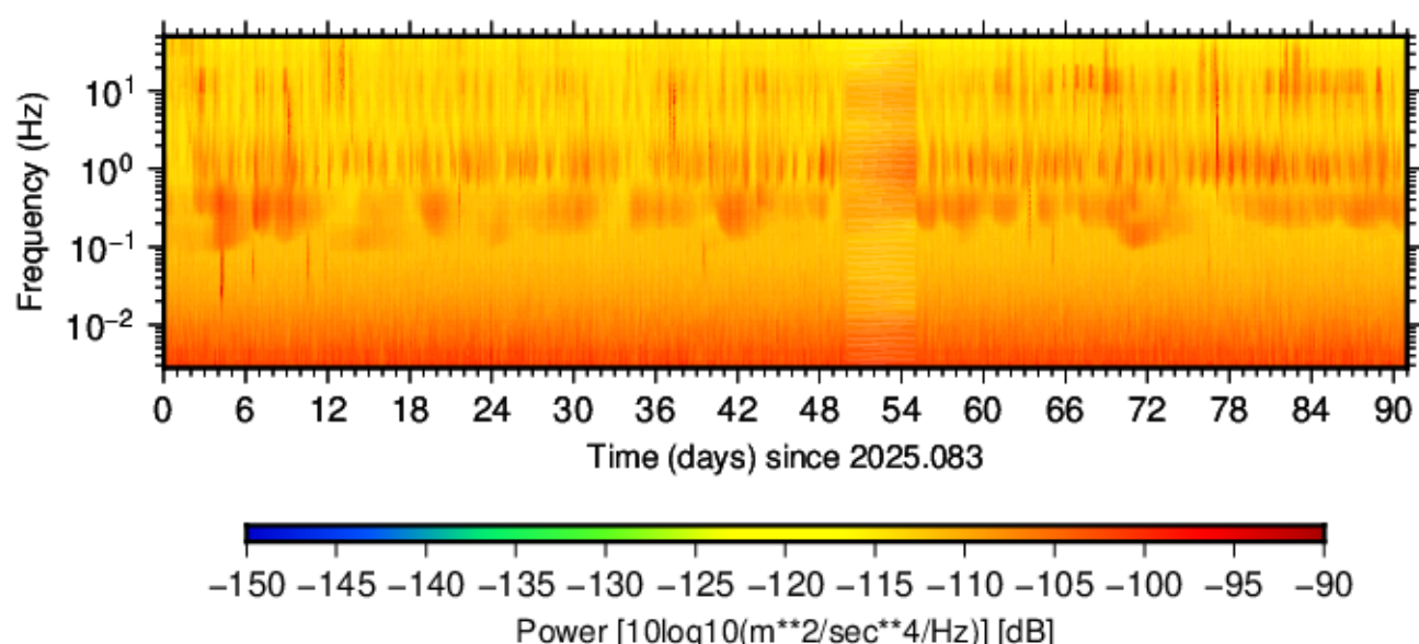
BK.PINL.HNE.00 (2025.083 - 2025.173)
