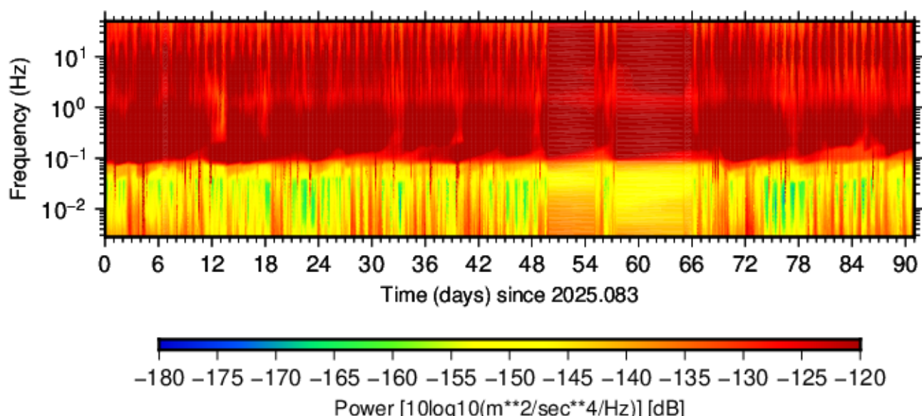
BK.PETL.HHN.00 (2025.083 - 2025.173)
