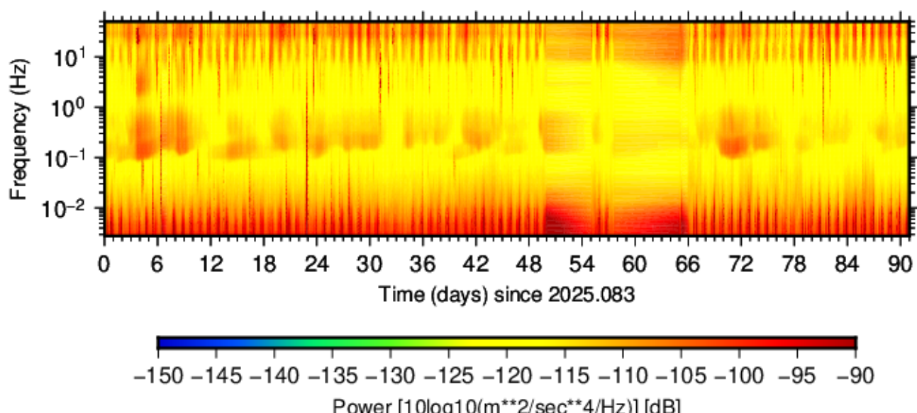
BK.PETL.HNN.00 (2025.083 - 2025.173)
