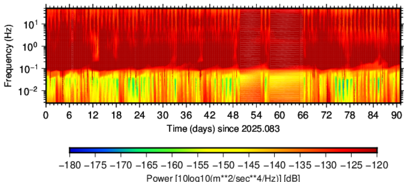
BK.PETL.HHE.00 (2025.083 - 2025.173)
