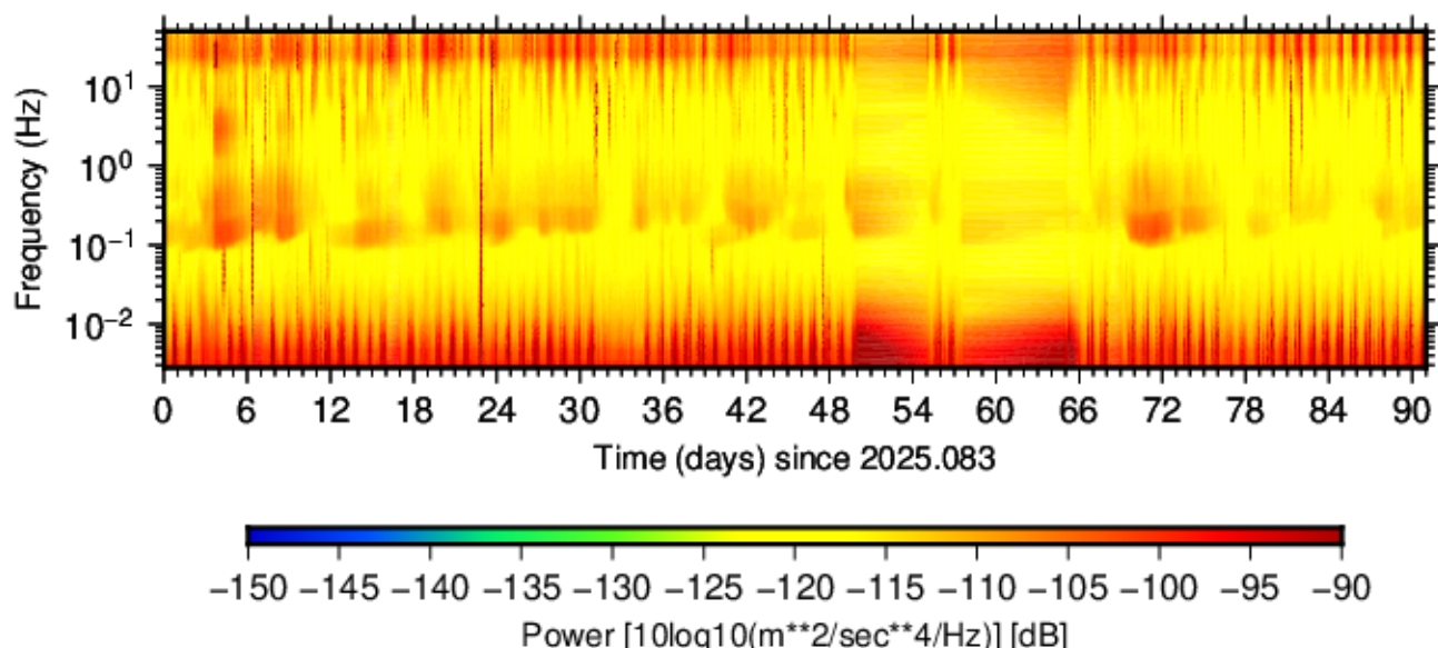
BK.PETL.HNE.00 (2025.083 - 2025.173)
