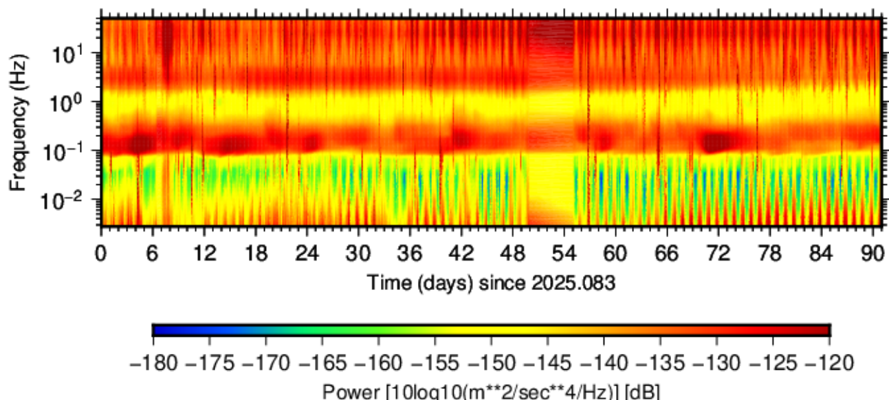
BK.PATT.HHE.00 (2025.083 - 2025.173)
