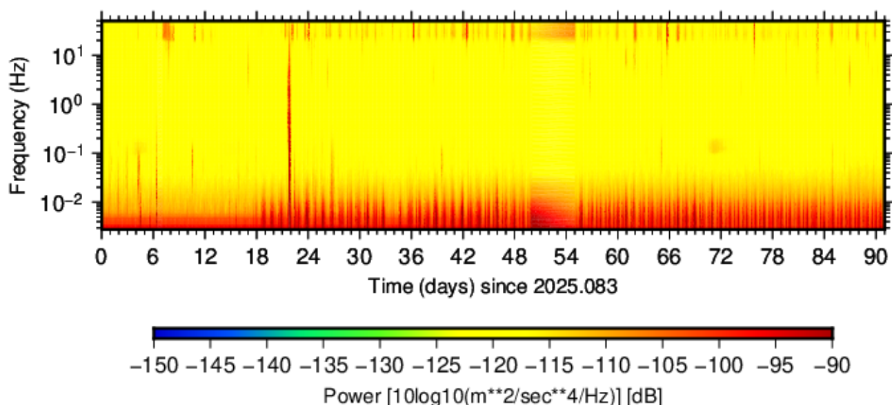
BK.PATT.HNN.00 (2025.083 - 2025.173)
