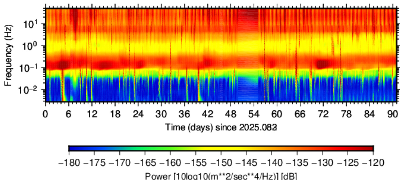
BK.PATT.HHZ.00 (2025.083 - 2025.173)
