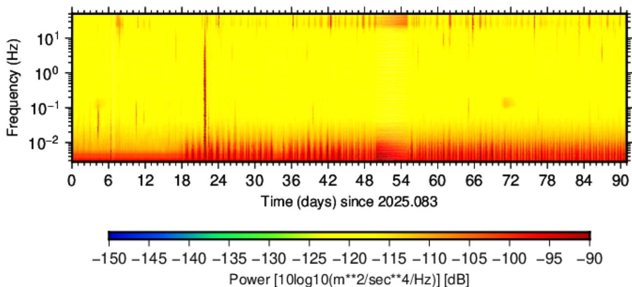
BK.PATT.HNE.00 (2025.083 - 2025.173)
