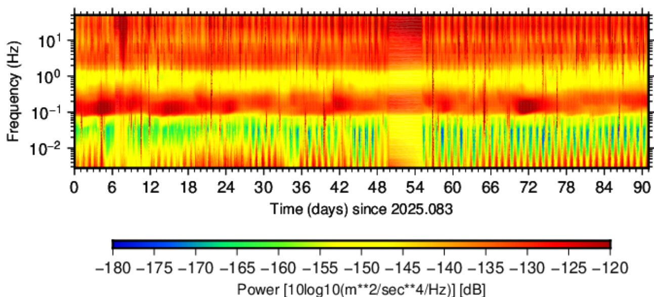
BK.PATT.HHN.00 (2025.083 - 2025.173)
