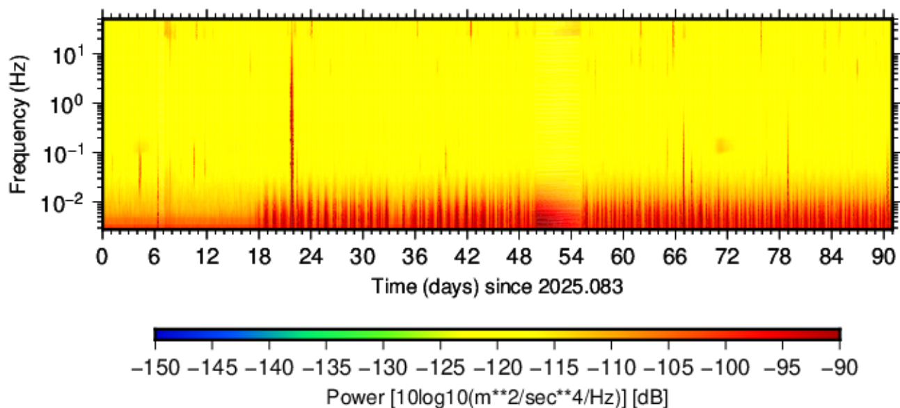
BK.PATT.HNZ.00 (2025.083 - 2025.173)
