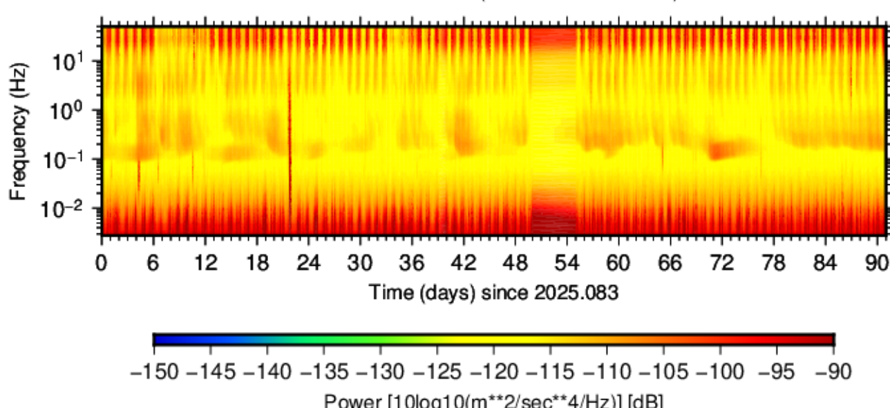
BK.PABC.HNN.00 (2025.083 - 2025.173)
