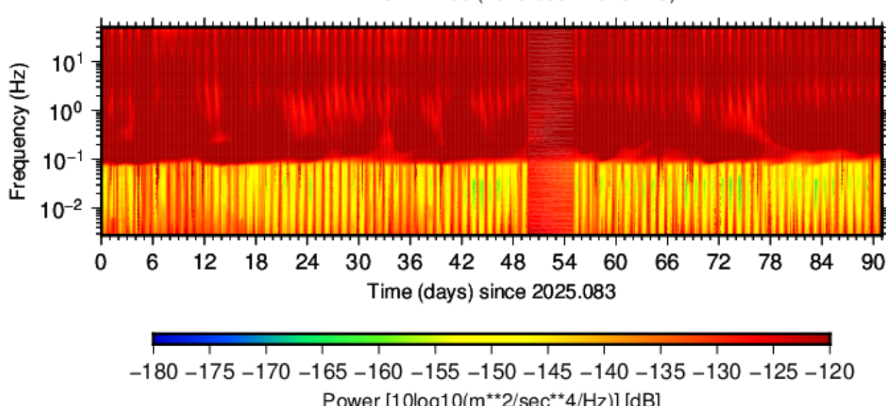
BK.PABC.HHE.00 (2025.083 - 2025.173)
