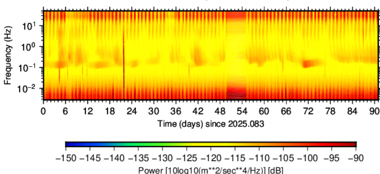
BK.PABC.HNE.00 (2025.083 - 2025.173)
