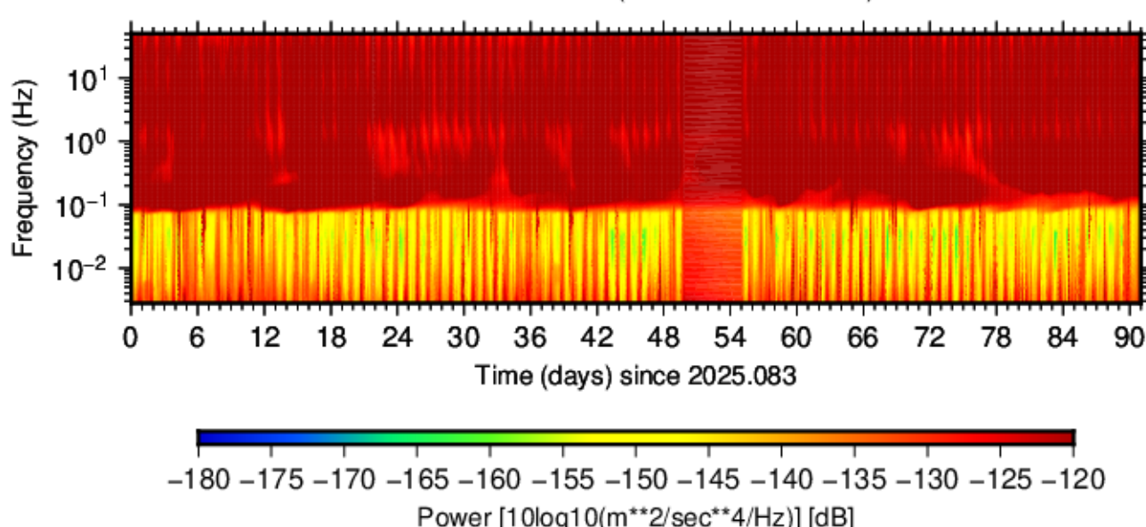
BK.PABC.HHN.00 (2025.083 - 2025.173)
