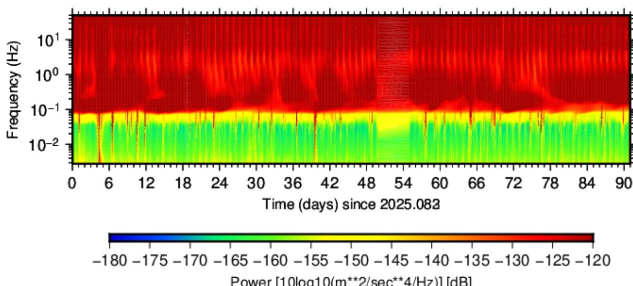
BK.PABC.HHZ.00 (2025.083 - 2025.173)
