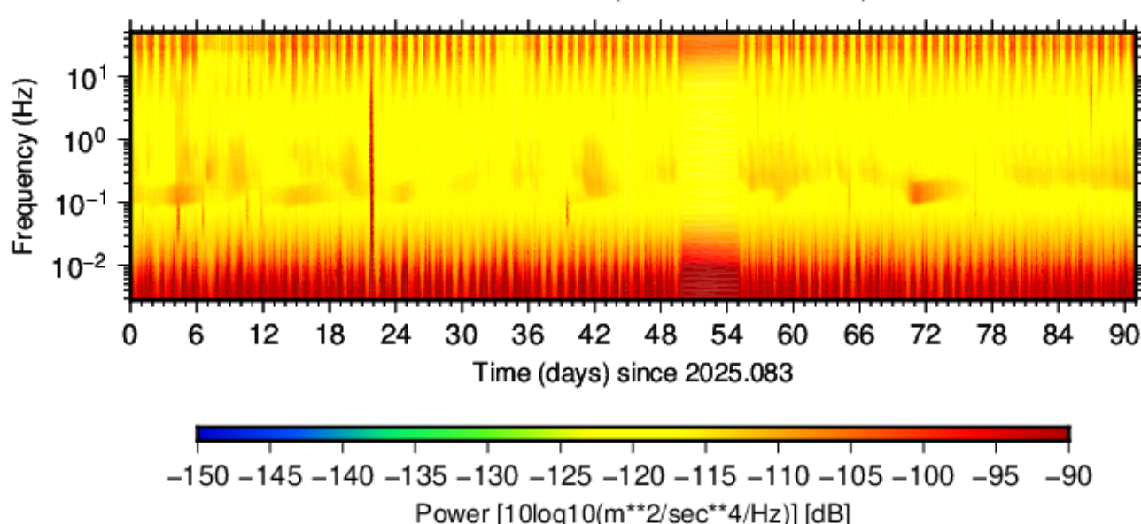
BK.PABC.HNZ.00 (2025.083 - 2025.173)
