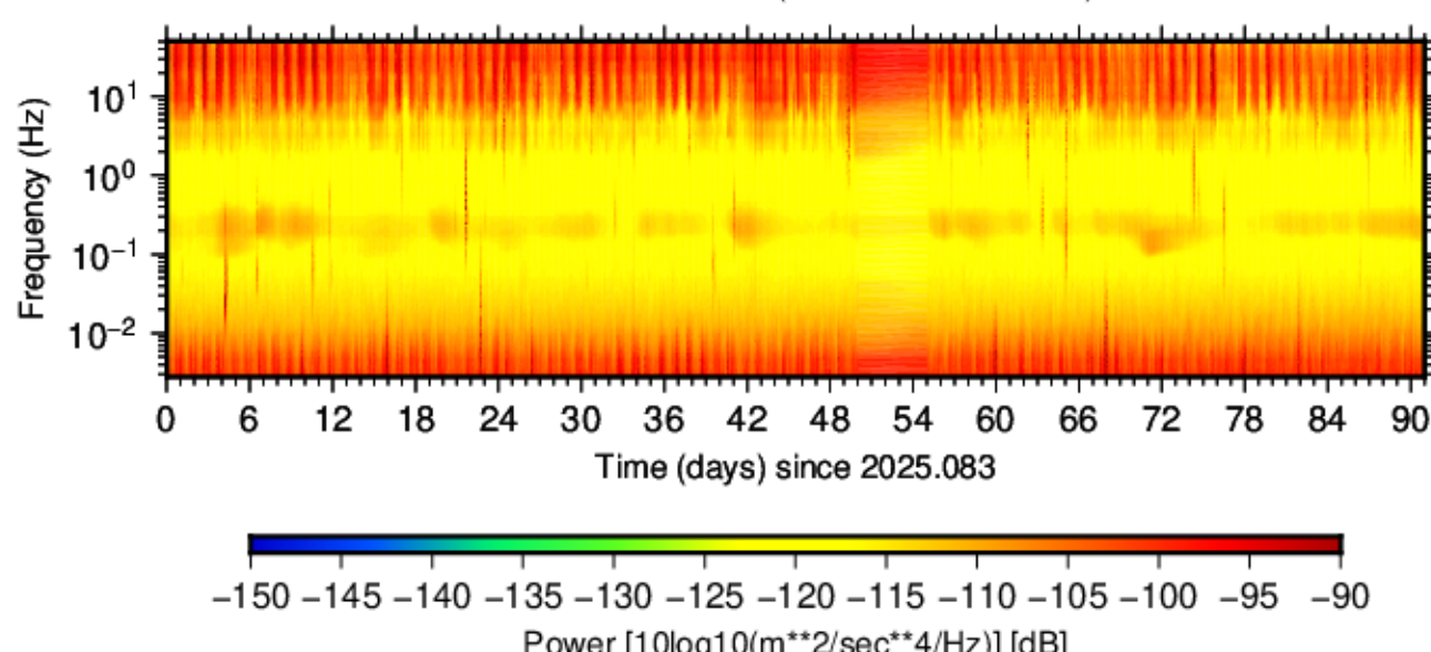
BK.OVRO.HNE.00 (2025.083 - 2025.173)
