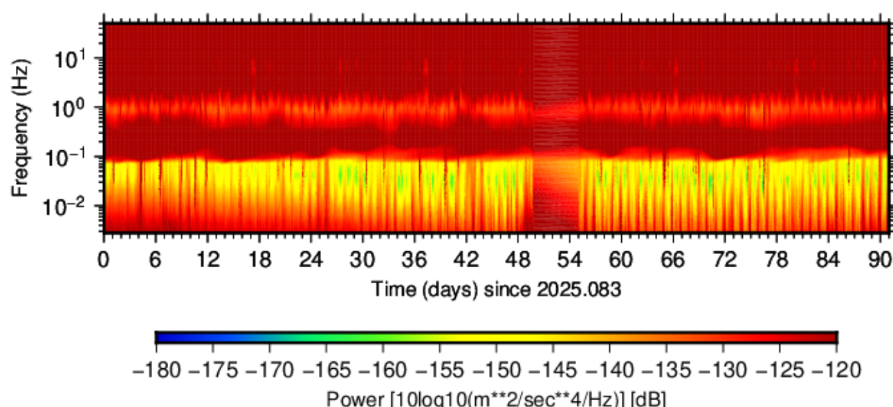
BK.OVRO.HHN.00 (2025.083 - 2025.173)
