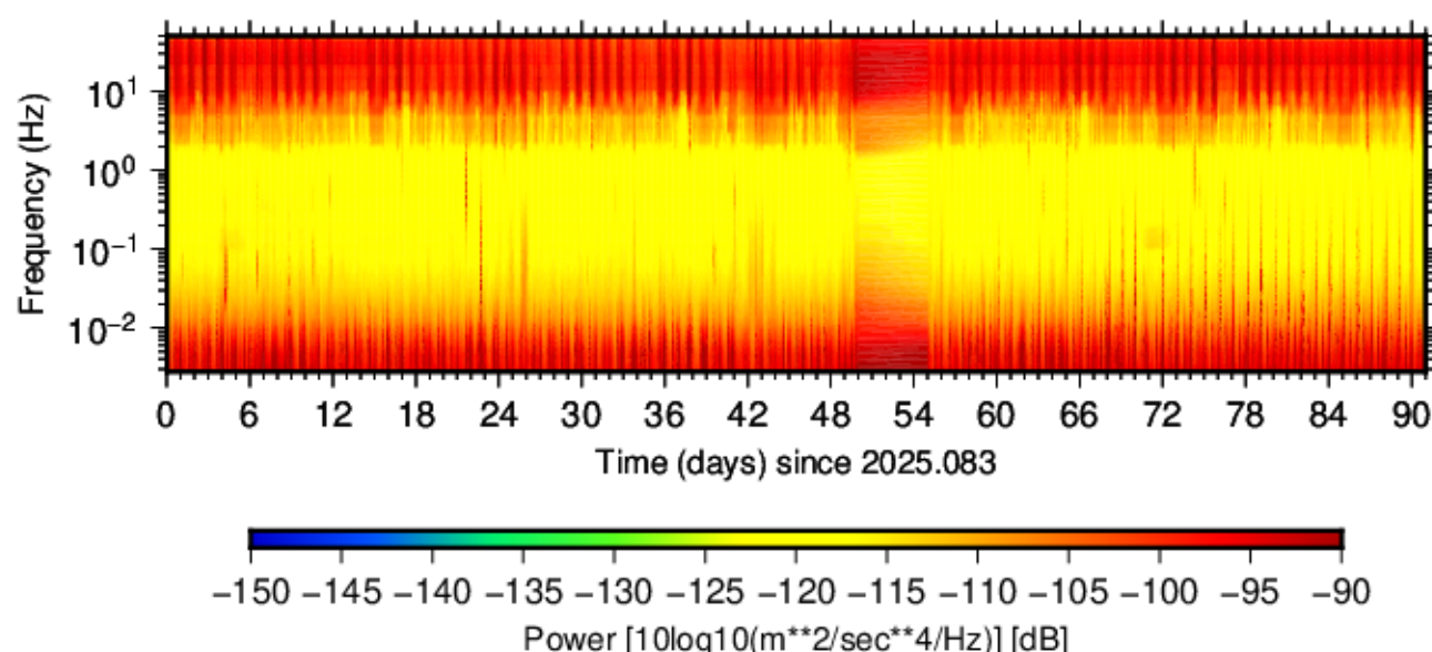
BK.OVRO.HNZ.00 (2025.083 - 2025.173)
