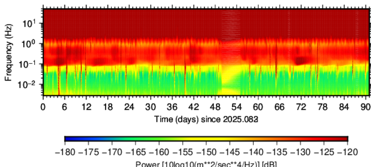
BK.OVRO.HHZ.00 (2025.083 - 2025.173)
