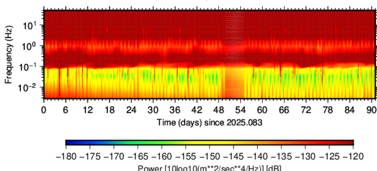
BK.OVRO.HHE.00 (2025.083 - 2025.173)
