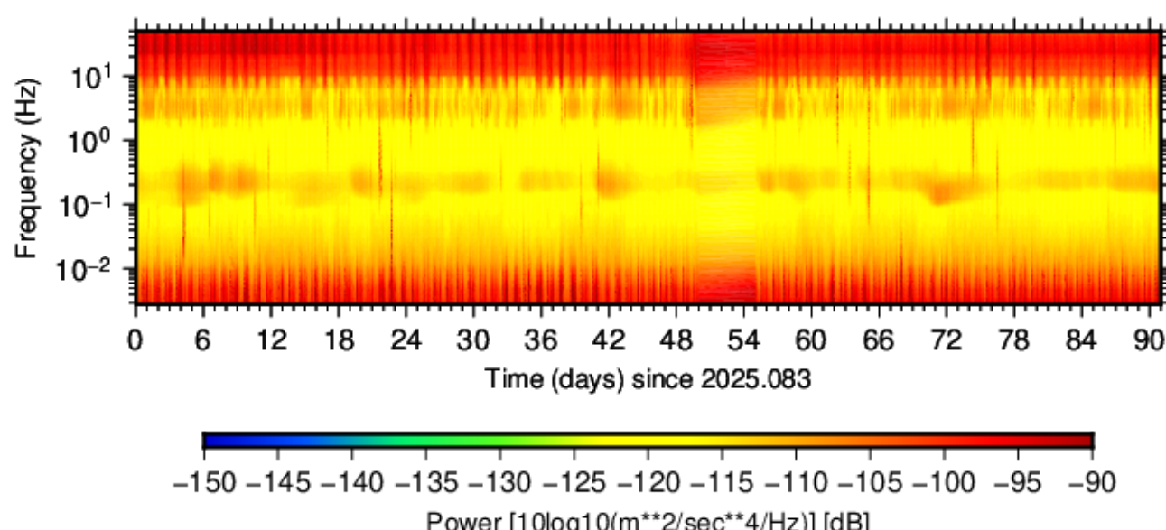
BK.OVRO.HNN.00 (2025.083 - 2025.173)
