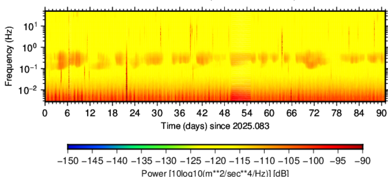
BK.ORRS.HNE.00 (2025.083 - 2025.173)
