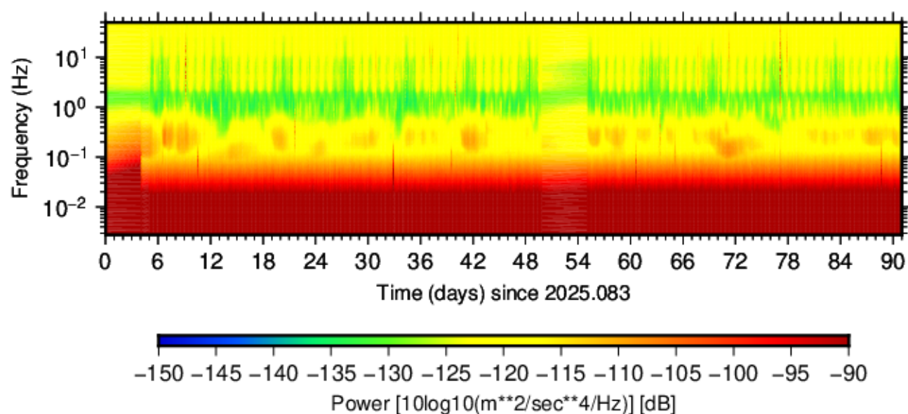
BK.OHLN.EP2.40 (2025.083 - 2025.173)
