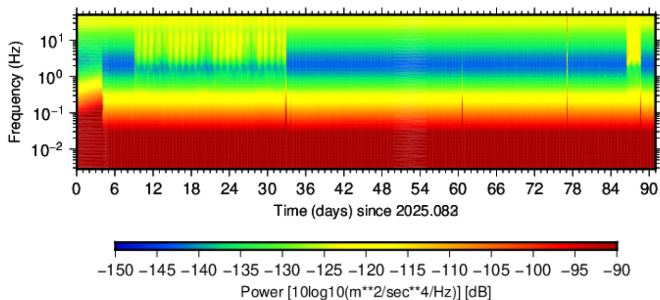
BK.OHLN.EP1.40 (2025.083 - 2025.173)
