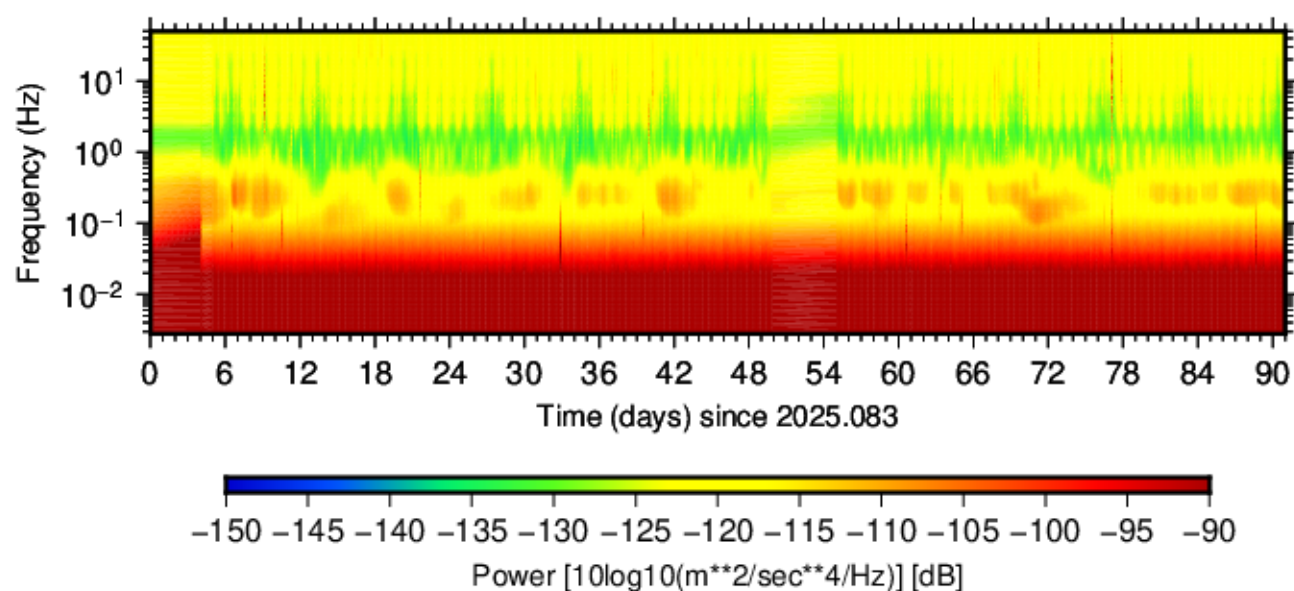
BK.OHLN.EP3.40 (2025.083 - 2025.173)
