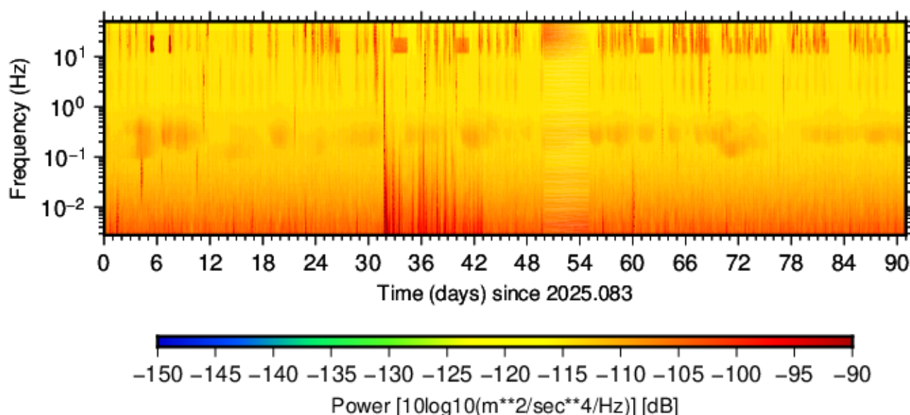
BK.OAKV.HNN.00 (2025.083 - 2025.173)
