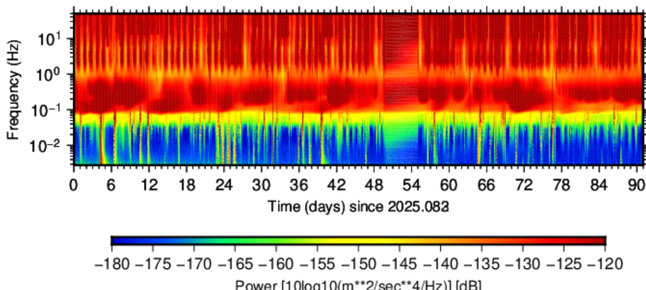
BK.OAKV.HHZ.00 (2025.083 - 2025.173)
