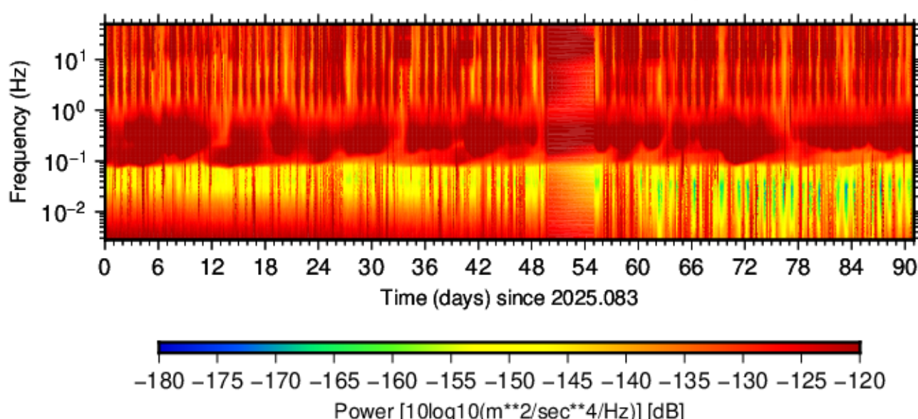
BK.OAKV.HHN.00 (2025.083 - 2025.173)
