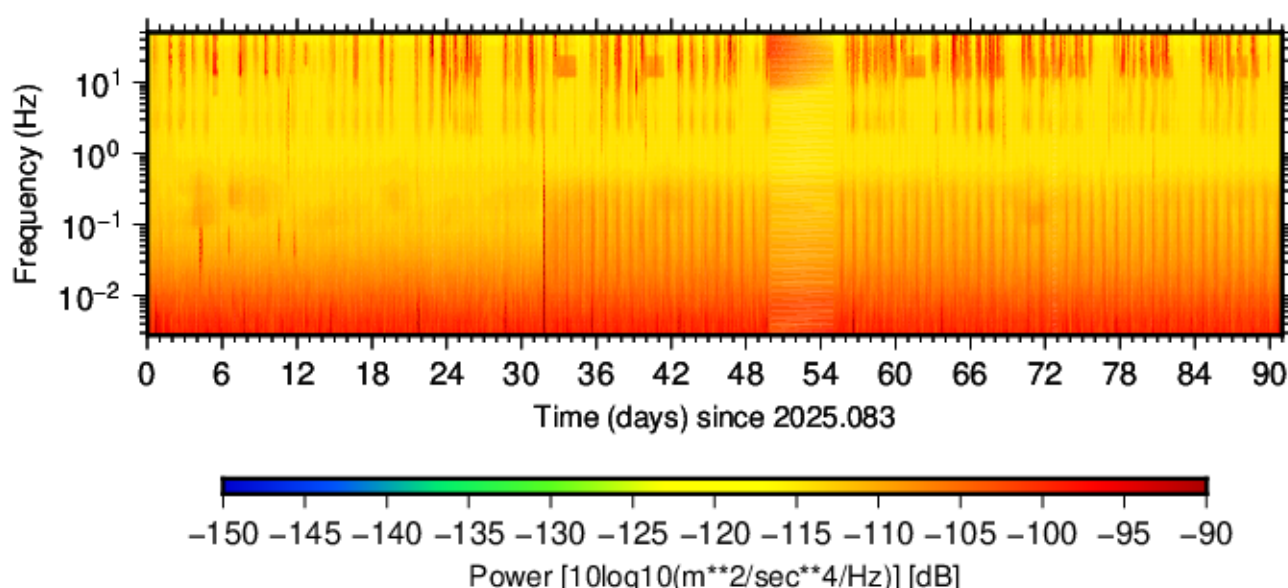
BK.OAKV.HNZ.00 (2025.083 - 2025.173)
