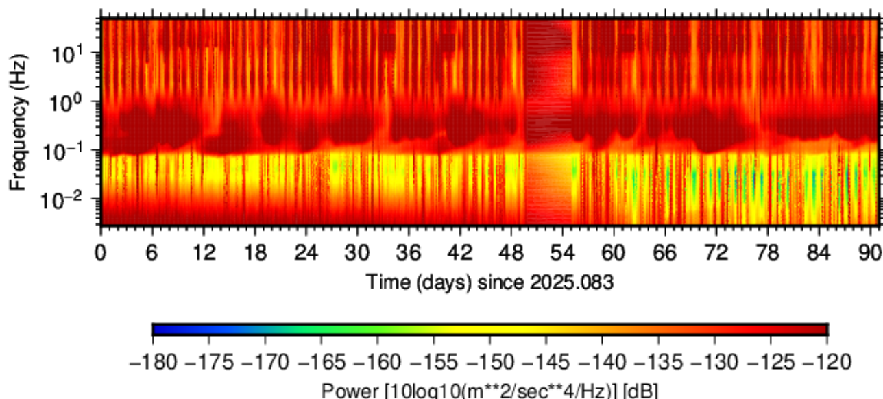
BK.OAKV.HHE.00 (2025.083 - 2025.173)
