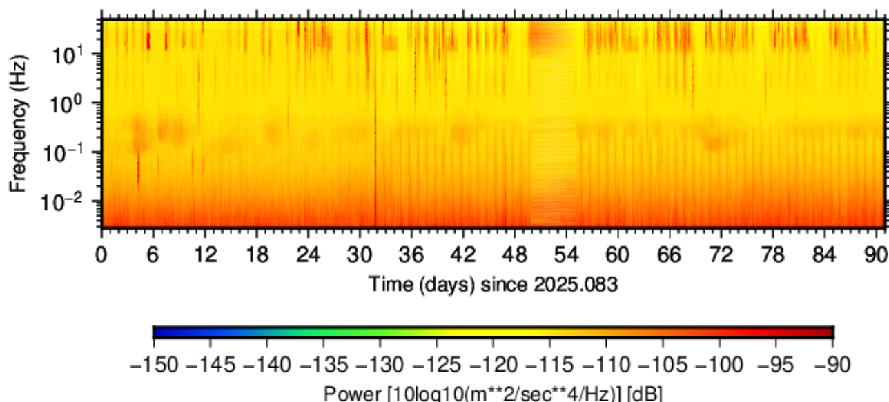
BK.OAKV.HNE.00 (2025.083 - 2025.173)
