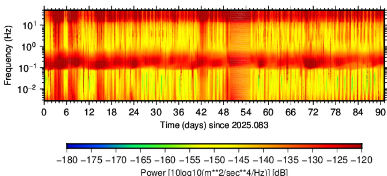
BK.MZTA.HHN.00 (2025.083 - 2025.173)
