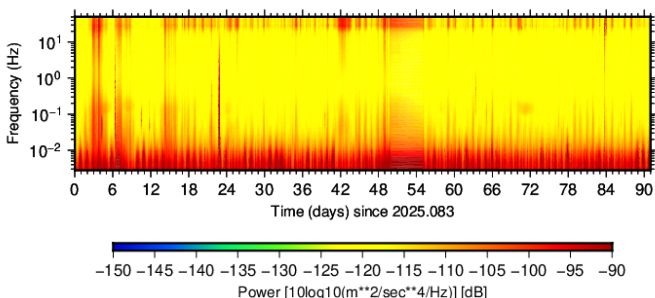
BK.MZTA.HNE.00 (2025.083 - 2025.173)
