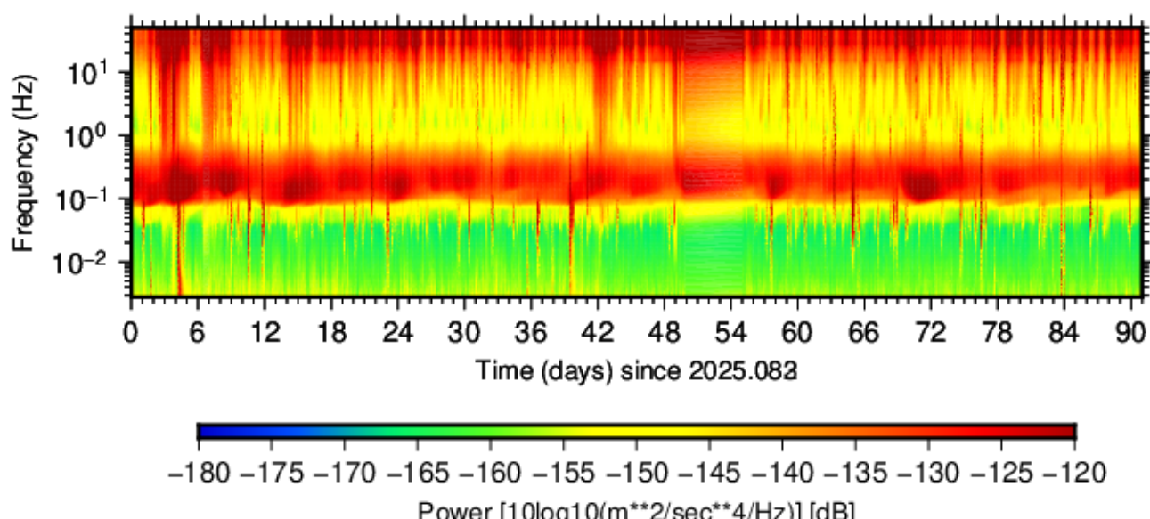
BK.MZTA.HHZ.00 (2025.083 - 2025.173)
