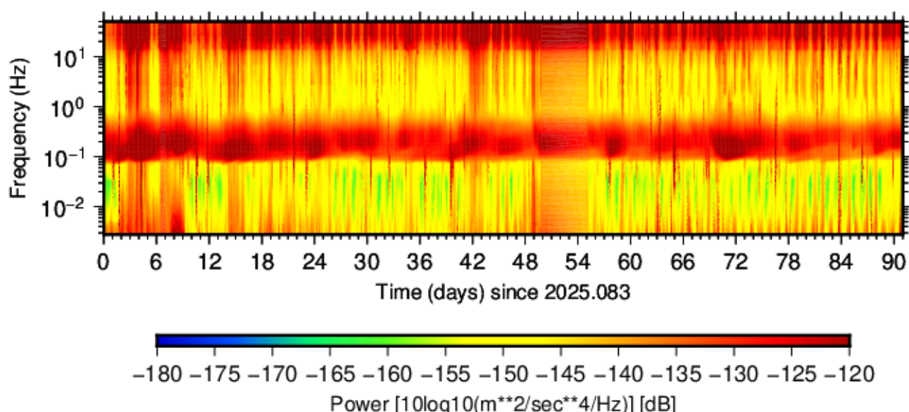
BK.MZTA.HHE.00 (2025.083 - 2025.173)
