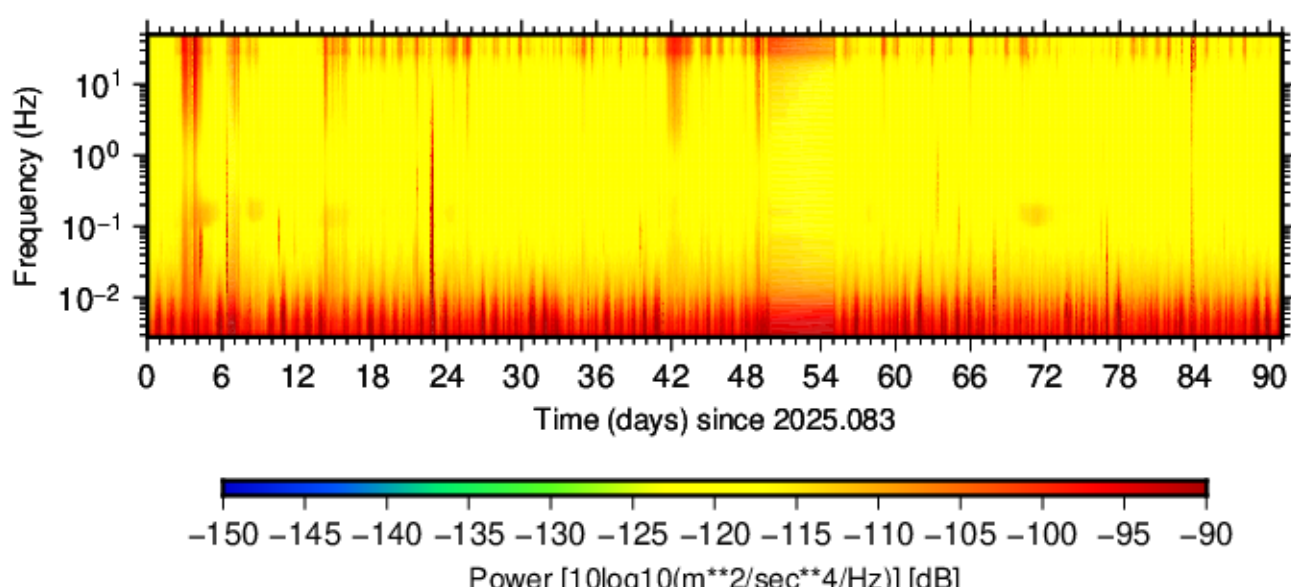
BK.MZTA.HNN.00 (2025.083 - 2025.173)
