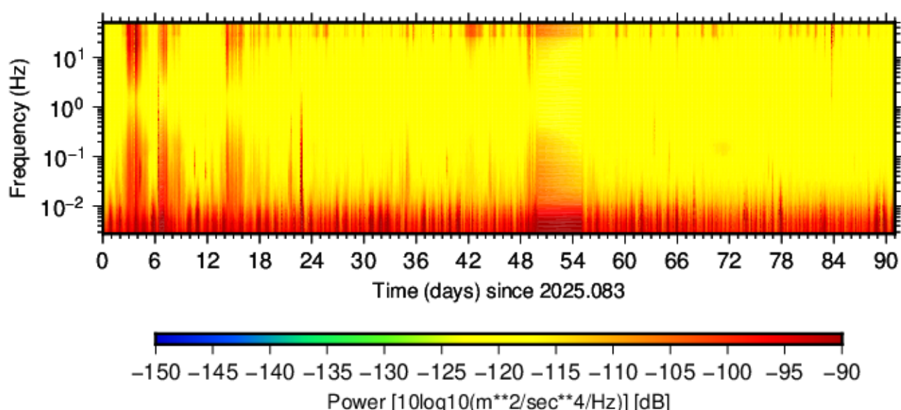
BK.MZTA.HNZ.00 (2025.083 - 2025.173)
