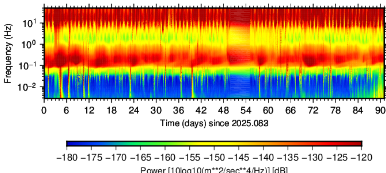
BK.MOGU.HHZ.00 (2025.083 - 2025.173)
