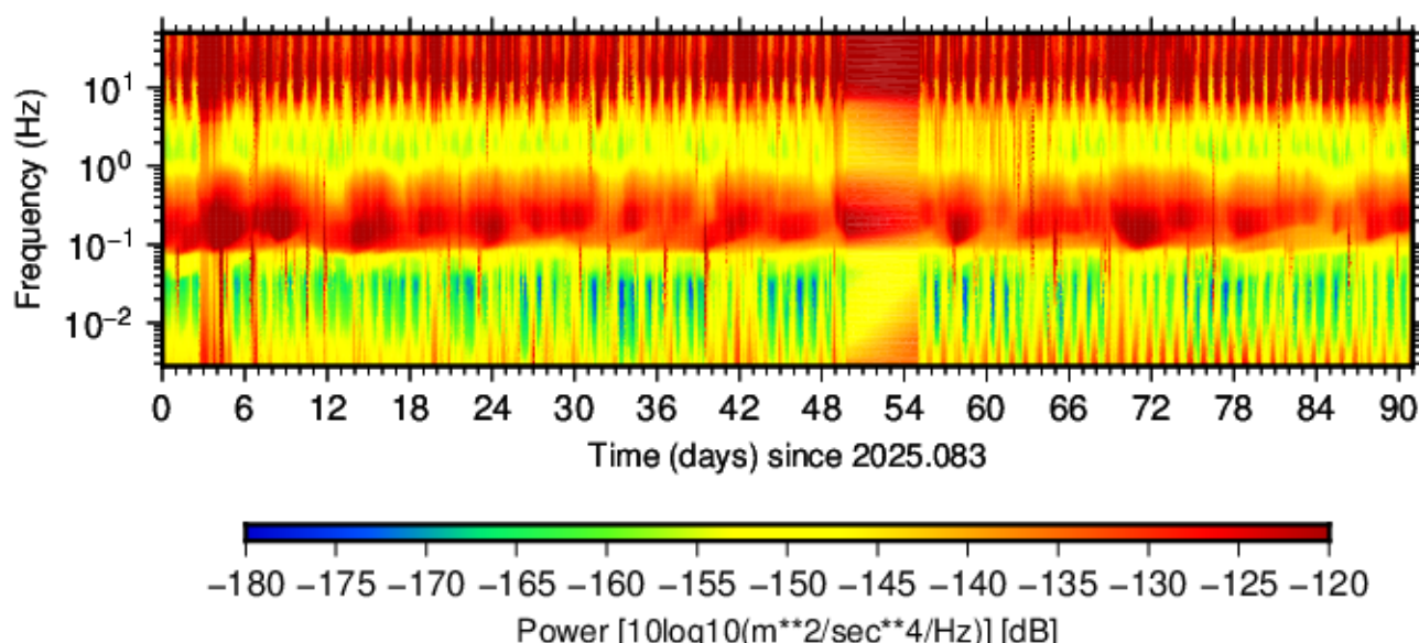
BK.MOGU.HHN.00 (2025.083 - 2025.173)
