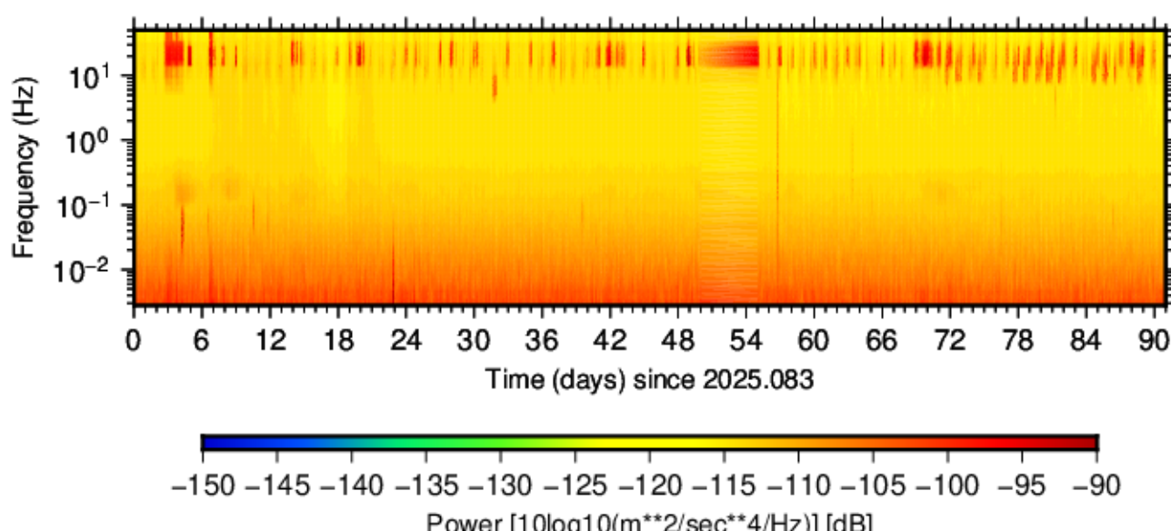
BK.MOGU.HNE.00 (2025.083 - 2025.173)
