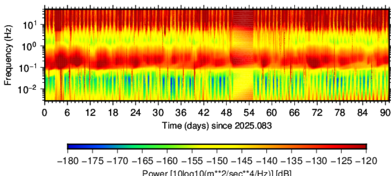
BK.MOGU.HHE.00 (2025.083 - 2025.173)
