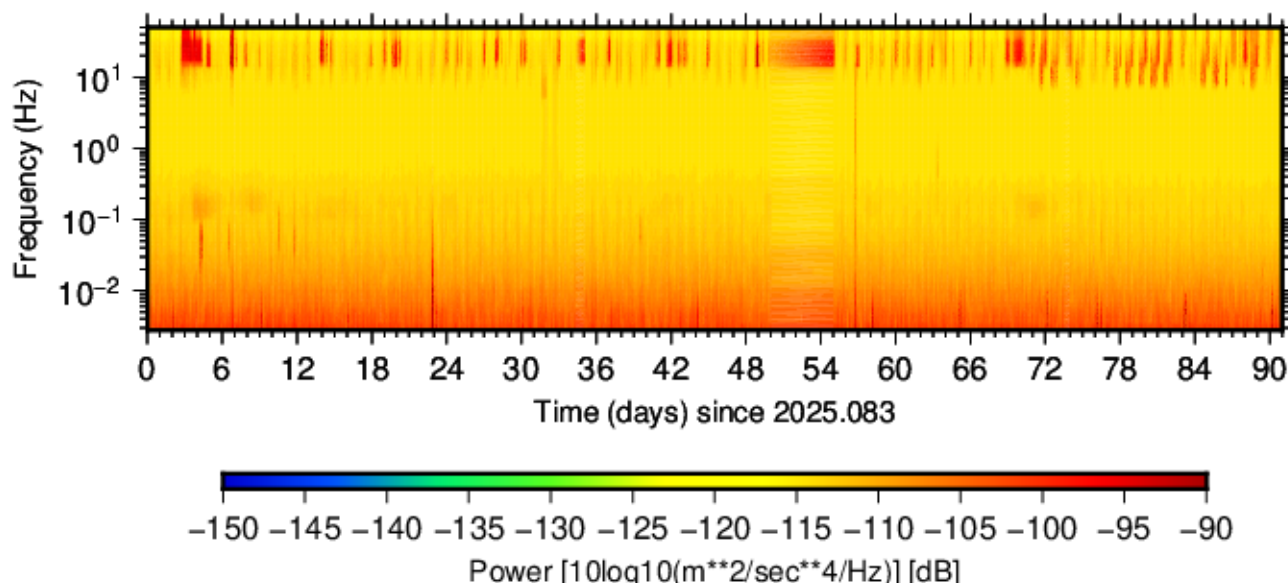
BK.MOGU.HNZ.00 (2025.083 - 2025.173)
