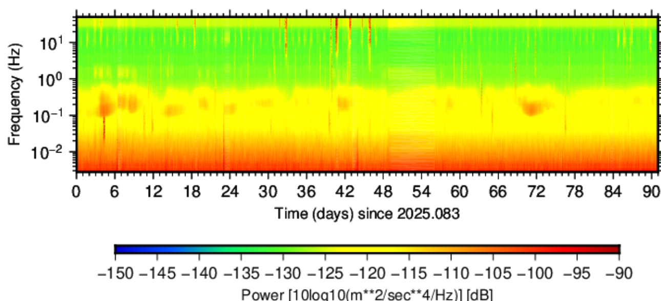
BK.MNRC.HNE.00 (2025.083 - 2025.173)
