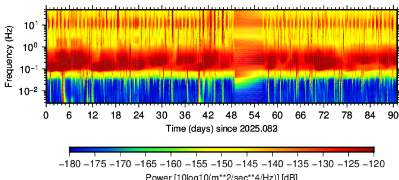
BK.MNRC.HHZ.00 (2025.083 - 2025.173)
