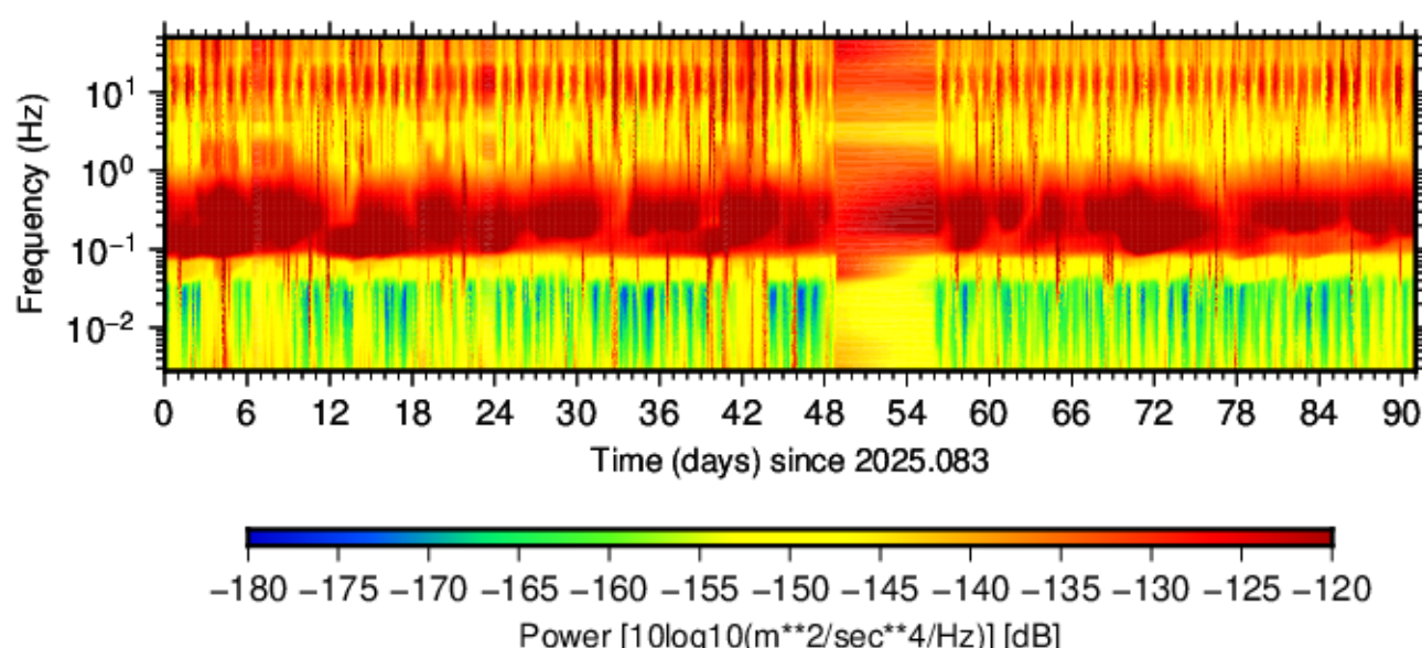
BK.MNRC.HHN.00 (2025.083 - 2025.173)
