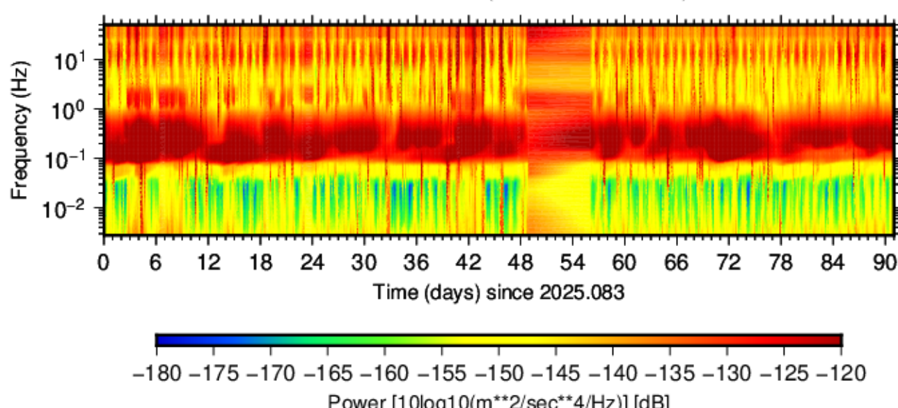
BK.MNRC.HHE.00 (2025.083 - 2025.173)
