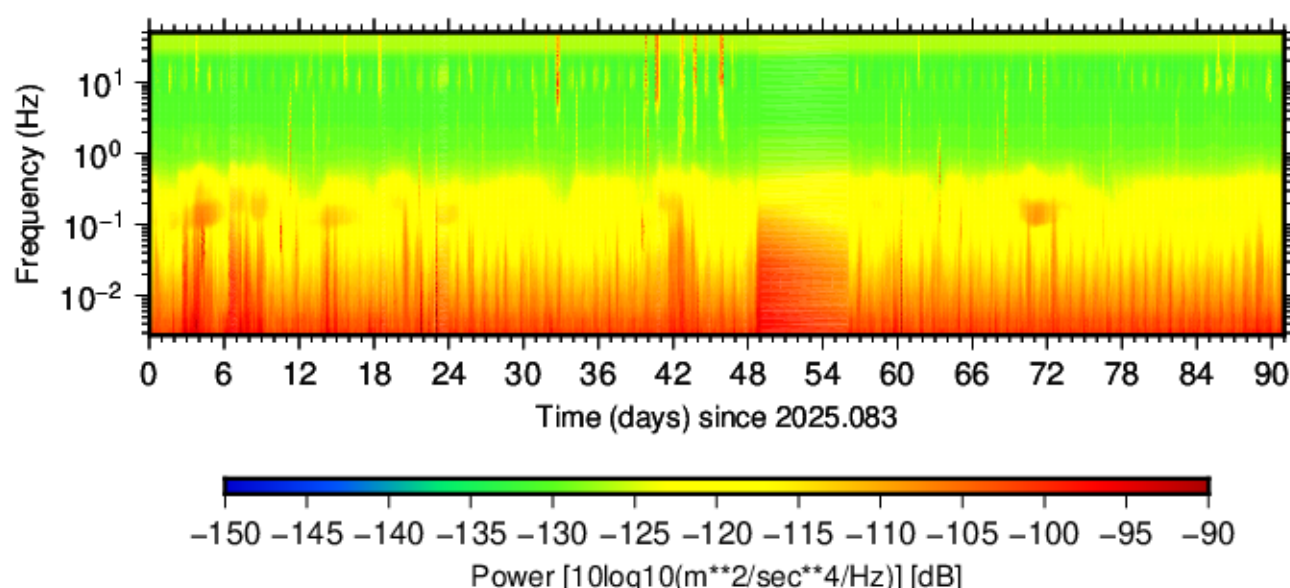
BK.MNRC.HNZ.00 (2025.083 - 2025.173)
