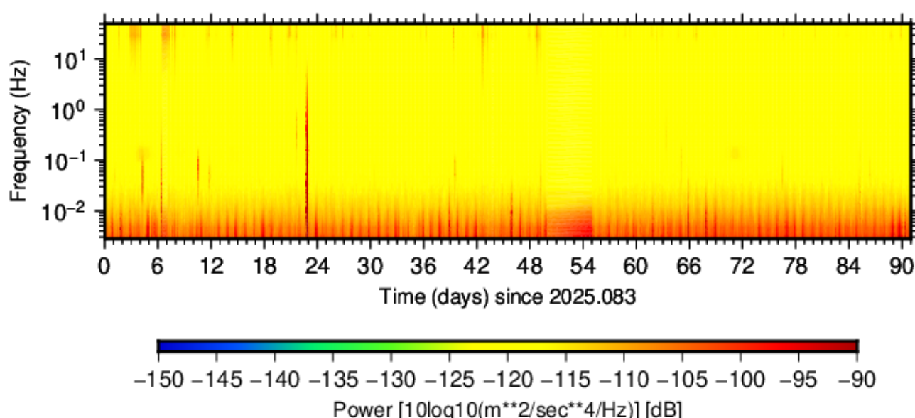
BK.MNLT.HNE.00 (2025.083 - 2025.173)
