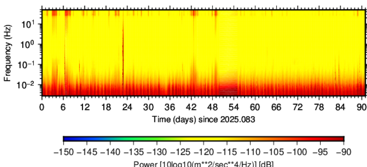
BK.MNLT.HNN.00 (2025.083 - 2025.173)
