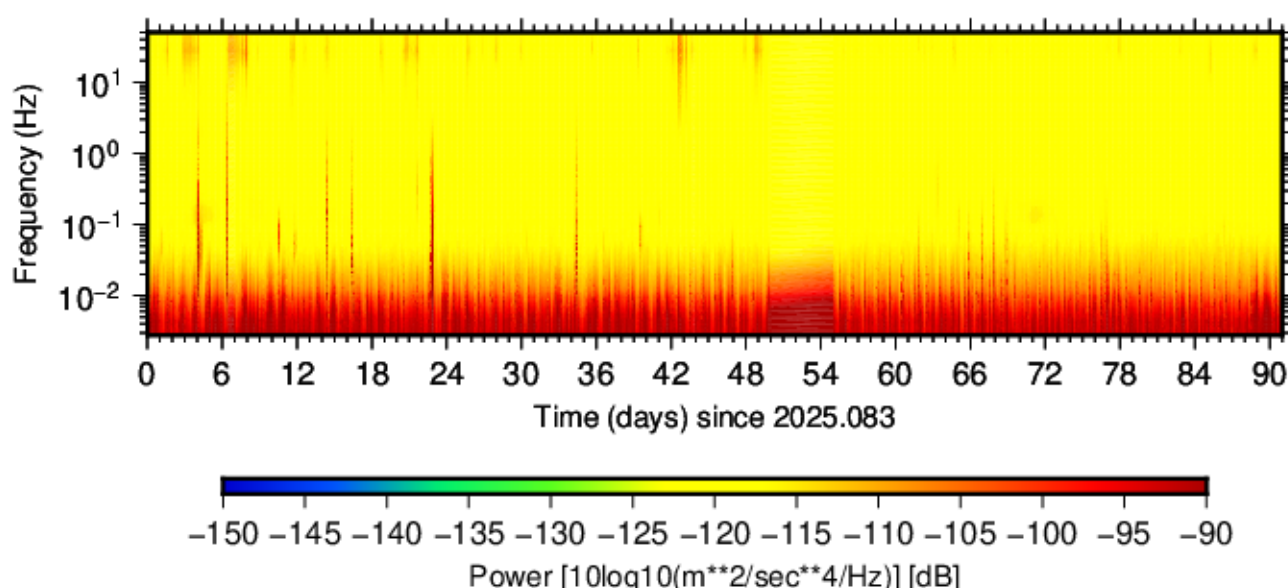
BK.MNLT.HNZ.00 (2025.083 - 2025.173)
