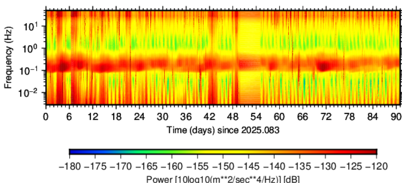
BK.MNLT.HHN.00 (2025.083 - 2025.173)
