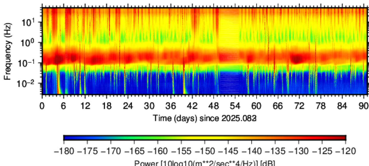
BK.MNLT.HHZ.00 (2025.083 - 2025.173)
