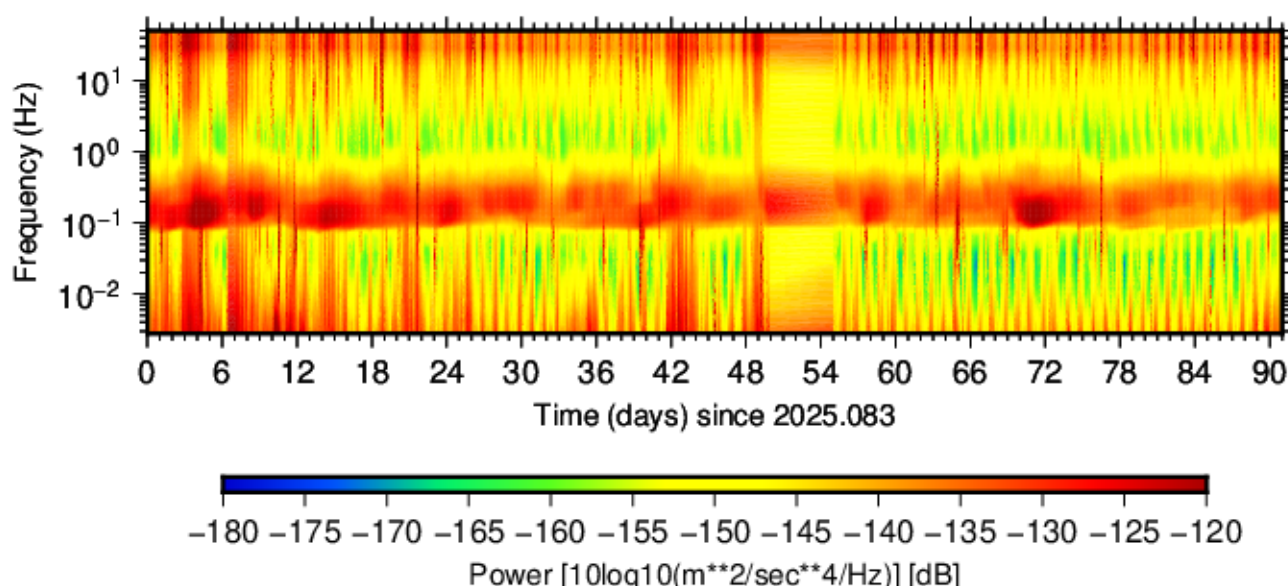
BK.MNLT.HHE.00 (2025.083 - 2025.173)
