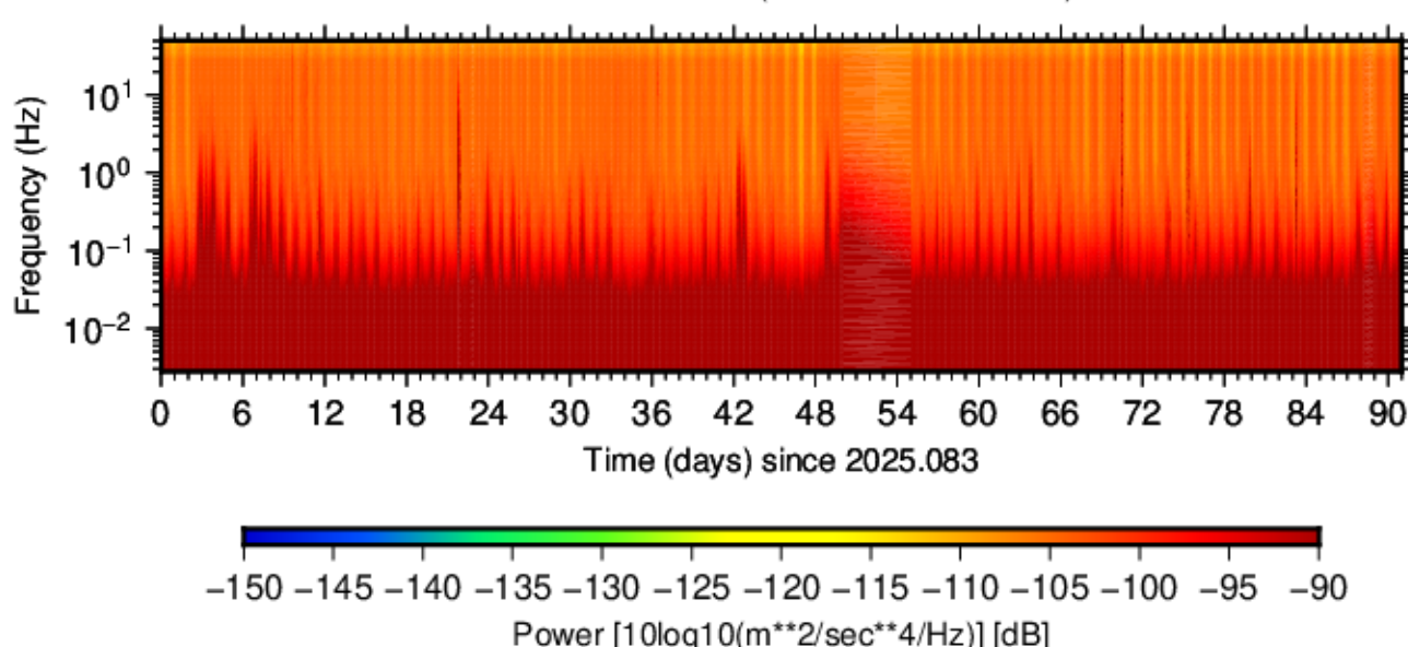
BK.MLKN.HNE.00 (2025.083 - 2025.173)
