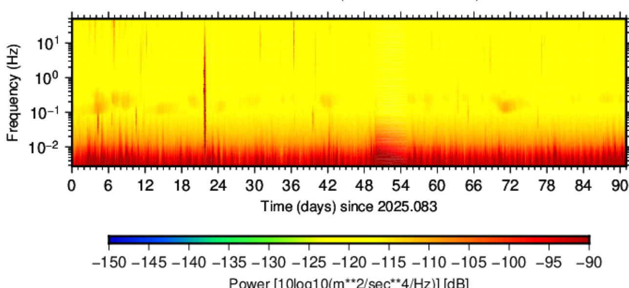
BK.MLKN.HNN.00 (2025.083 - 2025.173)
