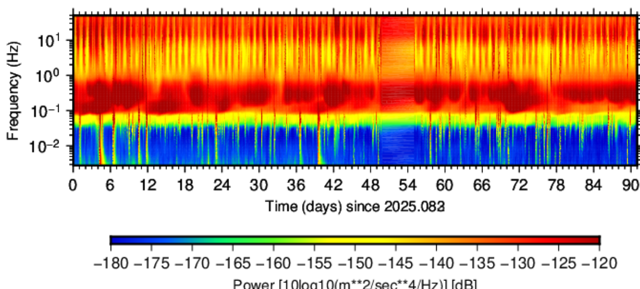
BK.MLKN.HHZ.00 (2025.083 - 2025.173)
