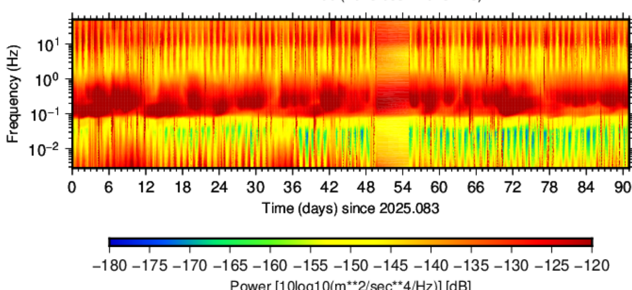
BK.MLKN.HHE.00 (2025.083 - 2025.173)
