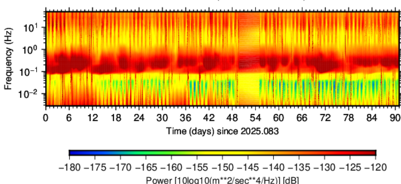
BK.MLKN.HHN.00 (2025.083 - 2025.173)
