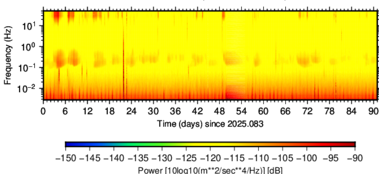
BK.MILL.HNE.00 (2025.083 - 2025.173)
