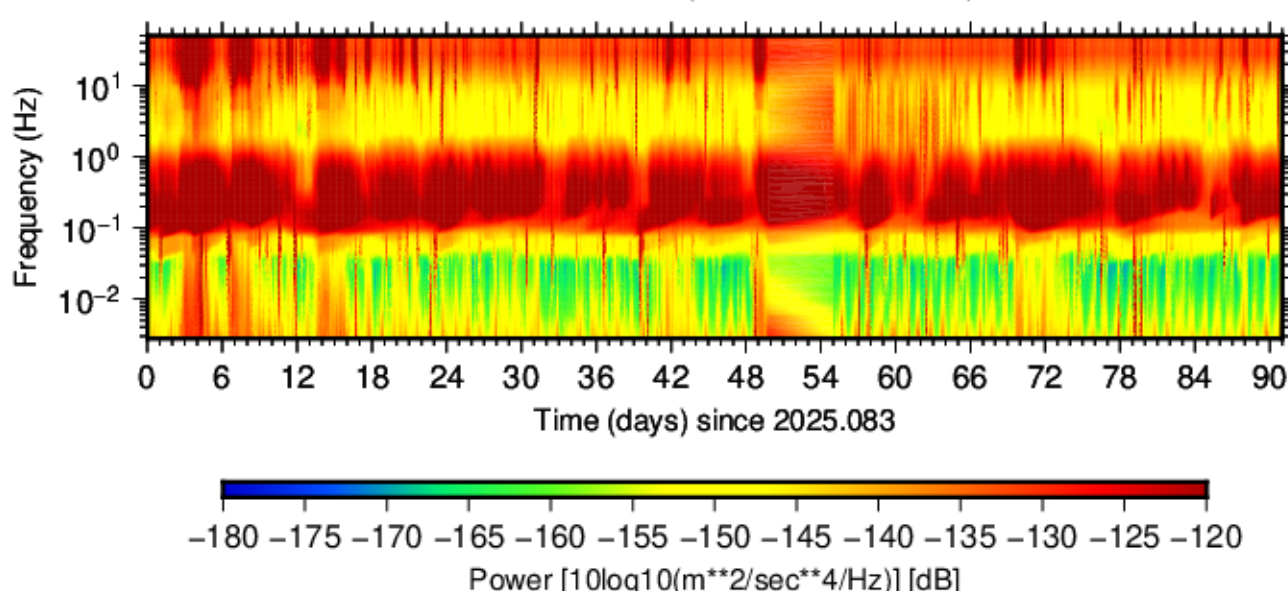
BK.MILL.HHE.00 (2025.083 - 2025.173)
