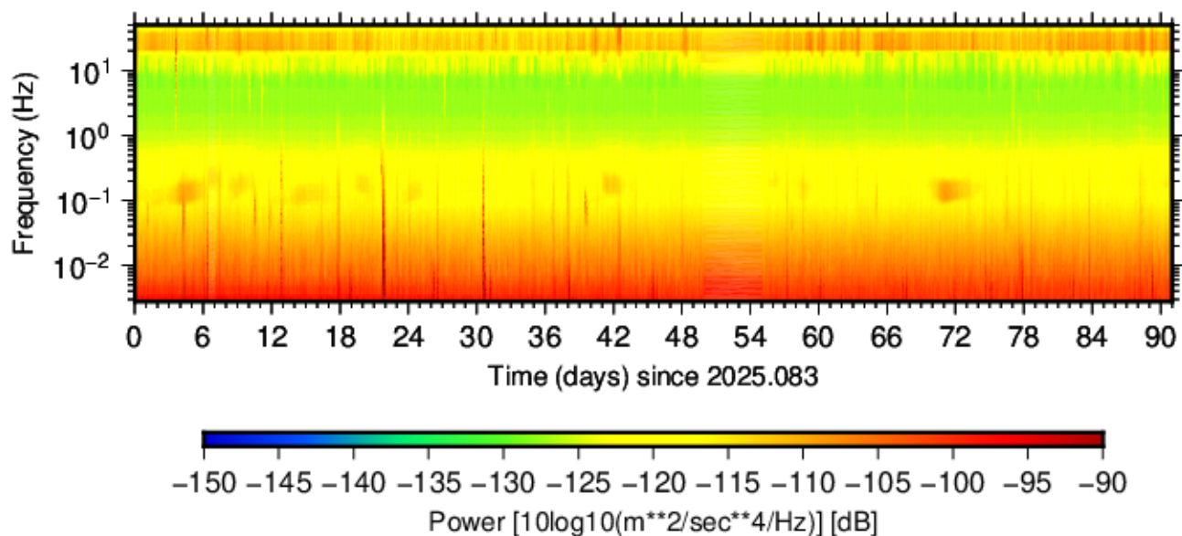
BK.MHC.HNZ.00 (2025.083 - 2025.173)
