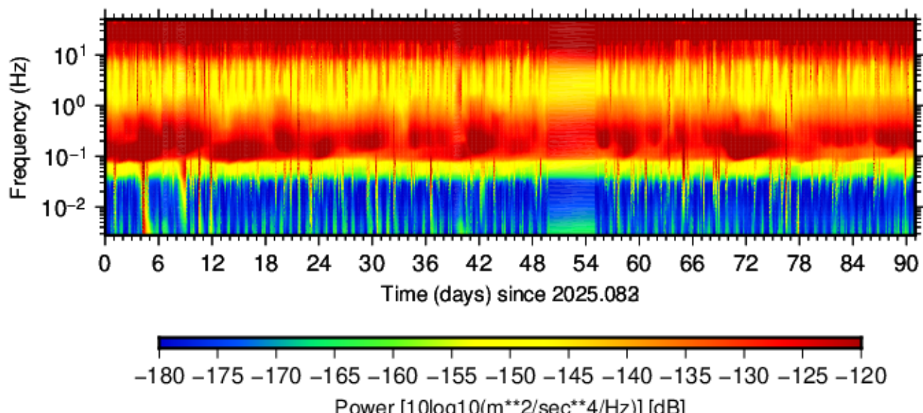
BK.MHC.HHZ.00 (2025.083 - 2025.173)
