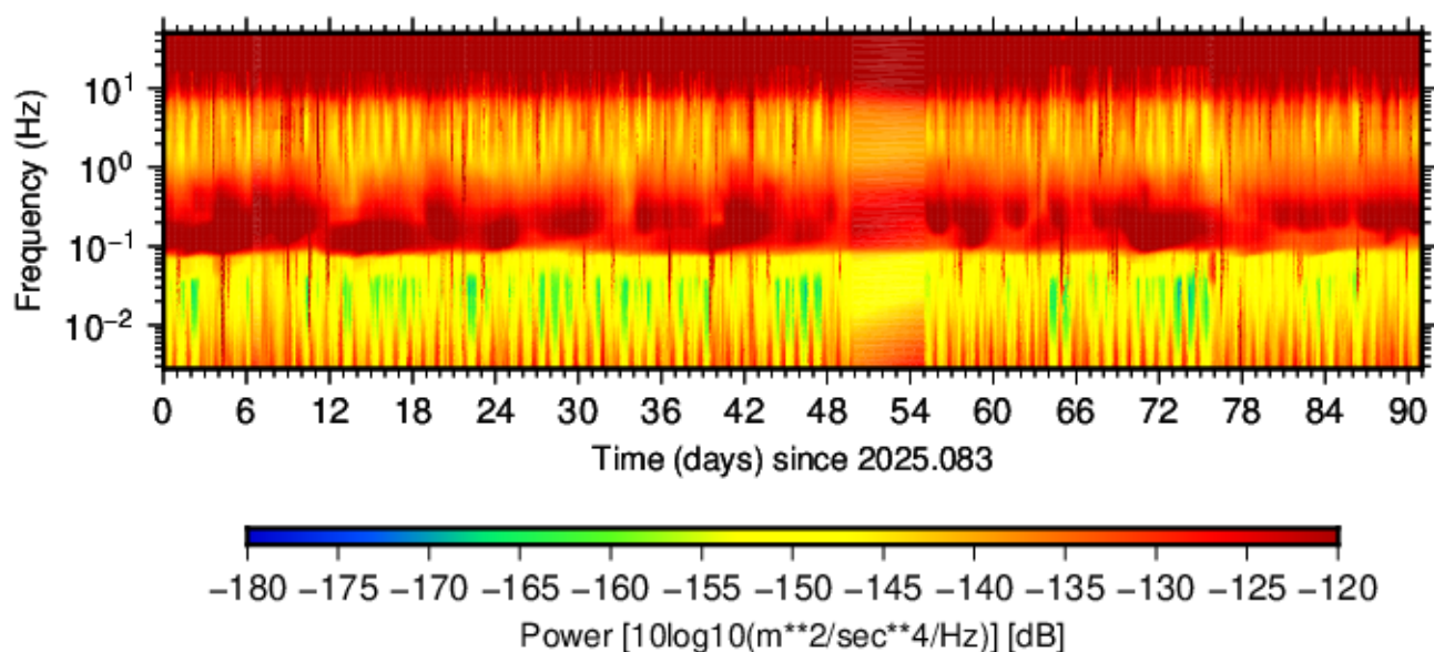
BK.MHC.HHN.00 (2025.083 - 2025.173)
