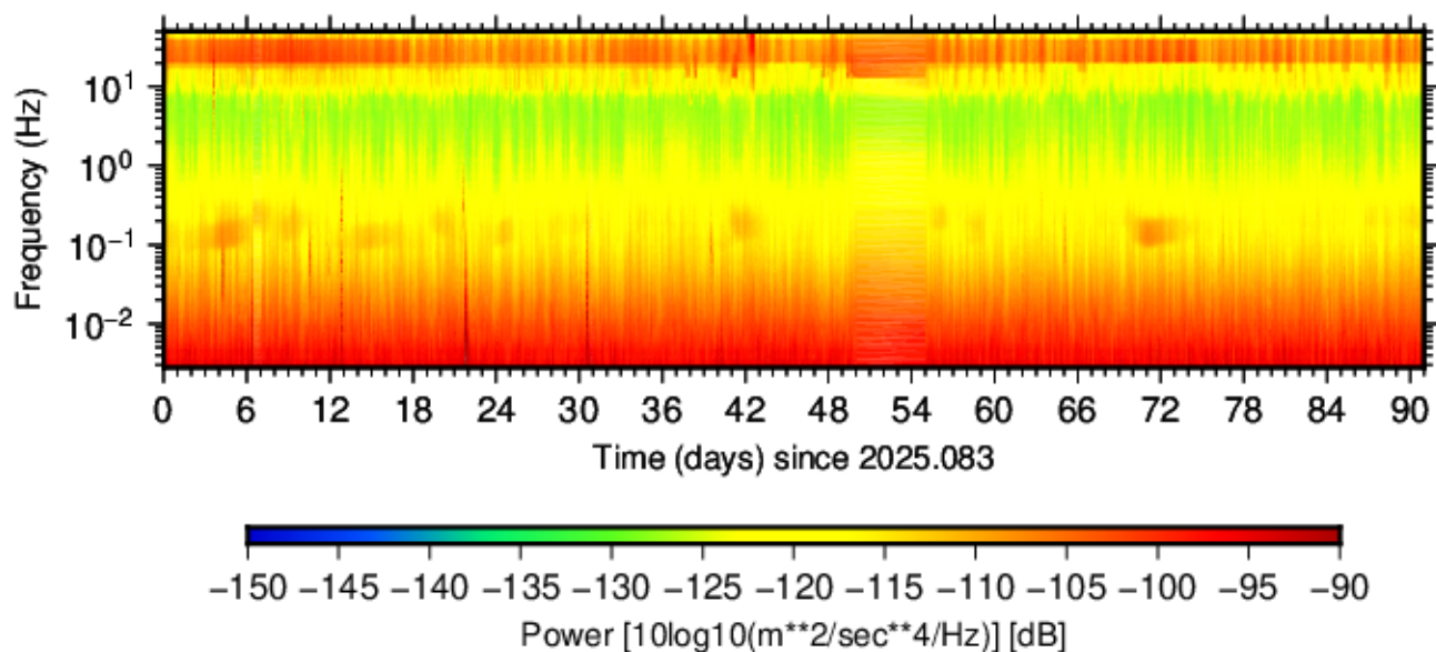
BK.MHC.HNE.00 (2025.083 - 2025.173)
