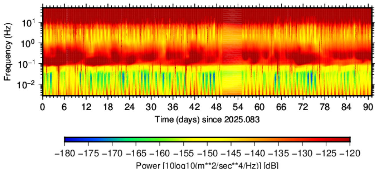
BK.MHC.HHE.00 (2025.083 - 2025.173)
